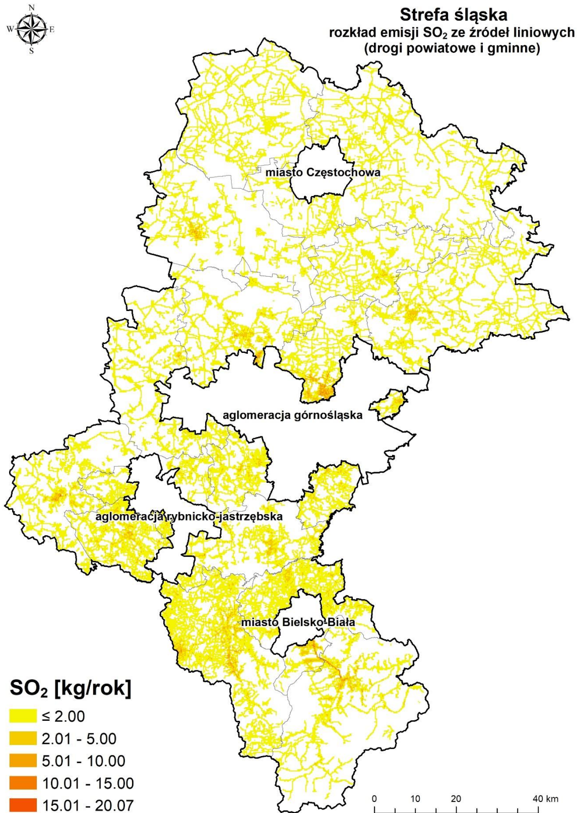
Rysunek 41. Lokalizacja i wielkość emisji dwutlenku siarki z dróg powiatowych i gminnych w strefie śląskiej w roku bazowym 2017
