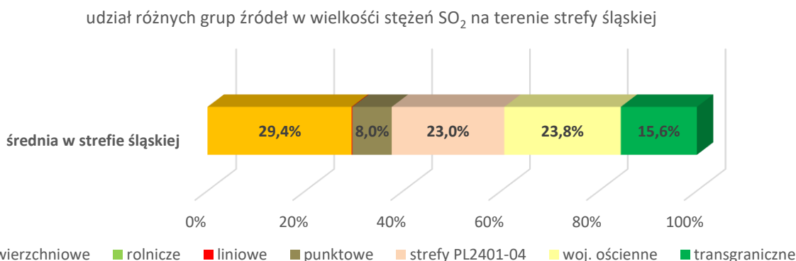
Rysunek 18. Udziały poszczególnych rodzajów źródeł emisji w wielkości stężeń średniorocznych dwutlenku siarki na terenie strefy śląskiej
