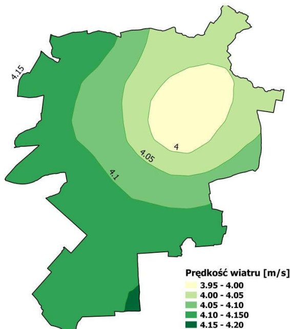
Rysunek 3 Rozkład średniej rocznej prędkości wiatru wyznaczonej przez model WRF/CALMET w strefie aglomeracja lubelska w 2015 r.
