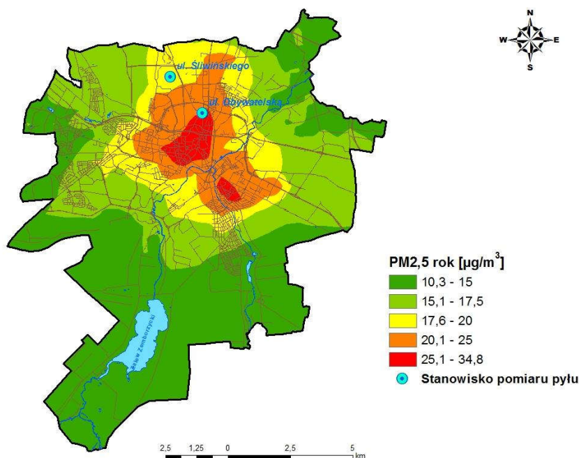
Rysunek 39 Stężenia pyłu zawieszzonego PM2,5 o okresie uśredniania wyników rok w strefie aglomeracja lubelska pochodzące z łącznej emisji wszystkich typów w 2015 r.
