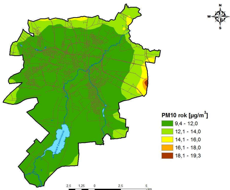
Rysunek 35 Stężenia pyłu zawieszzonego PM10 o okresie uśredniania wyników rok w strefie aglomeracja lubelska pochodzące z tła całkowitego w 2015 r.
