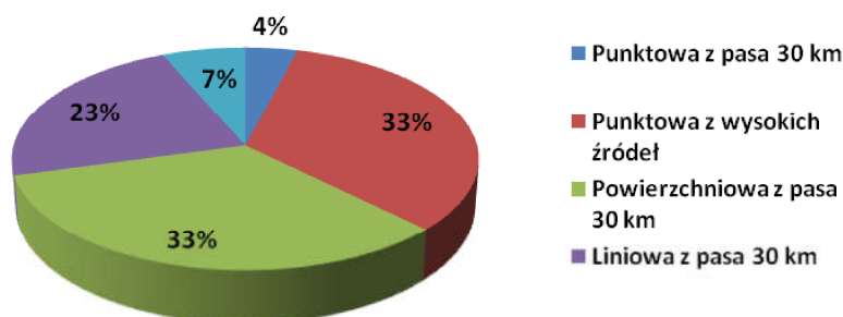
Rysunek 24 Udział procentowy emisji pyłu zawieszzonego PM10 poszczególnych typów poza strefą aglomeracji lubelskiej w 2015 r.
