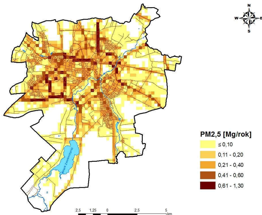
Rysunek 33 Emisja liniowa pyłu zawieszanego PM2,5 z terenu strefy aglomeracji lubelska w 2015 r.
