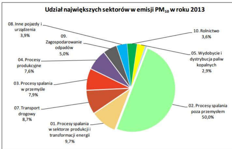
Rysunek 16 Udziały poszczególnych rodzajów emitentów w emisji pyłu zawieszzonego PM 10
