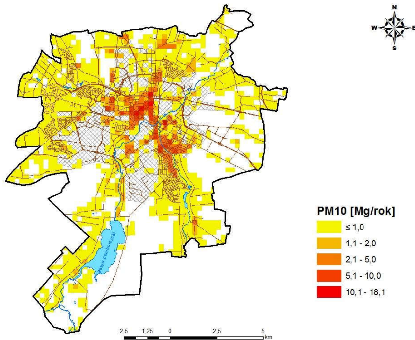
Rysunek 27 Emisja powierzchniowa pyłu zawieszzonego PM10 z terenu strefy aglomeracja lubelska w 2015 r.
