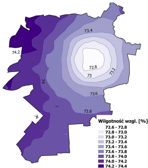
Rysunek 12 Rozkład średniej rocznej wilgotności względnej powietrza wyznaczony przez model WRF/CALMET w strefie aglomeracja lubelska w 2015 r.
