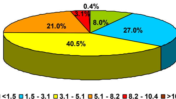
Rysunek 5 Procentowy rozkład prawdopodobieństwa występowania prędkości wiatru w określonych przedziałach w strefie aglomeracja lubelska w 2015 r.
