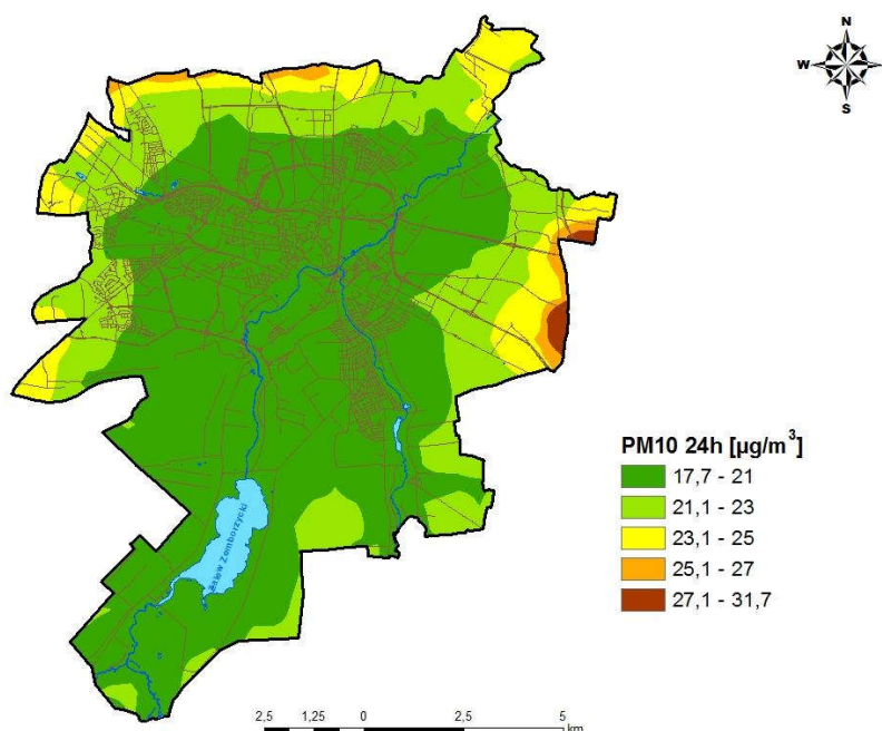
Rysunek 34 Stężenia pyłu zawieszzonego PM10 o okresie uśredniania wyników 24 h w strefie aglomeracja lubelska pochodzące z tła całkowitego w 2015 r.
