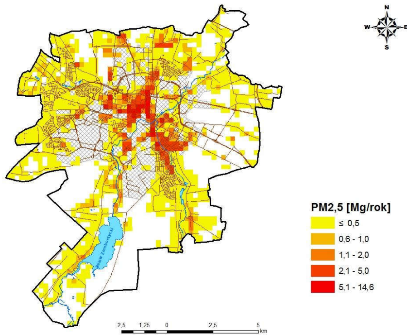
Rysunek 32 Emisja powierzchniowa pyłu zawieszzonego PM2,5 z terenu strefy aglomeracja lubelska w 2015 r.
