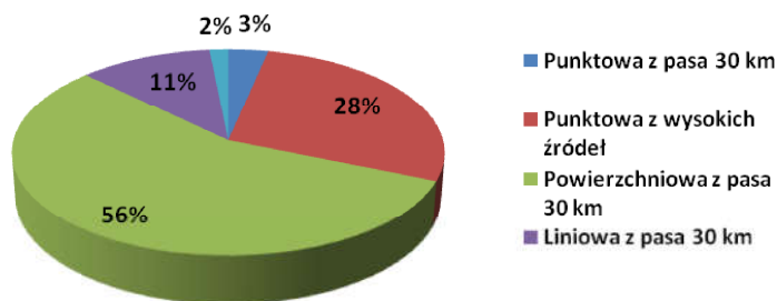
Rysunek 29 Udział procentowy emisji pyłu zawieszzonego PM2,5 poszczególnych typów poza strefą aglomeracja lubelska w 2015 r.
