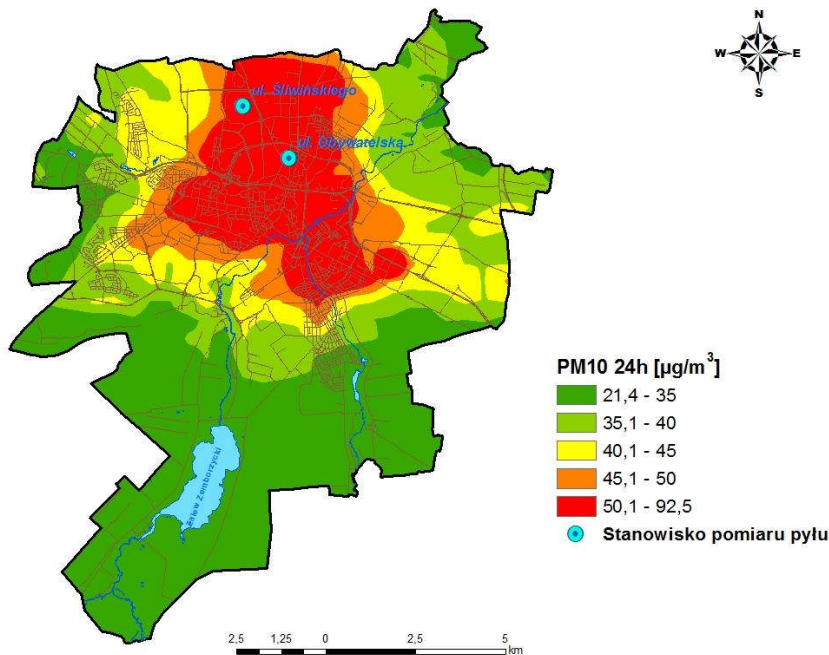
Rysunek 36 Stężenia pyłu zawieszzonego PM10 o okresie uśredniania wyników 24 h w strefie aglomeracja lubelska pochodzące z łącznej emisji wszystkich typów w 2015 r.
