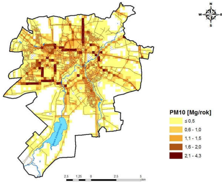
Rysunek 28 Emisja liniowa pyłu zawieszzonego PM10 z terenu strefy aglomeracja lubelska w 2015 r.
