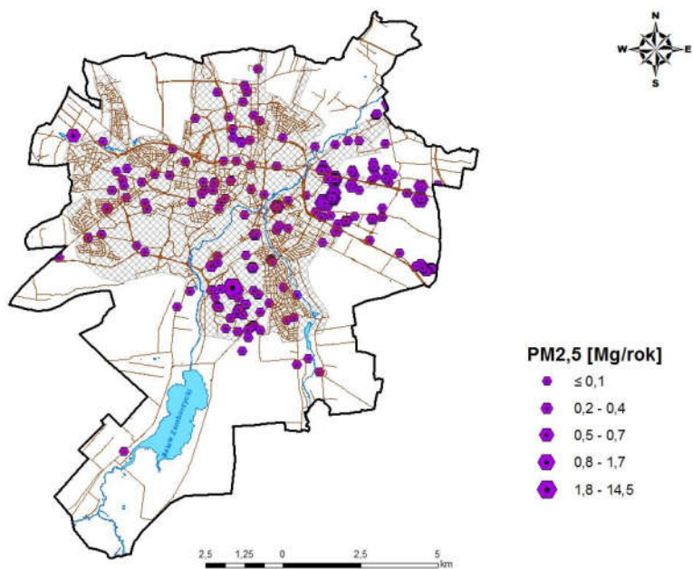
Rysunek 31 Emisja punktowa pyłu zawieszzonego PM2,5 z terenu strefy aglomeracja lubelska w 2015 r.
