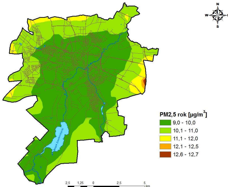
Rysunek 38 Stężenia pyłu zawieszzonego PM2,5 o okresie uśredniania wyników rok w strefie aglomeracja lubelska pochodzące z tła całkowitego w 2015 r.
