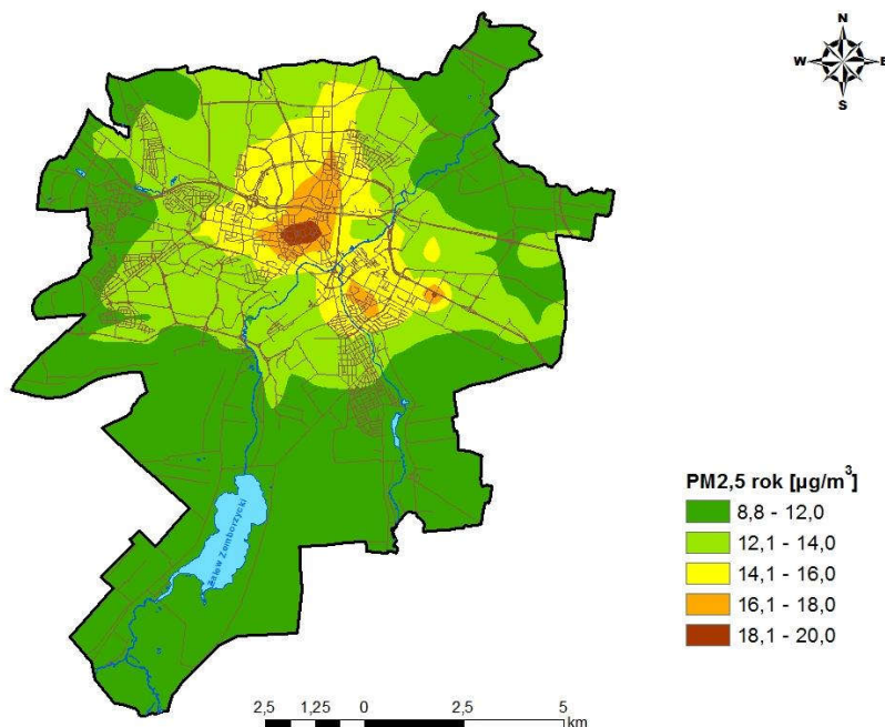
Rysunek 48 Prognozowane stężenia pyłu zawieszony PM2,5 o okresie uśredniania wyników rok w strefie aglomeracja lubelska pochodzące z łącznej emisji wszystkich typów w 2026 r.
