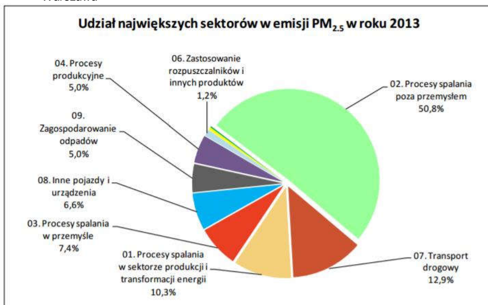
Rysunek 17 Udziały poszczególnych rodzajów emitentów w emisji pyłu zawieszzonego PM 2,5
