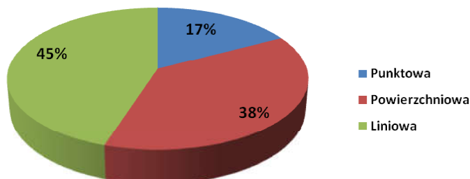
Rysunek 25 Udział procentowy emisji pyłu zawieszzonego PM10 poszczególnych typów w emisji całkowitej ze strefy aglomeracji lubelskiej w 2015 r.
