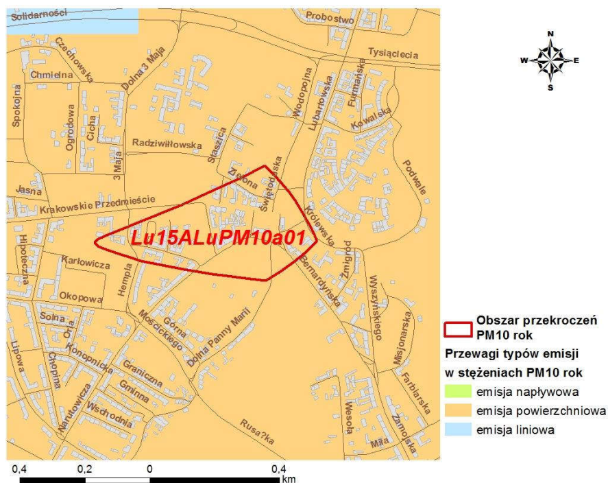
Rysunek 43 Przewagi typów emisji w stężeniach pyłu zawieszanego PM 10 o okresie uśredniania wyników rok Lu15ALuPM10a01 w strefie aglomeracja lubelska w 2015 r.
