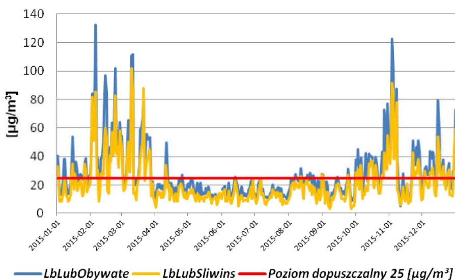
Rysunek 19 Roczny przebieg średnich dobowych wartości pyłu zawieszanego PM2,5 na stanowiskach pomiarowych w strefie aglomeracja lubelska w 2015 r.
