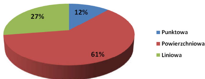
Rysunek 30 Udział procentowy emisji pyłu zawieszzonego PM2,5 poszczególnych typów w emisji całkowitej ze strefy aglomeracja lubelska w 2015 r.
