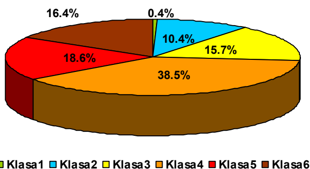
Rysunek 15 Rozkład prawdopodobieństwa występowania klas równowagi atmosfery wyznaczony przez model WRF/CALMET w strefie aglomeracji lubelskiej w 2015 r.
