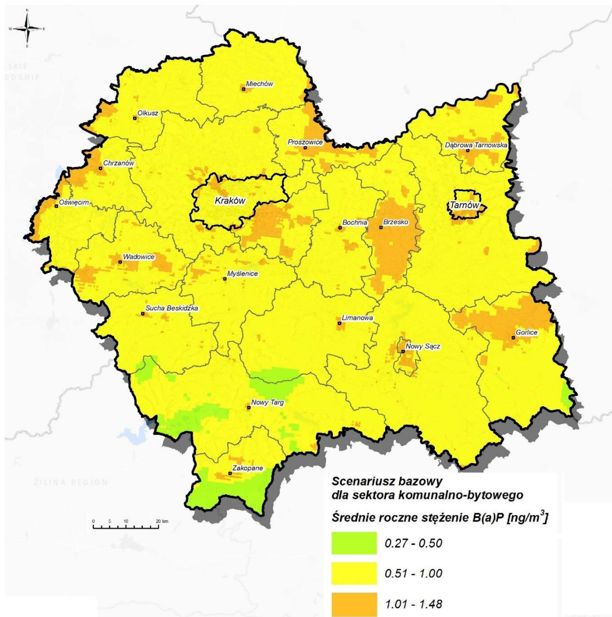
Rysunek 52. Rozkład stężeń średniorocznych pyłu PM 10 na obszarze województwa w roku prognozy 2026 w ramach scenariusza realizacyjnego 143 .
