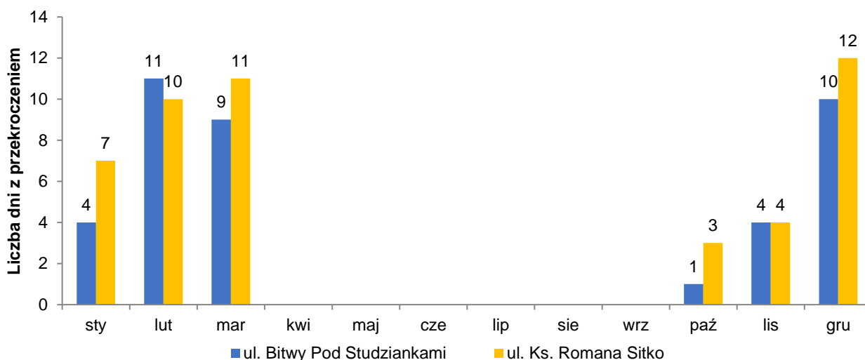
Rysunek 13. Liczba dni z przekroczeniem dopuszczalnego stężenia 24-godz. PM10 w strefie miasto Tarnów w 2021 roku 56
