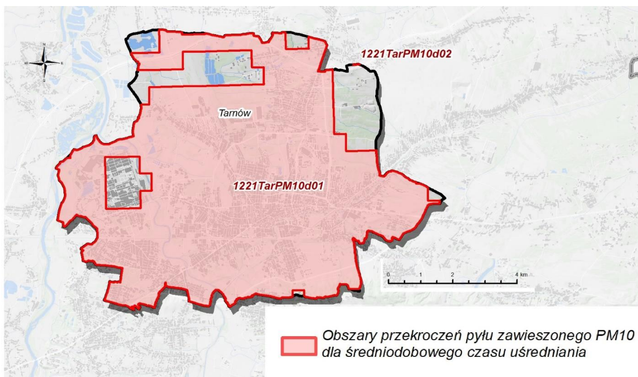
Rysunek 28. Obszar przekroczeń stężeń 24-godzinnych pyłu PM 10 w strefie miasto Tarnów w 2021 roku. 75
