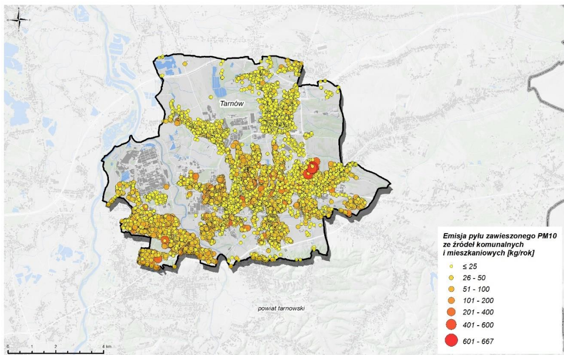
Rysunek 74. Emisja pyłu zawieszonego PM10 ze źródeł komunalno-bytowych w strefie miasto Tarnów w 2021 r.
