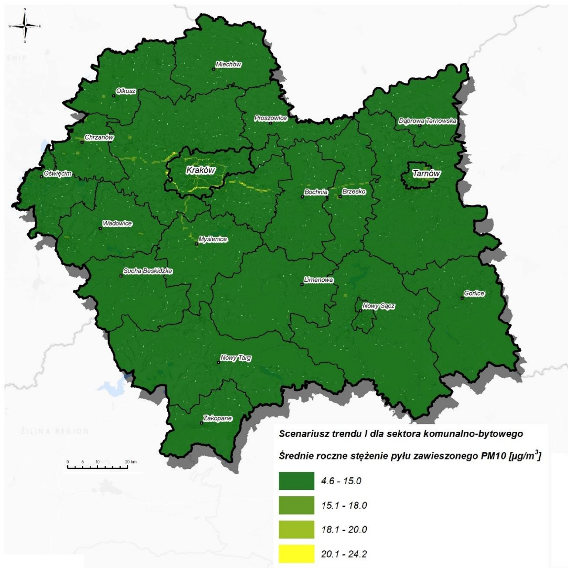
Rysunek 118. Rozkład stężeń średniorocznych pyłu PM10 na obszarze województwa w roku prognozy 2026 w ramach scenariusza trendu 203 .
