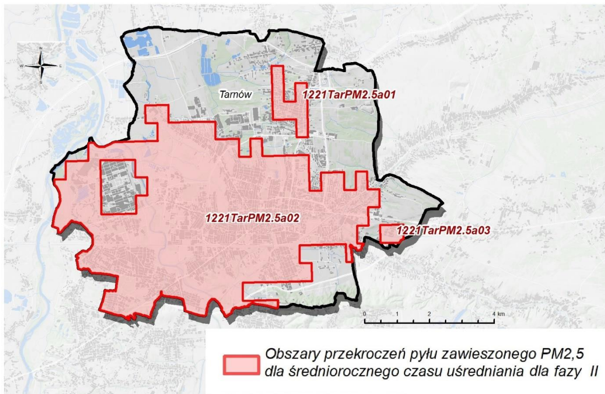
Rysunek 29. Obszar przekroczeń stężeń średniorocznych pyłu PM2,5 w strefie miasto Tarnów w 2021 roku. 76
