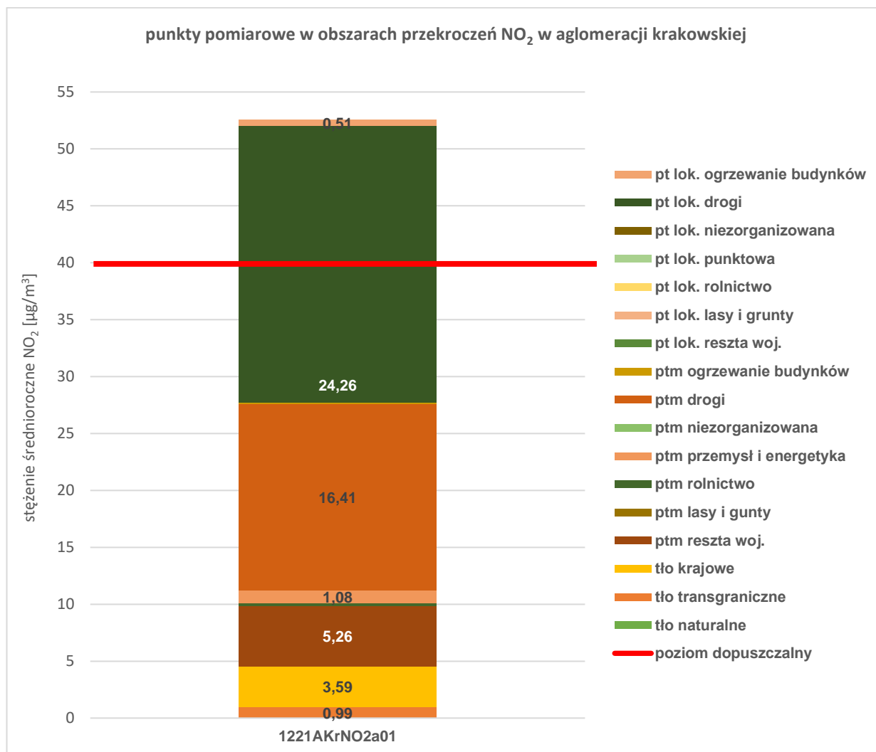
Rysunek 37. Prezentacja poziomów tła regionalnego, tła miejskiego oraz przyrostu tła lokalnego dwutlenku azotu w obszarze przekroczeń w strefie Aglomeracja Krakowska w 2021 roku 95
