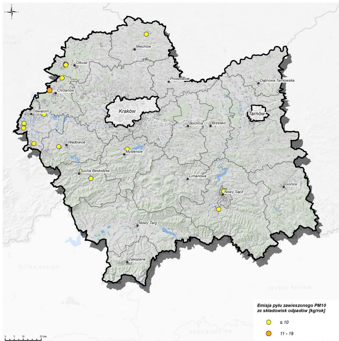
Rysunek 62. Emisja pyłu zawieszonego PM10 ze składowisk odpadów w strefie małopolskiej w 2021 r.
