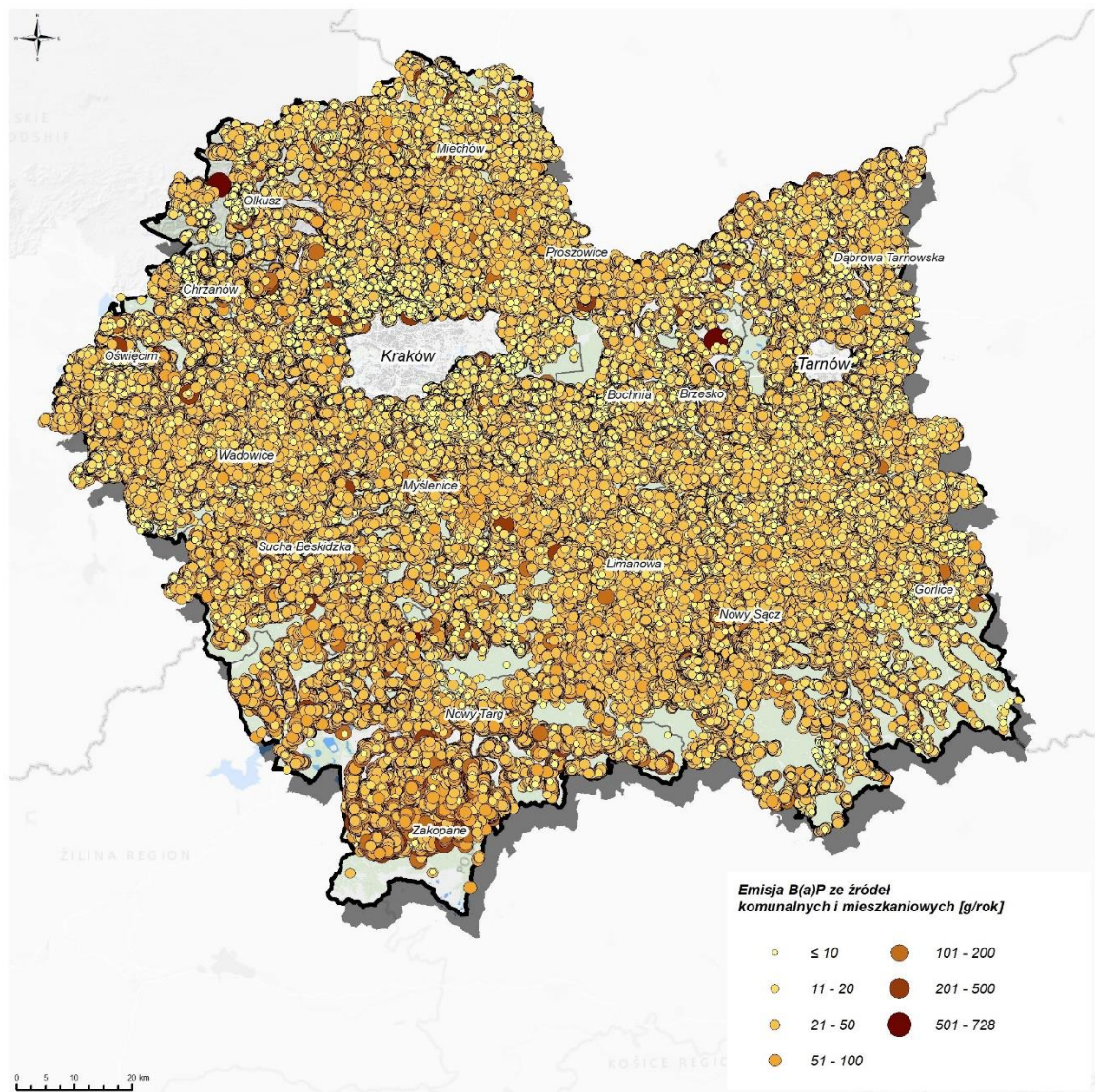
Rysunek 106. Emisja benzo(a)pirenu ze źródeł komunalno-bytowych w strefie małopolskiej w 2021 r.
