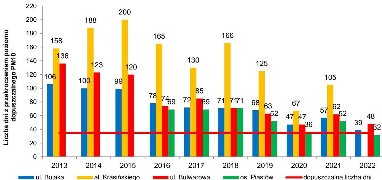
Rysunek 5. Liczba dni z przekroczeniami stężenia 24-godzinowego dla pyłu zawieszonego PM10 na stacjach pomiarowych PMS w strefie Aglomeracja Krakowska w latach 2013-2022 45
