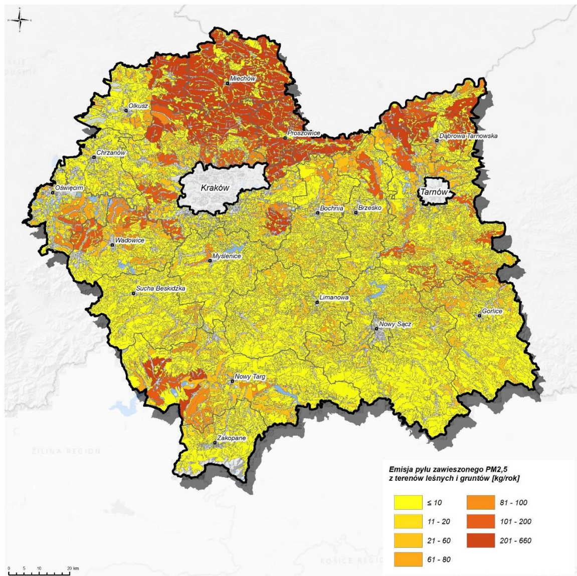
Rysunek 88. Emisja pyłu zawieszonego PM 2,5 ze źródeł rolniczych (uprawy, nawożenie, maszyny rolnicze) w strefie małopolskiej w 2021 r.
