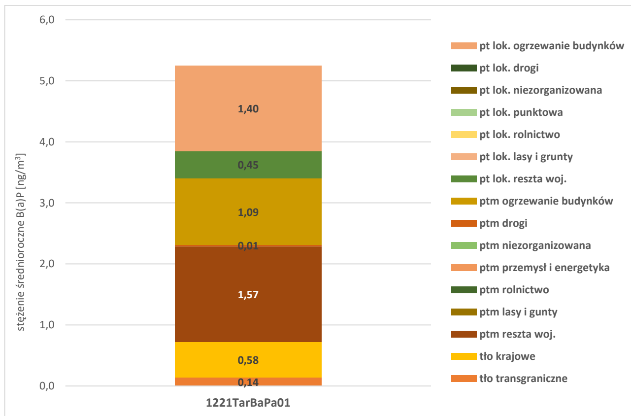
Rysunek 40. Prezentacja poziomów tła regionalnego, tła miejskiego oraz przyrostu tła lokalnego benzo(a)pirenu w obszarze przekroczeń w strefie miasto Tarnów w 2021 roku 101 .
