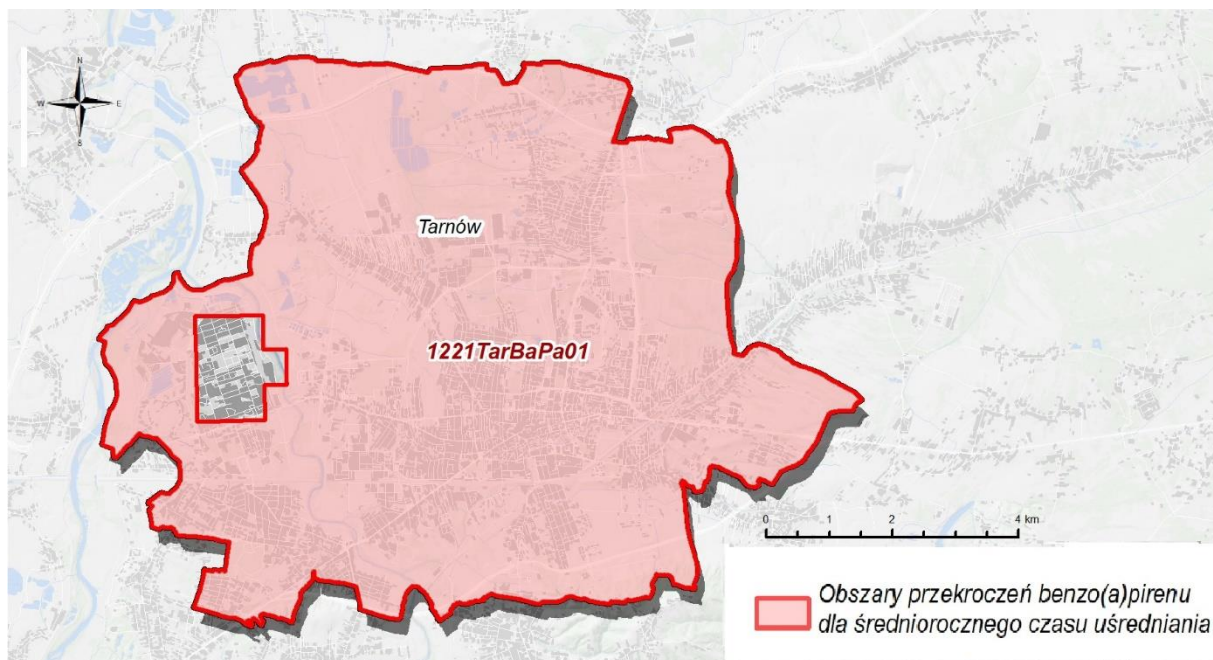
Rysunek 30. Obszar przekroczeń stężeń średniorocznych benzo(a)pirenu w strefie miasto Tarnów w 2021 roku. 77
