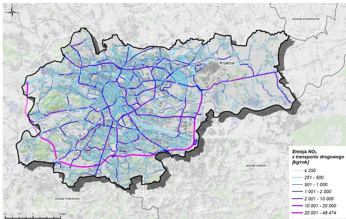
Rysunek 117. Emisja NO 2 ze źródeł transportowych w strefie Aglomeracja Krakowska w 2021 r.
