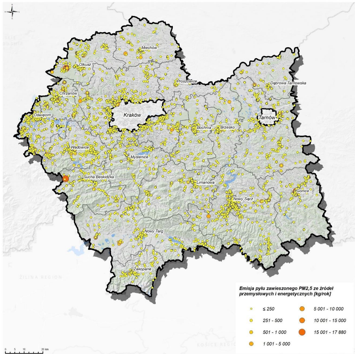
Rysunek 81. Emisja pyłu zawieszonego PM 2,5 ze źródeł przemysłowych i energetycznych w strefie małopolskiej w 2021 r.
