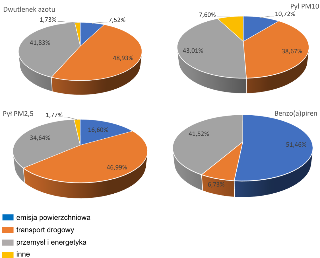
Rysunek 44. Udziały procentowe emisji NO 2 , PM 10 , PM 2,5 oraz benzo(a)pirenu w strefie aglomeracja krakowska w 2021 roku. 111
