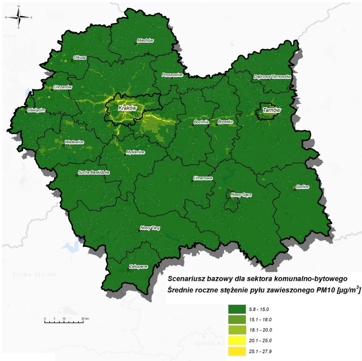
Rysunek 47. Rozkład stężeń średniorocznych pyłu PM10 na obszarze województwa w roku prognozy 2026 w ramach scenariusza bazowego 137 .
