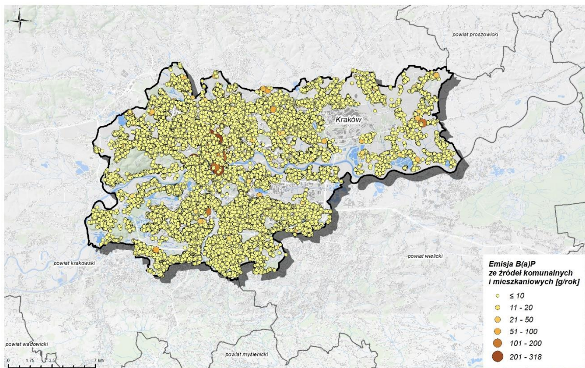
Rysunek 110. Emisja benzo(a)pirenu ze źródeł komunalno-bytowych w strefie Aglomeracja Krakowska w 2021 r.
