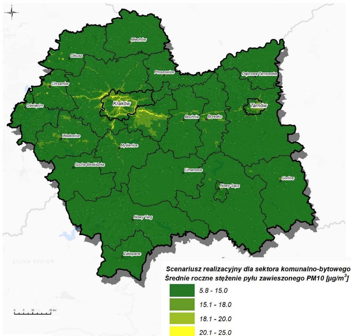
Rysunek 50. Rozkład stężeń średniorocznych pyłu PM10 na obszarze województwa w roku prognozy 2026 w ramach scenariusza realizacyjnego 141 .
