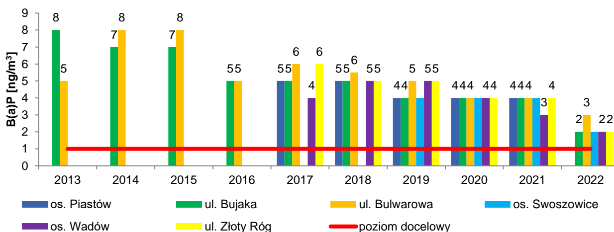
Rysunek 10. Stężenia średnioroczne benzo(a)pirenu na stacjach pomiarowych PMS w strefie Aglomeracji Krakowskiej w latach 2013-2022 52
