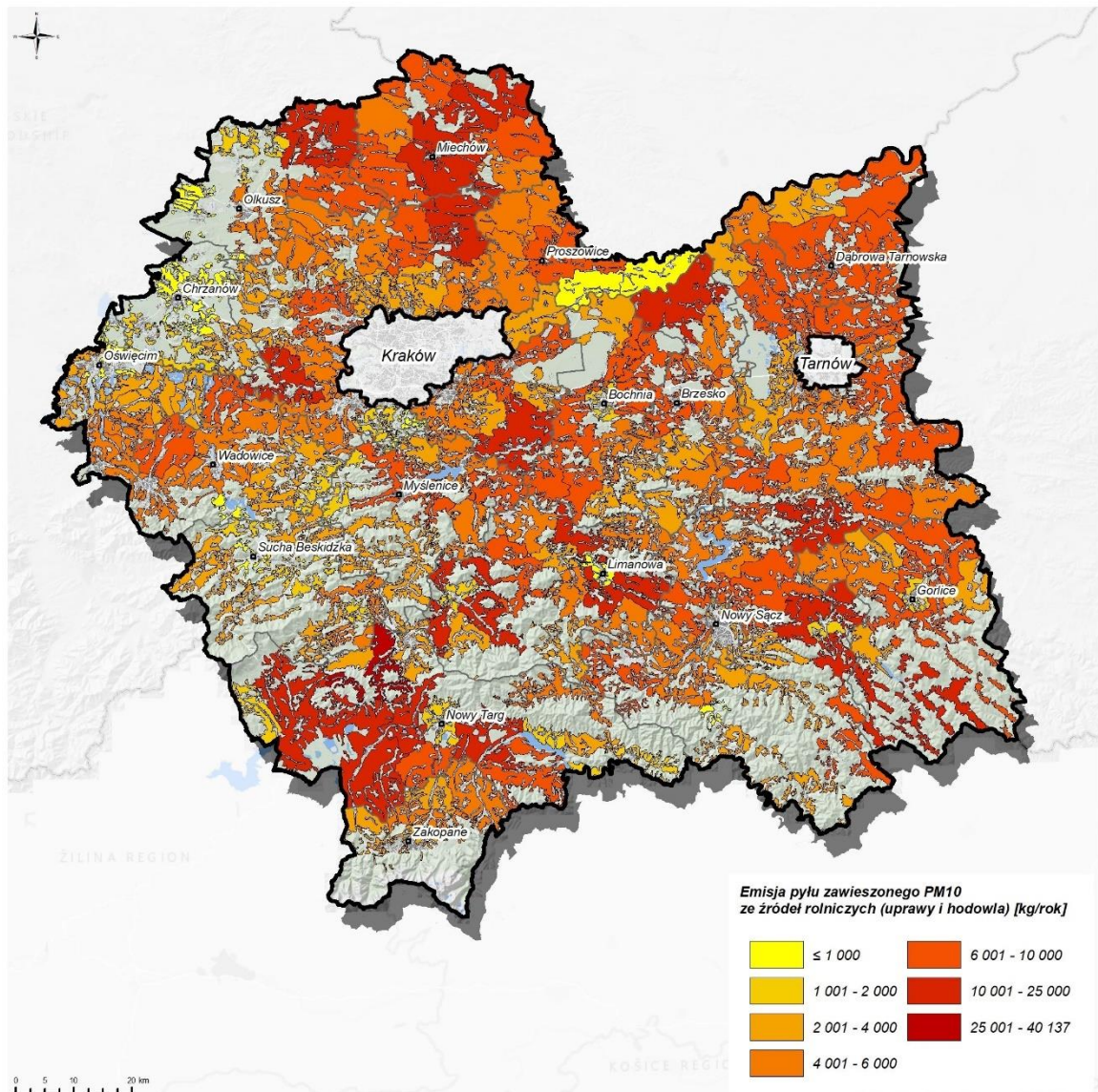
Rysunek 63. Emisja pyłu zawieszonego PM10 ze źródeł rolniczych (hodowla) w strefie małopolskiej w 2021 r.
