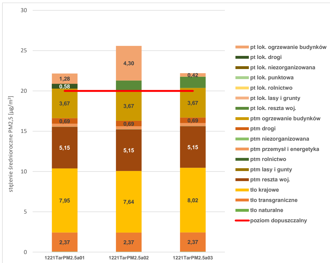
Rysunek 39. Prezentacja poziomów tła regionalnego, tła miejskiego oraz przyrostu tła lokalnego pyłu PM 2,5 w obszarze przekroczeń w strefie miasto Tarnów w 2021 roku 99 .
