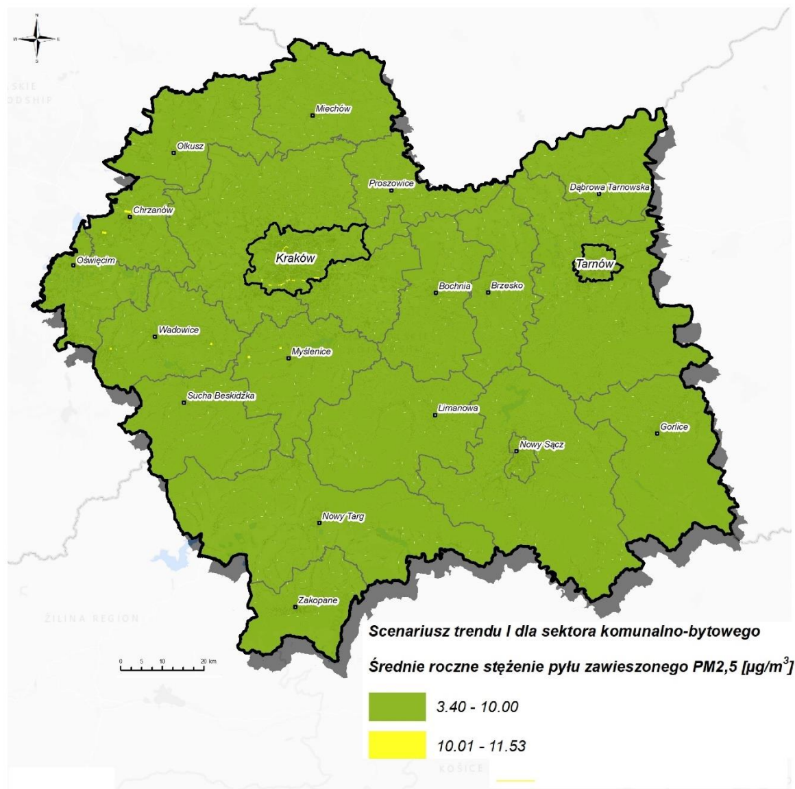
Rysunek 119. Rozkład stężeń średniorocznych pyłu PM 2,5 na obszarze województwa w roku prognozy 2026 w ramach scenariusza trendu P 04 .
