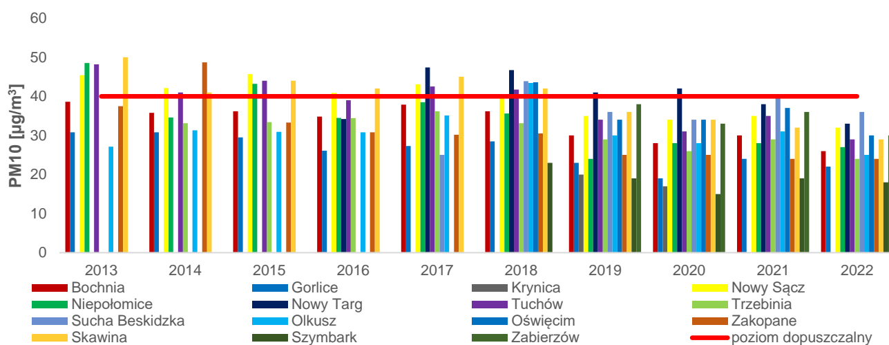
Rysunek 16. Stężenia średnioroczne pyłu PM10 na stacjach pomiarowych PMS 60 w strefie małopolskiej w latach 2013-2022 60
