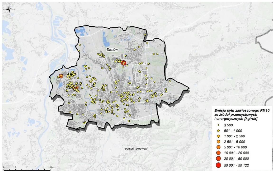
Rysunek 73. Emisja pyłu zawieszonego PM10 ze źródeł przemysłowych i energetycznych w strefie miasto Tarnów w 2021 r.
