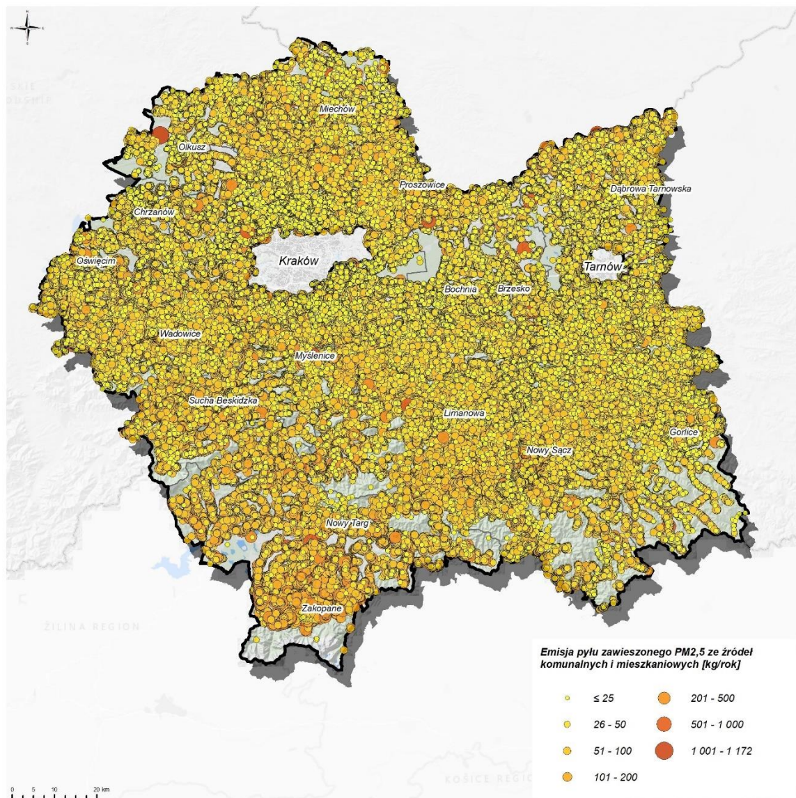
Rysunek 82. Emisja pyłu zawieszonego PM 2,5 ze źródeł komunalno-bytowych w strefie małopolskiej w 2021 r.
