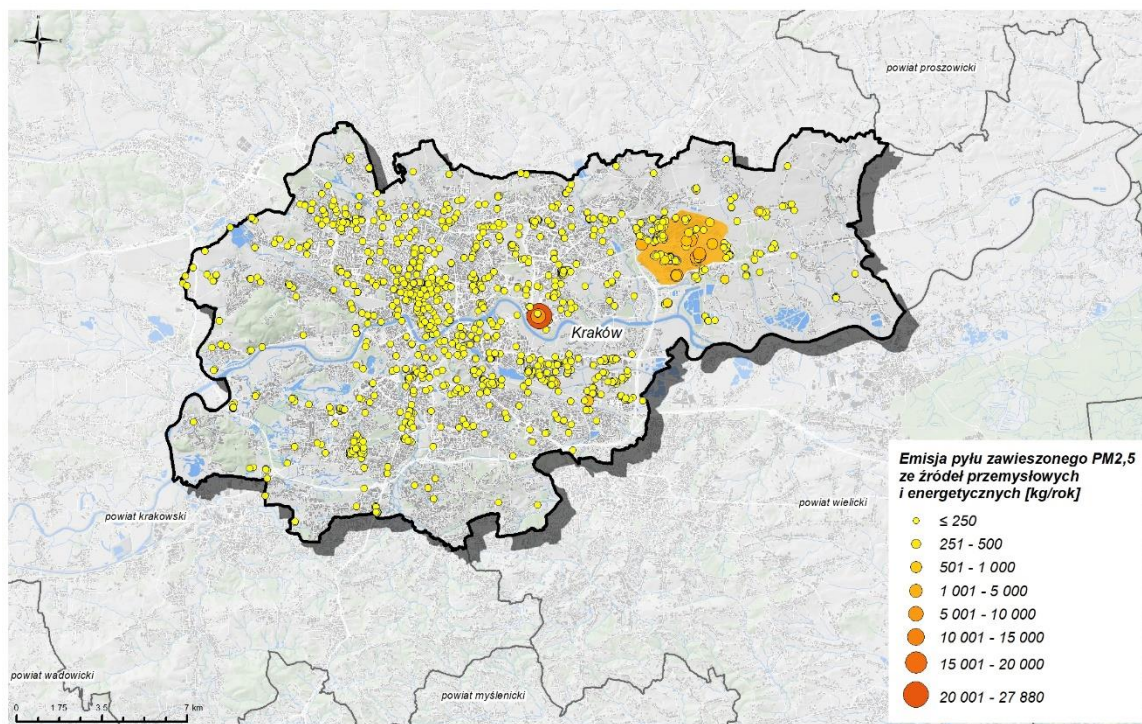
Rysunek 89. Emisja pyłu zawieszonego PM 2,5 ze źródeł przemysłowych i energetycznych w strefie Aglomeracja Krakowska w 2021 r.
