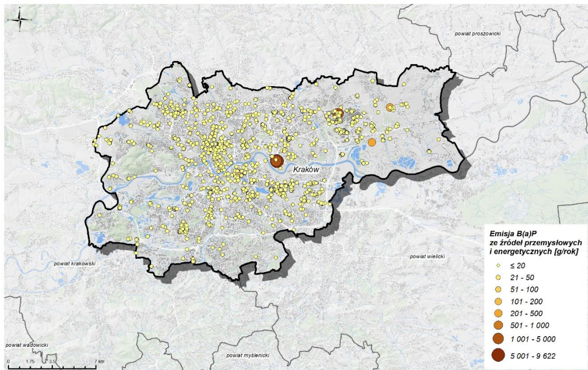
Rysunek 109. Emisja benzo(a)pirenu ze źródeł przemysłowych i energetycznych w strefie Aglomeracja Krakowska w 2021 r.
