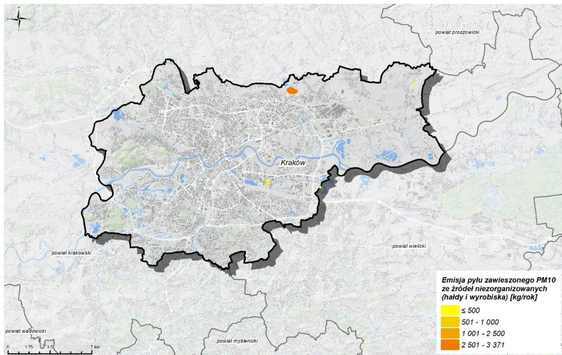
Rysunek 67. Emisja pyłu zawieszonego PM10 ze źródeł niezorganizowanych (kopalnie kruszyw i wyrobiska) w strefie Aglomeracja Krakowska w 2021 r.
