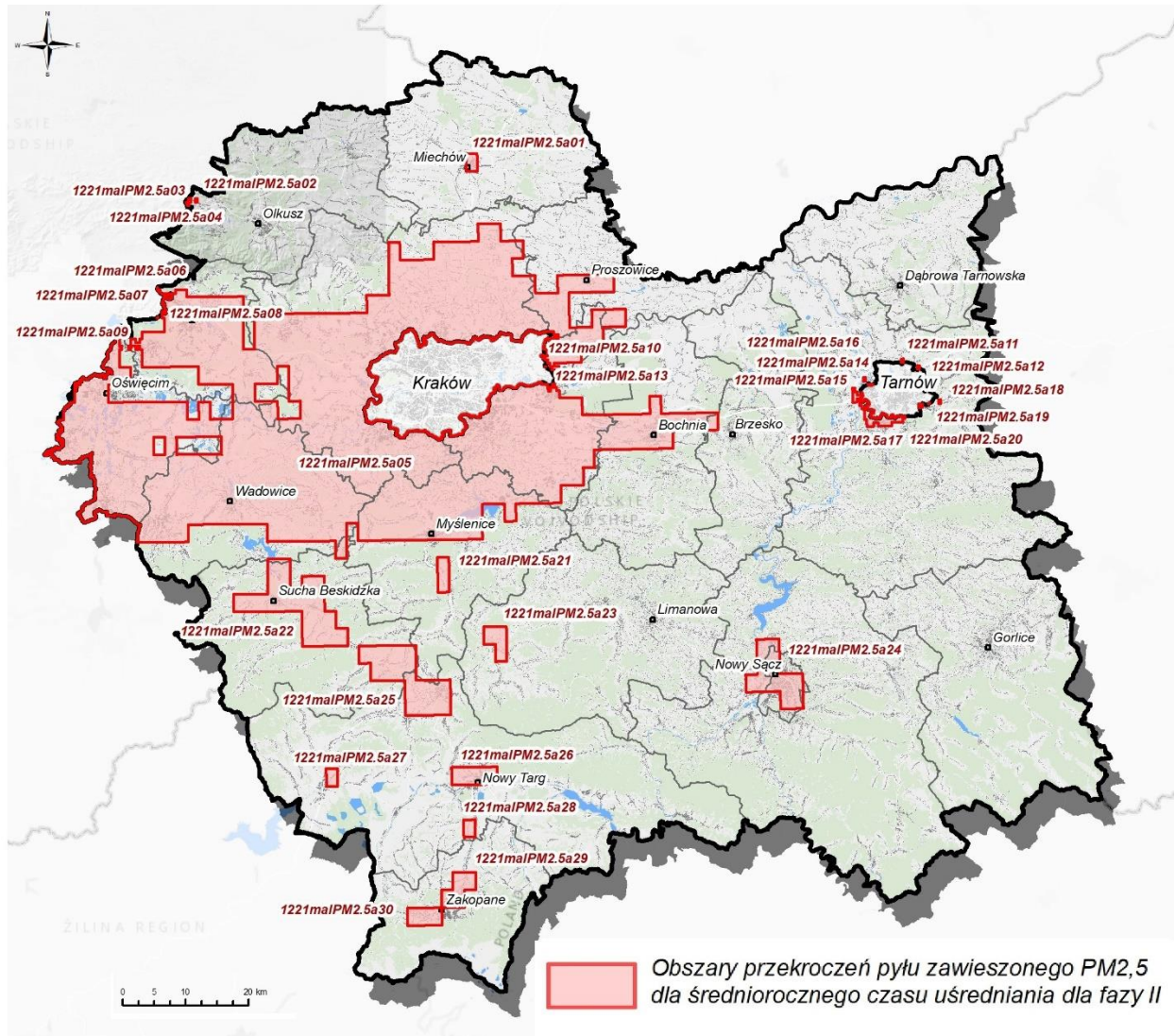
Rysunek 32. Obszar przekroczeń stężeń średniorocznych pyłu PM 2,5 w strefie małopolskiego w 2021 roku. 81
