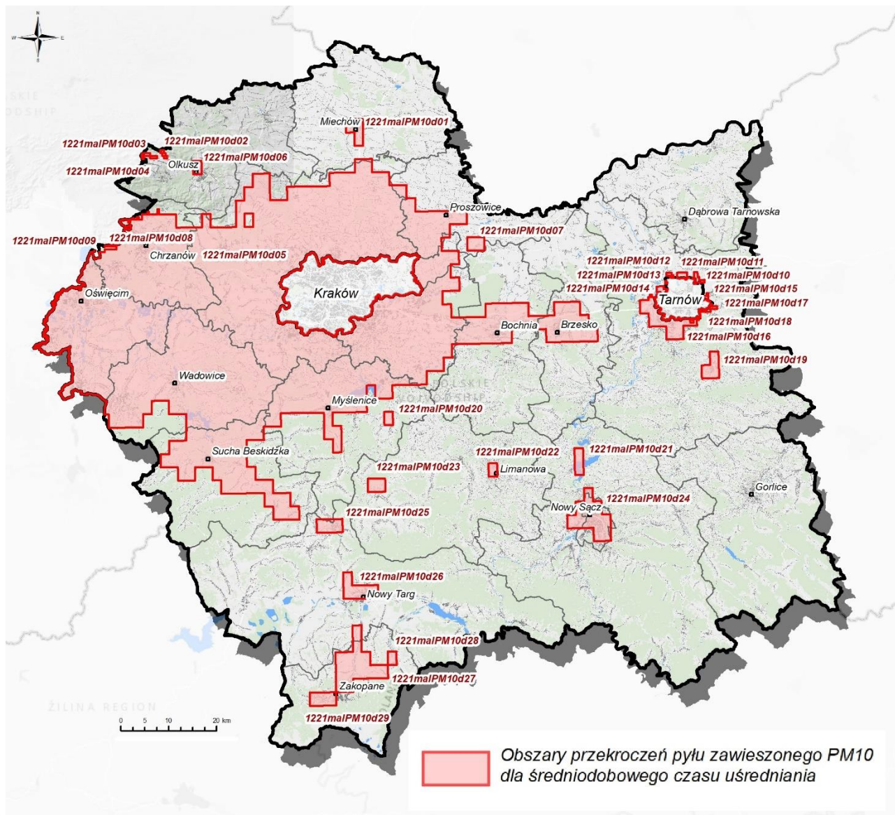
Rysunek 31. Obszary przekroczeń stężeń 24-godzinnych pyłu PM10 w strefie małopolskiej w 2021 roku. 79
