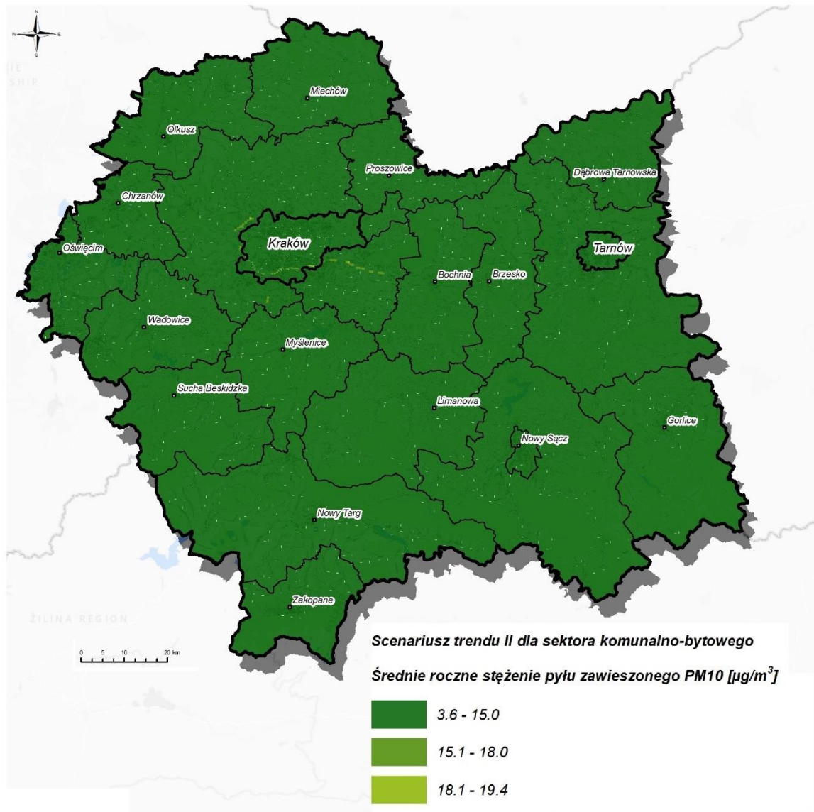
Rysunek 121. Rozkład stężeń średniorocznych pyłu PM10 na obszarze województwa w roku prognozy 2026 w ramach scenariusza trendu II 206 .
