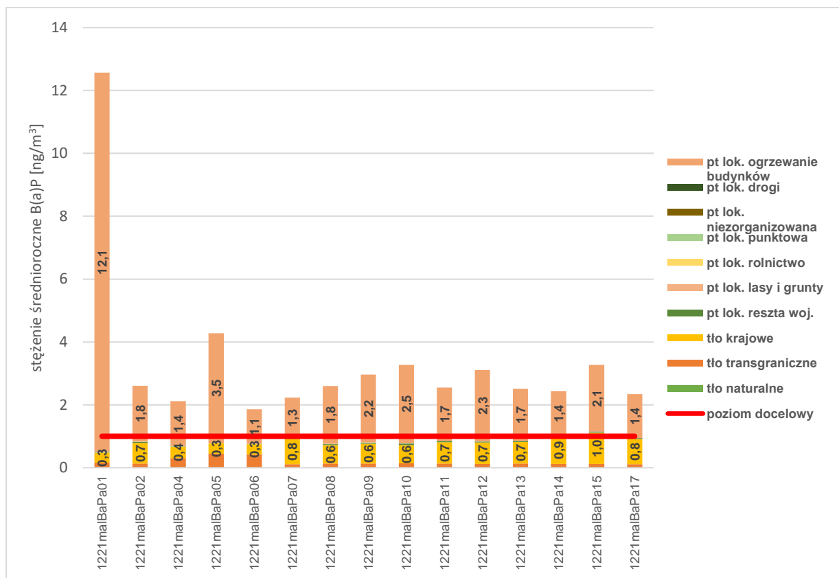
Rysunek 43. Prezentacja poziomów tła regionalnego, tła miejskiego oraz przyrostu tła lokalnego benzo(a)pirenu w obszarze przekroczeń w strefie małopolskiej w 2021 roku 107 .
