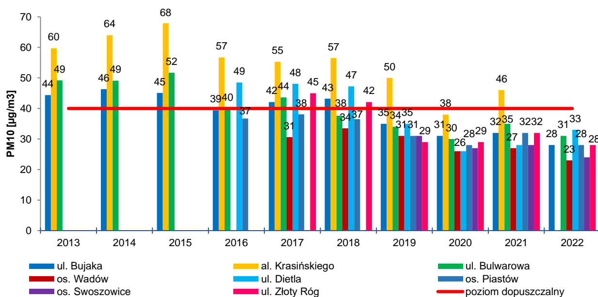
Rysunek 4. Stężenia średnioroczne pyłu PM10 na stacjach pomiarowych PMŚ w strefie Aglomeracja Krakowska w latach 2013-2022 44
