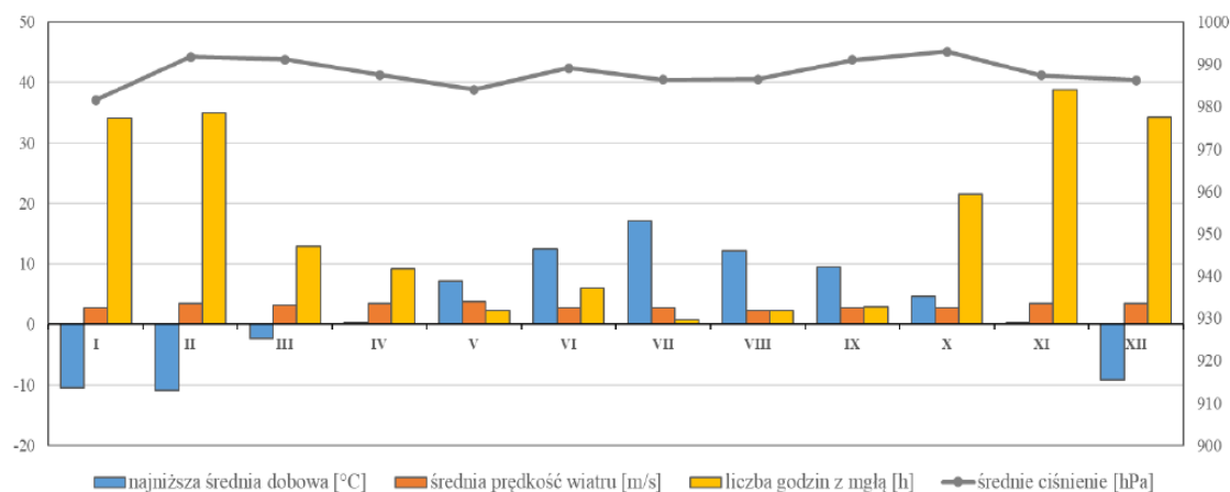
Rysunek 54. Miesięczny rozkład parametrów mogących sprzyjać powstawaniu epizodów wysokich stężeń w Krakowie w 2021 roku. 195
