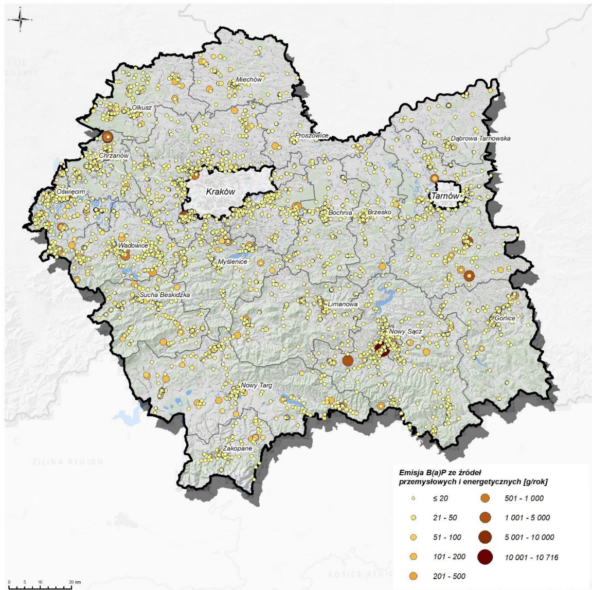
Rysunek 105. Emisja benzo(a)pirenu ze źródeł przemysłowych i energetycznych w strefie małopolskiej w 2021 r.
