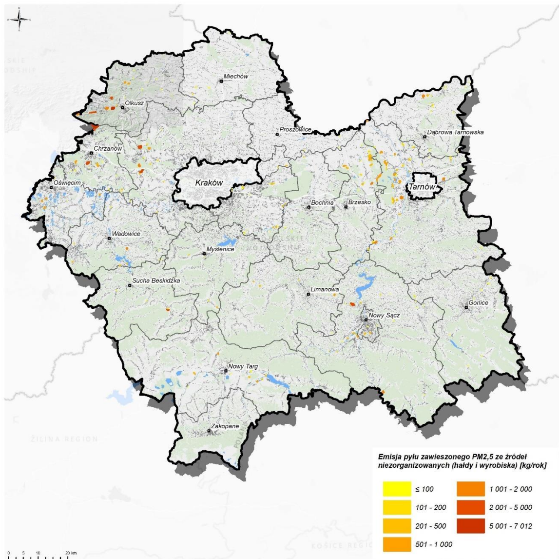
Rysunek 83. Emisja pyłu zawieszonego PM 2,5 ze źródeł niezorganizowanych w strefie małopolskiej w 2021 r.
