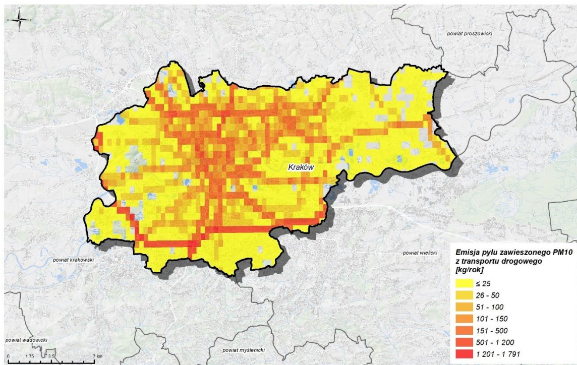
Rysunek 68. Emisja pyłu zawieszonego PM10 z transportu drogowego w strefie Aglomeracja Krakowska w 2021 r.
