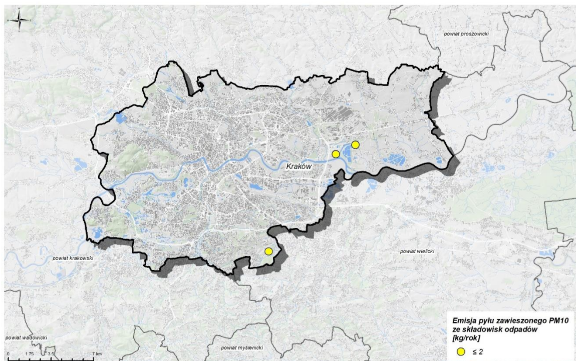
Rysunek 70. Emisja pyłu zawieszonego PM10 ze składowisk odpadów w strefie Aglomeracja Krakowska w 2021 r.
