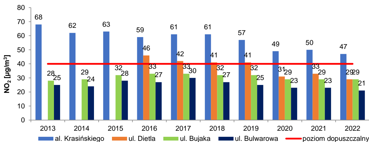
Rysunek 3. Stężenia średnioroczne dwutlenku azotu ( \text{NO}_2 ) na stacjach pomiarowych PMŚ w strefie Aglomeracja Krakowska w latach 2013-2022 42
