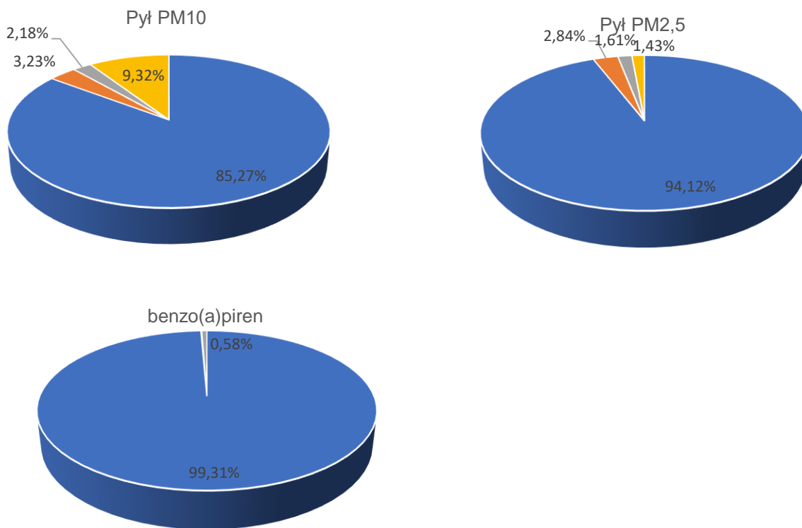
Rysunek 45. Udziały procentowe emisji PM10, PM2,5 oraz benzo(a)pirenu w strefie miasto Tarnobrzeg w 2021 roku. 112
