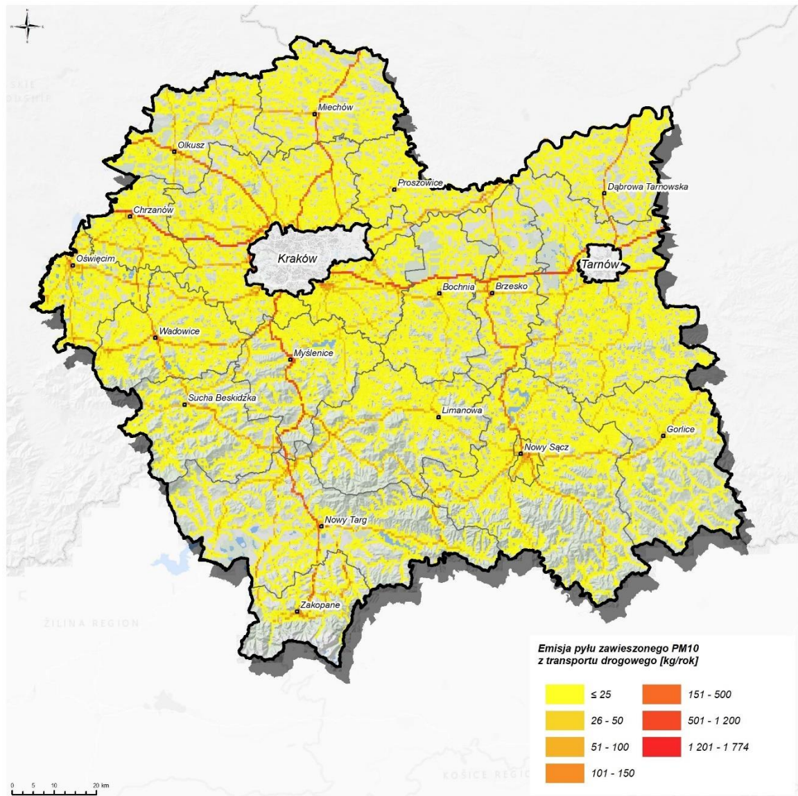
Rysunek 60. Emisja pyłu zawieszonego PM10 z transportu drogowego w strefie małopolskiej w 2021 r.
