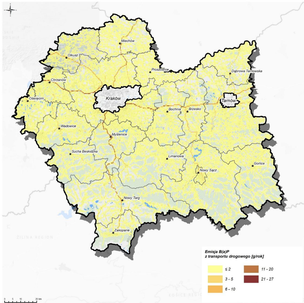
Rysunek 107. Emisja benzo(a)pirenu z transportu drogowego w strefie małopolskiej w 2021 r.
