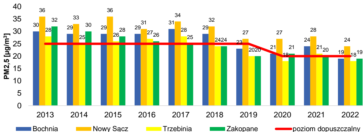
Rysunek 21. Stężenia średnioroczne pyłu PM 2,5 na stacjach pomiarowych PMŚ w strefie małopolskiej w latach 2013-2022 66
