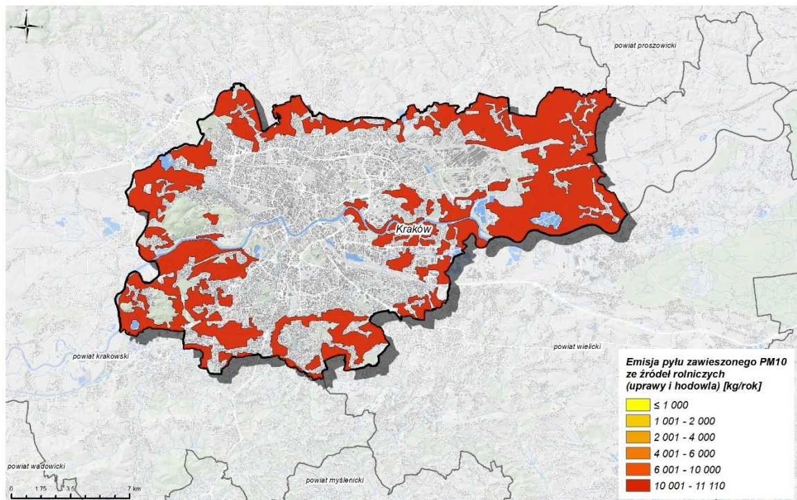
Rysunek 71. Emisja pyłu zawieszonego PM10 ze źródeł rolniczych (hodowla) w strefie Aglomeracja Krakowska w 2021 r.
