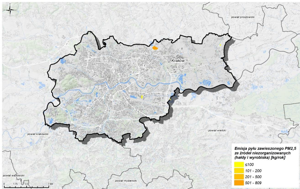
Rysunek 91. Emisja pyłu zawieszonego PM2,5 ze źródeł niezorganizowanych w strefie Aglomeracja Krakowska w 2021 r.
