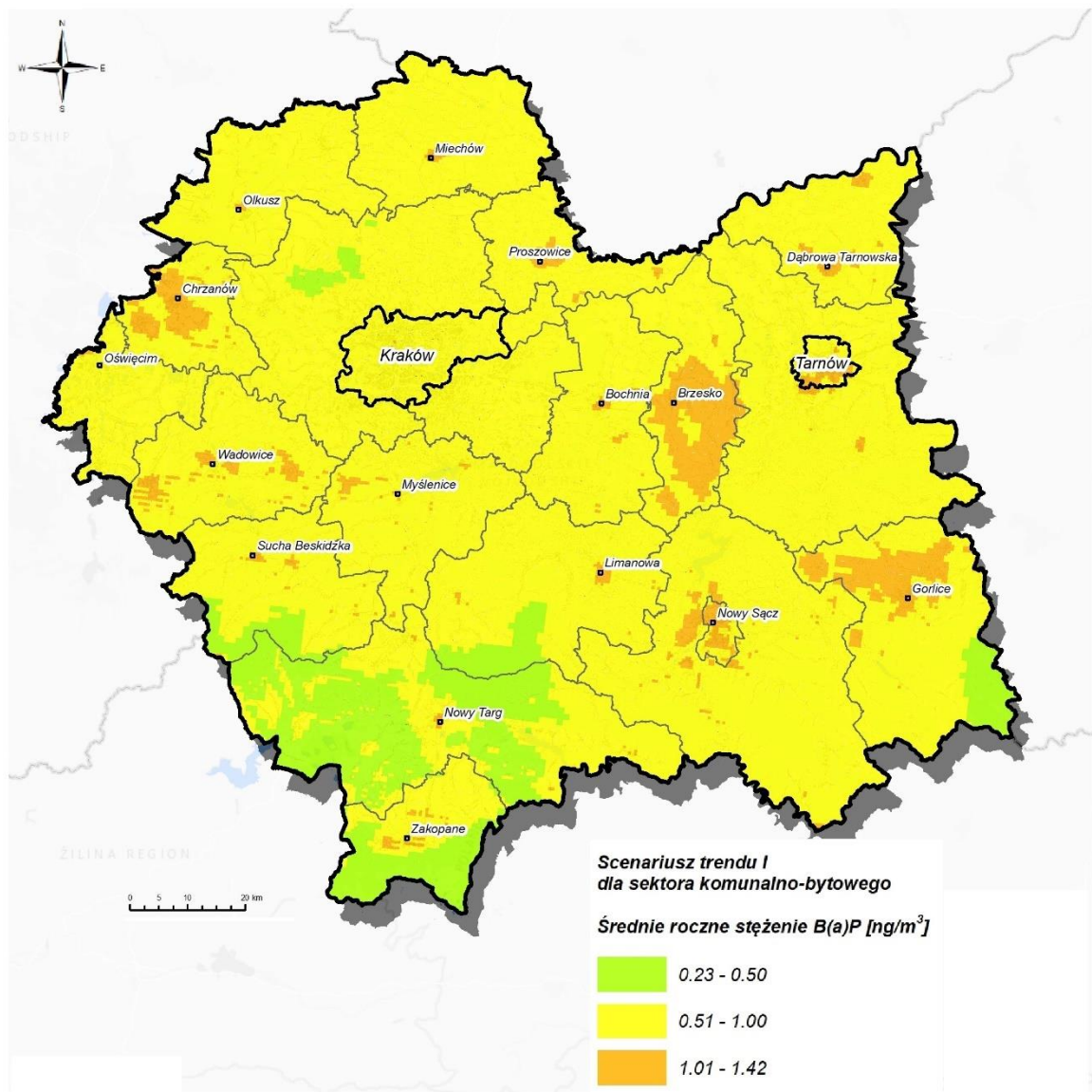
Rysunek 120. Rozkład stężeń średniorocznych benzo(a)pirenu na obszarze województwa w roku prognozy 2026 w ramach scenariusza trendu P 05 .
