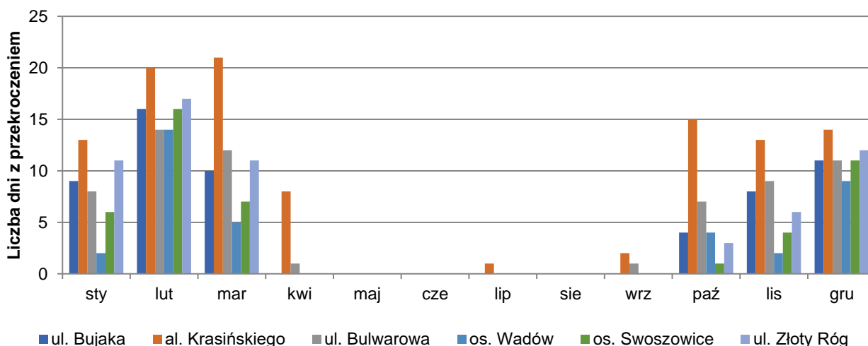
Rysunek 6. Liczba dni z przekroczeniem dopuszczalnego stężenia 24-godz. PM10 w strefie Aglomeracja Krakowska w 2021 roku 46
