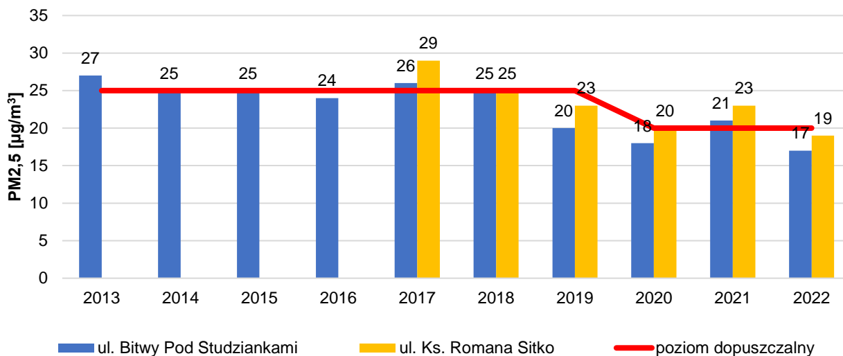
Rysunek 14. Stężenia średnioroczne pyłu PM 2,5 na stacjach pomiarowych PMS w strefie miasto Tarnów w latach 2013-2022 57
