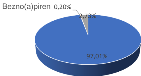
Rysunek 45. Udziały procentowe emisji PM10, PM2,5 oraz benzo(a)pirenu w strefie miasto Tarnobrzeg w 2021 roku. 112
