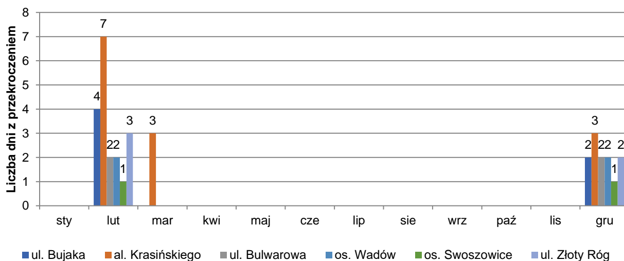
Rysunek 7. Liczba dni ze stężeniem średniodobowym pyłu PM 10 powyżej poziomu informowania społeczeństwa (100 µg/m 3 ) na stacjach tła miejskiego w Aglomeracji Krakowskiej w 2021 roku. 47
