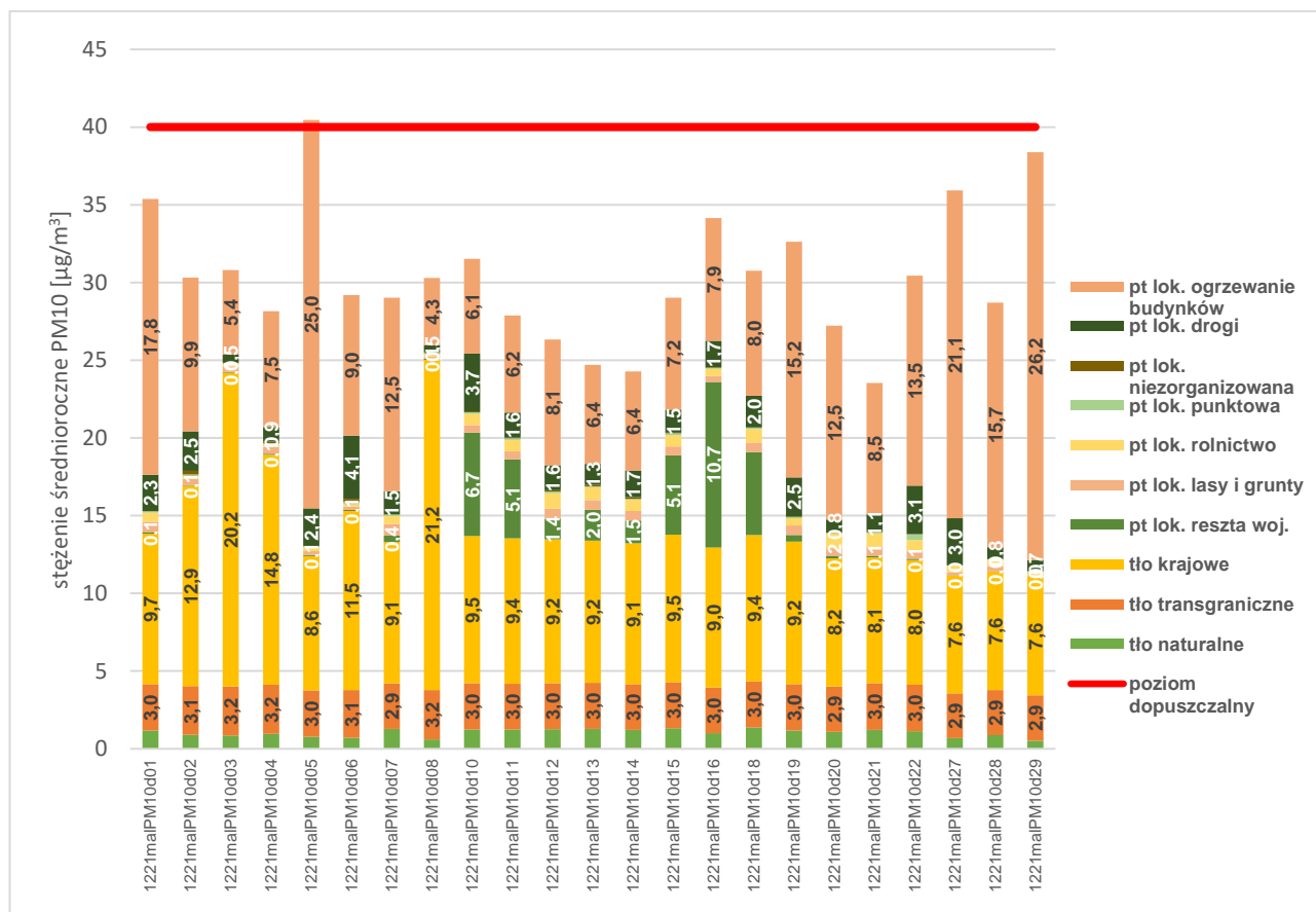
Rysunek 41. Prezentacja poziomów tła regionalnego, tła miejskiego oraz przyrostu tła lokalnego pyłu PM10 w obszarze przekroczeń w strefie małopolskiej w 2021 roku 103 .
