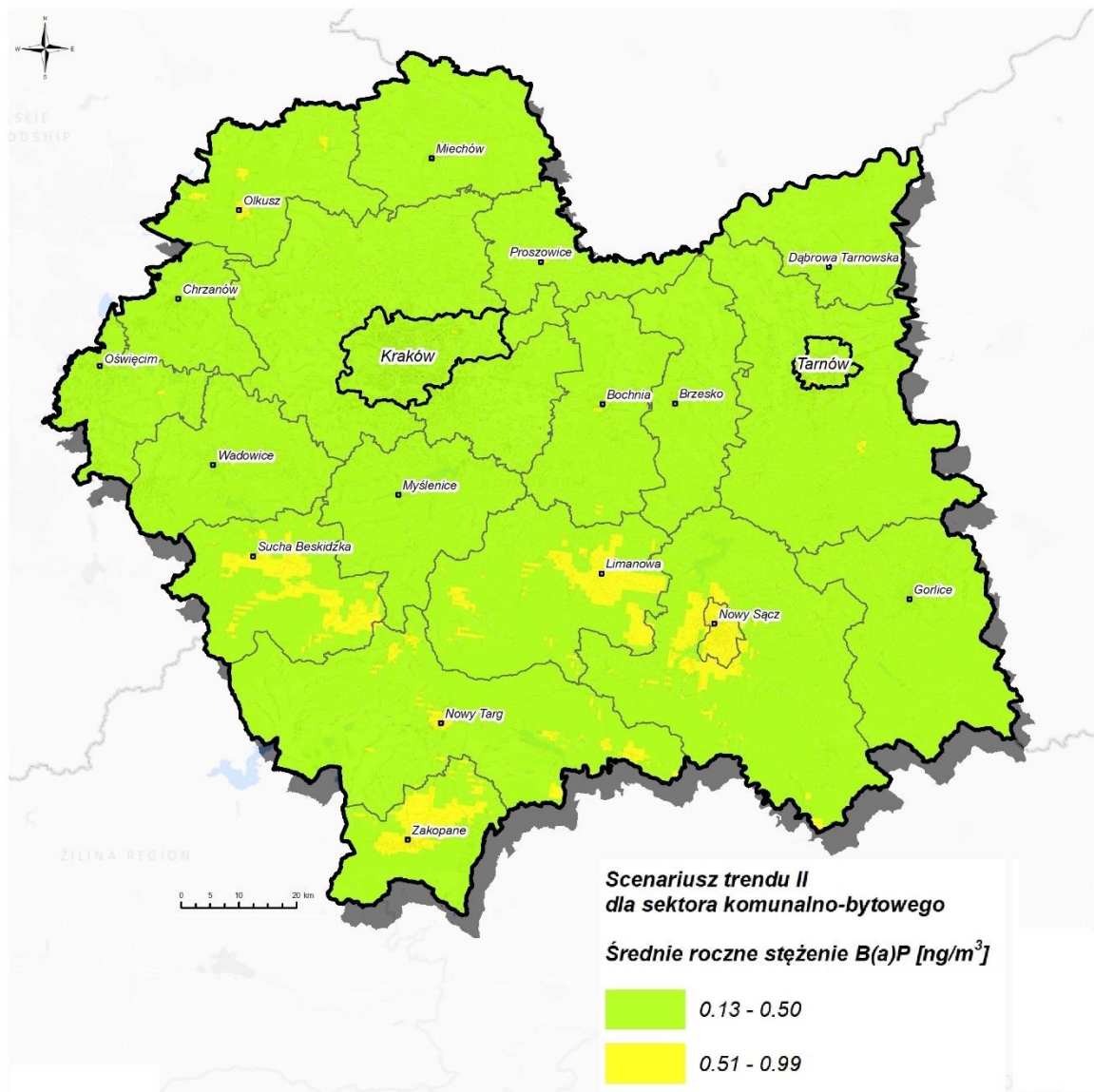
Rysunek 123. Rozkład stężeń średniorocznych benzo(a)pirenu na obszarze województwa w roku prognozy 2026 w ramach scenariusza trendu II 208 .
