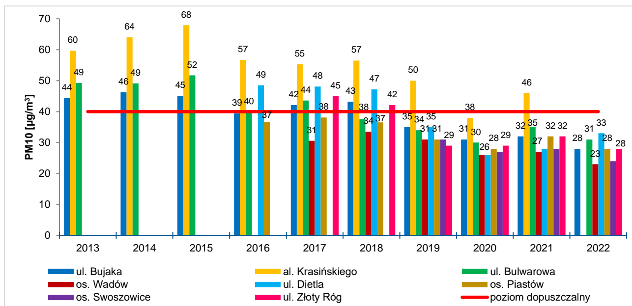
Rysunek 2. Stężenia średnioroczne pyłu PM10 w strefie Aglomeracji Krakowska. 3
