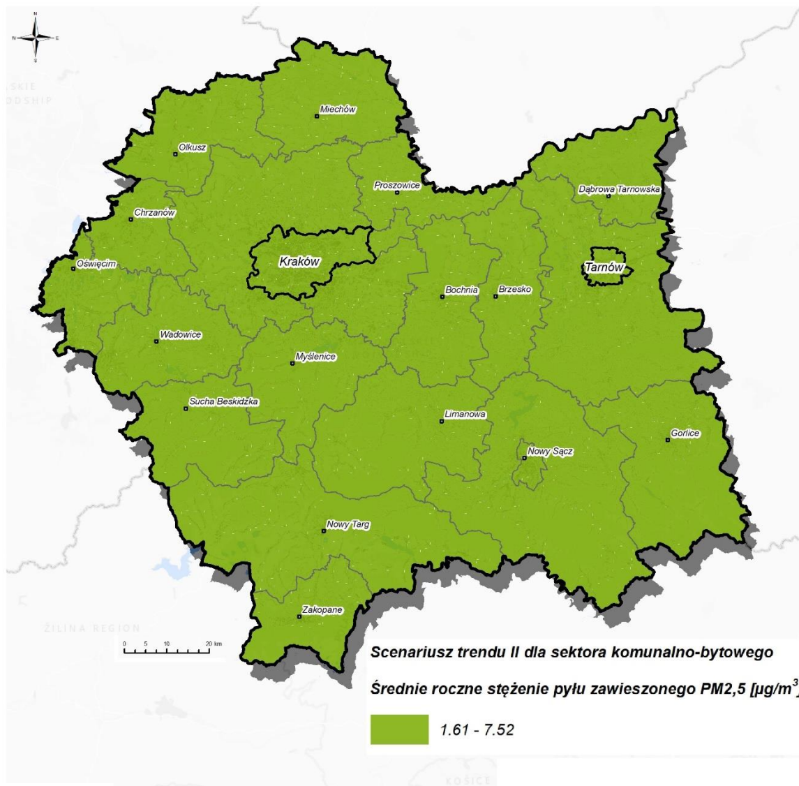
Rysunek 122. Rozkład stężeń średniorocznych pyłu PM 2,5 na obszarze województwa w roku prognozy 2026 w ramach scenariusza trendu II 207 .
