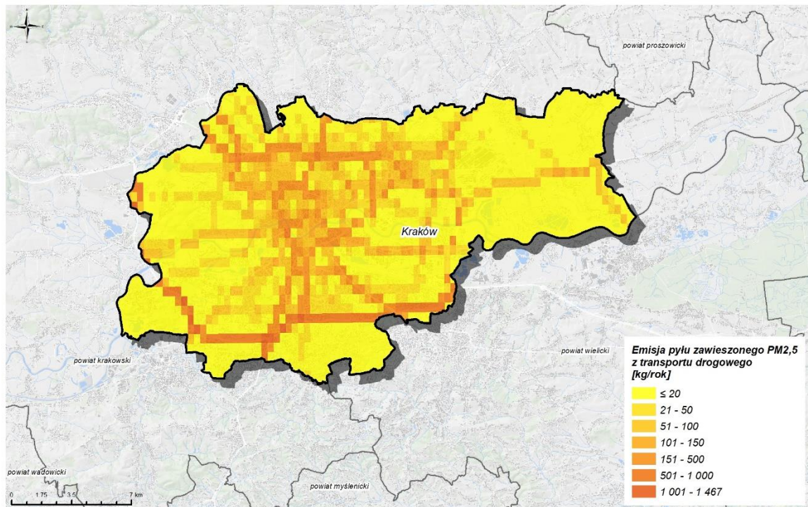
Rysunek 92. Emisja pyłu zawieszonego PM2,5 z transportu drogowego w strefie Aglomeracja Krakowska w 2021 r.
