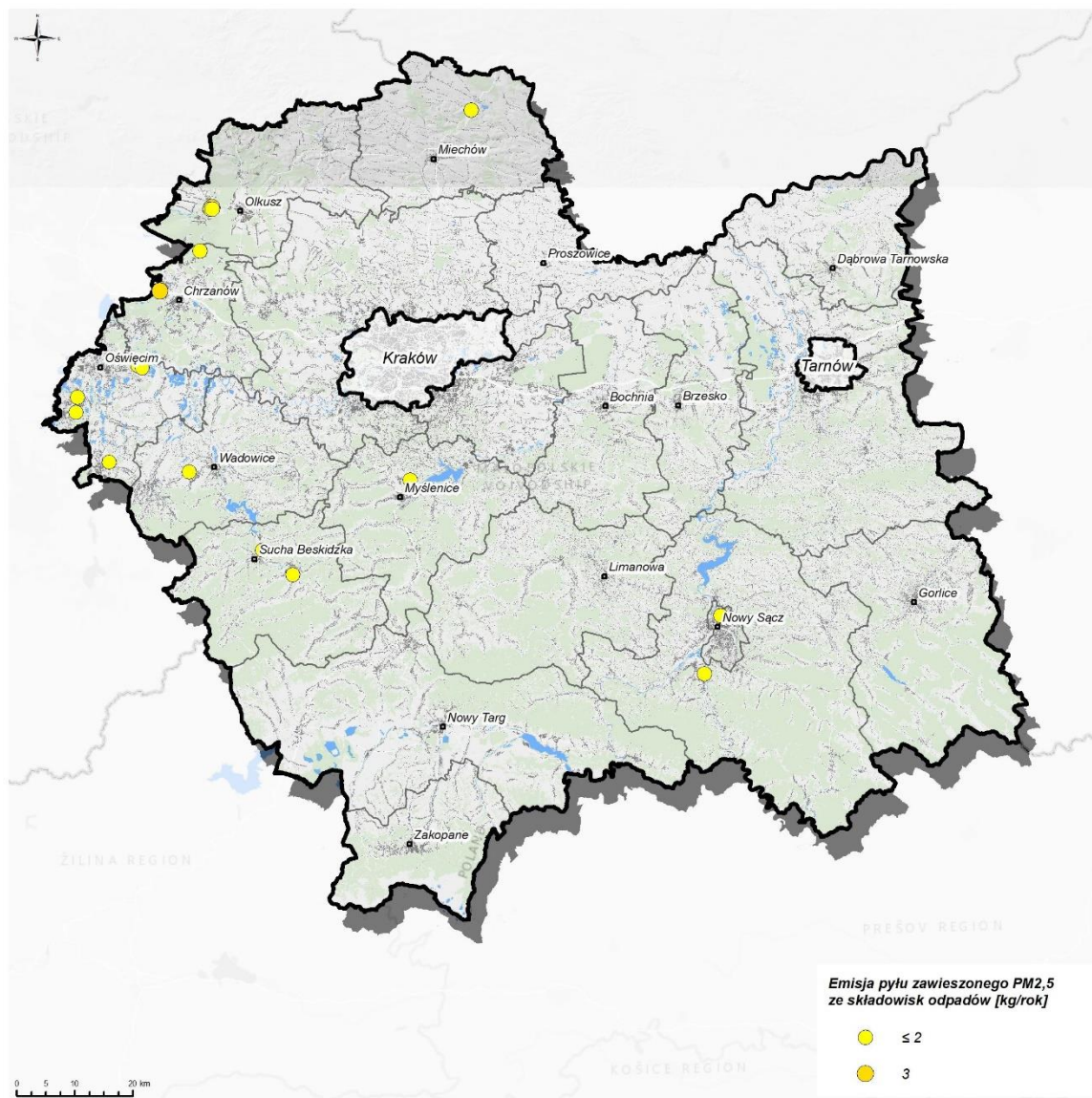
Rysunek 86. Emisja pyłu zawieszonego PM 2,5 ze składowisk odpadów w strefie małopolskiej w 2021 r.
