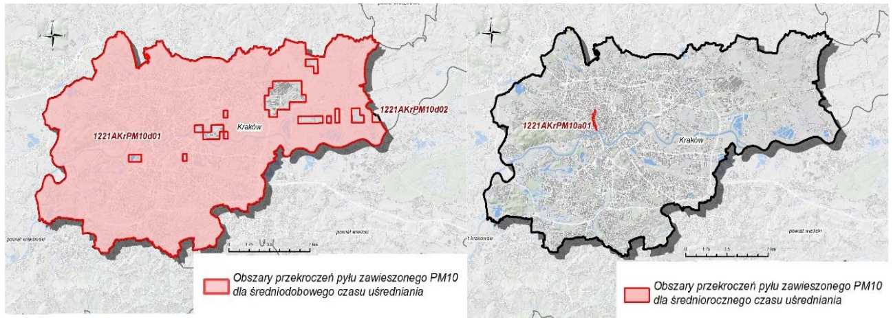
Rysunek 9. Obszary przekroczeń stężeń średniodobowych (po lewej) i średniorocznych (po prawej) pyłu PM10 w strefach Aglomeracja Krakowska zgodnie z Roczną oceną jakości powietrza w województwie małopolskim za 2021 r. 11
