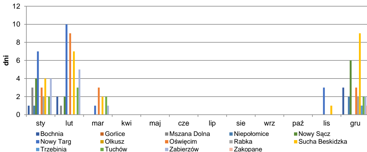
Rysunek 19. Liczba dni ze stężeniem średniodobowym pyłu PM10 powyżej poziomu informowania społeczeństwa (100 µg/m³) na stacjach pomiarowych PMS w strefie małopolskiej w 2021 roku. 63
