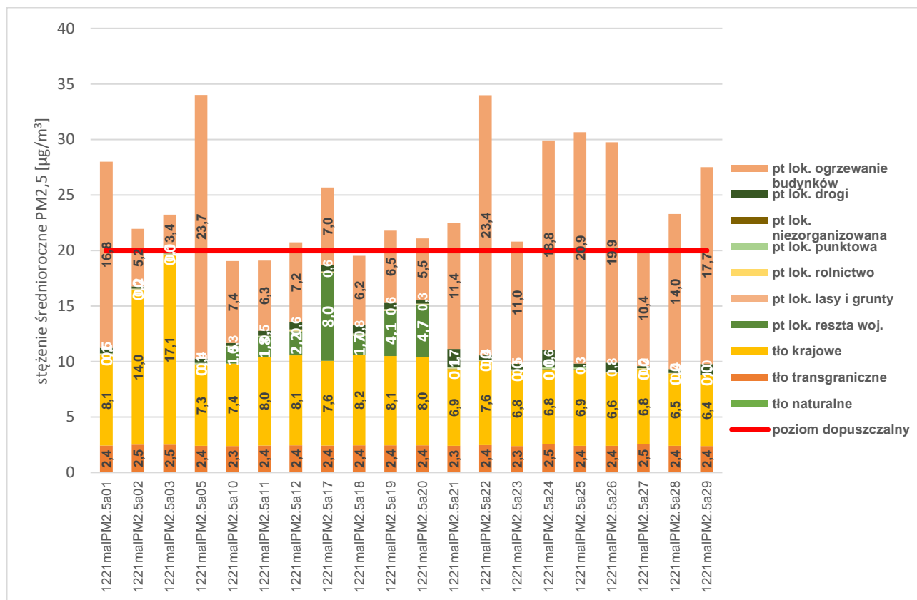
Rysunek 42. Prezentacja poziomów tła regionalnego, tła miejskiego oraz przyrostu tła lokalnego pyłu PM 2,5 w obszarze przekroczeń w strefie małopolskiej w 2021 roku 105 .
