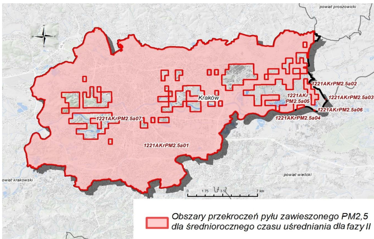
Rysunek 25. Obszary występowania przekroczeń stężeń średniorocznych pyłu PM 2,5 na obszarze Aglomeracji Krakowskiej na podstawie oceny jakości powietrza za rok 2021 dla województwa małopolskiego 71 .
