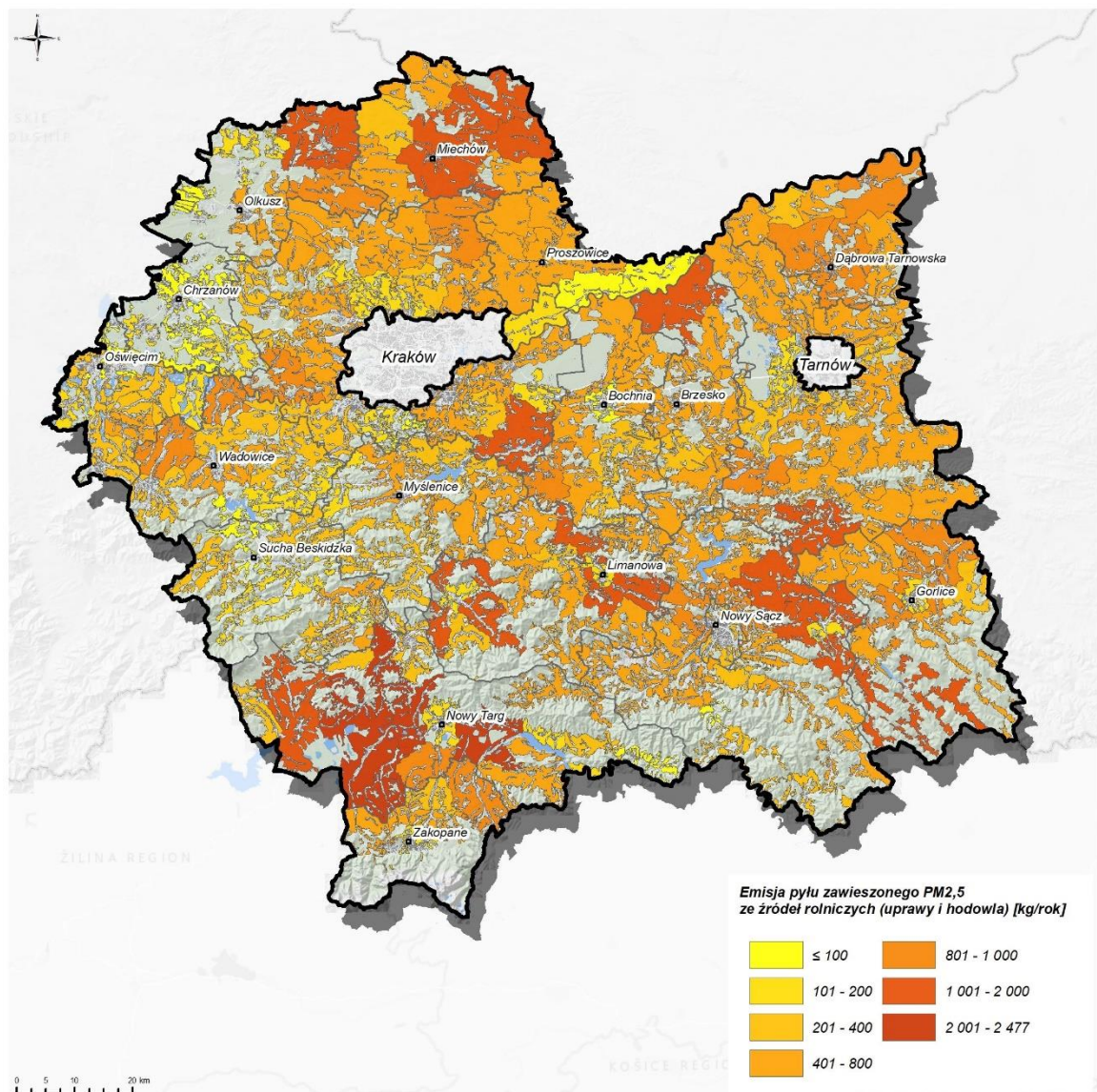
Rysunek 87. Emisja pyłu zawieszzonego PM 2,5 ze źródeł rolniczych (hodowla) w strefie małopolskiej w 2021 r.
