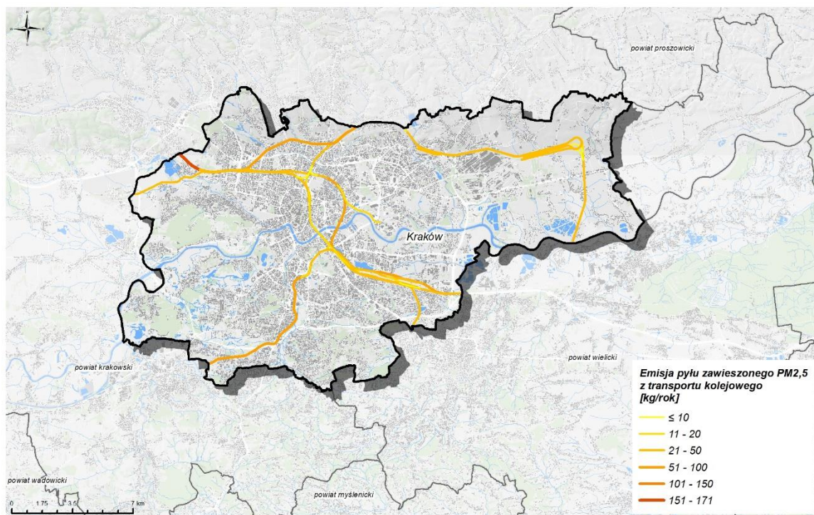
Rysunek 93. Emisja pyłu zawieszonego PM 2,5 z innych źródeł transportowych – kolej w strefie Aglomeracja Krakowska w 2021 r.
