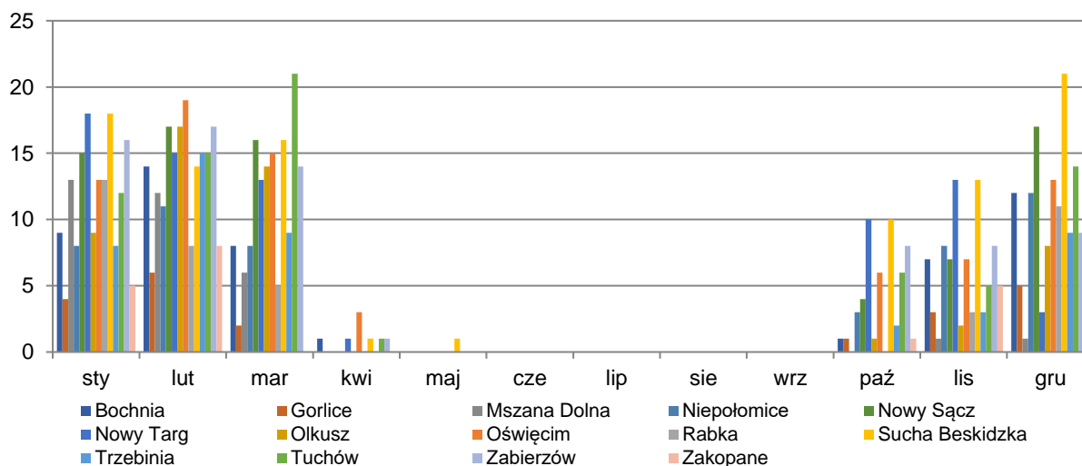
Rysunek 18. Liczba dni z przekroczeniem dopuszczalnego stężenia 24-godz. PM10 na stacjach pomiarowych PMS w strefie małopolskiej w 2021 roku 62
