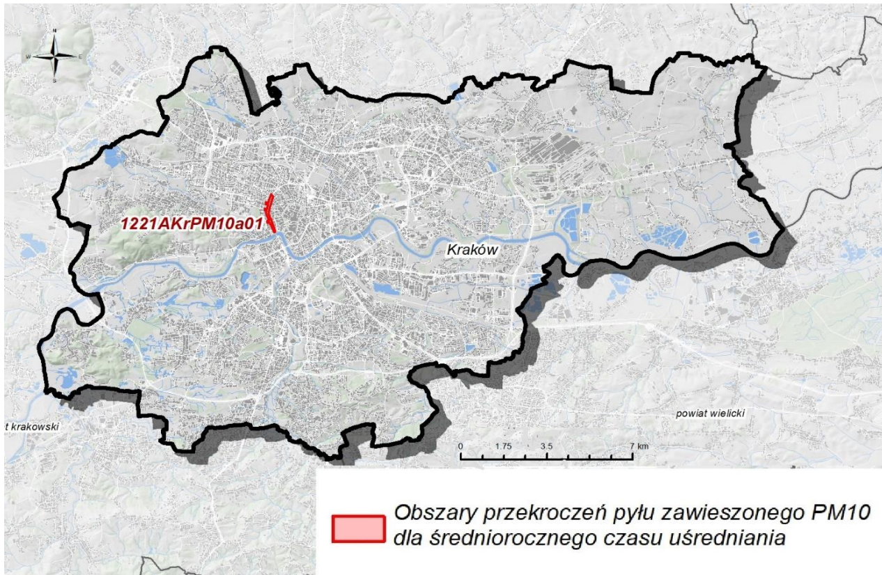
Rysunek 23. Obszary występowania przekroczeń stężeń średniorocznych pyłu PM10 na obszarze Aglomeracji Krakowskiej na podstawie oceny jakości powietrza za rok 2021 dla województwa małopolskiego 69 .
