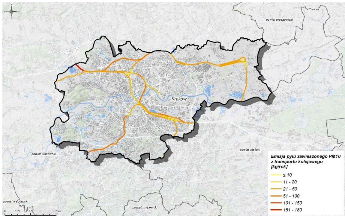
Rysunek 69. Emisja pyłu zawieszonego PM10 z innych źródeł (kolej) w strefie Aglomeracja Krakowska w 2021 r.
