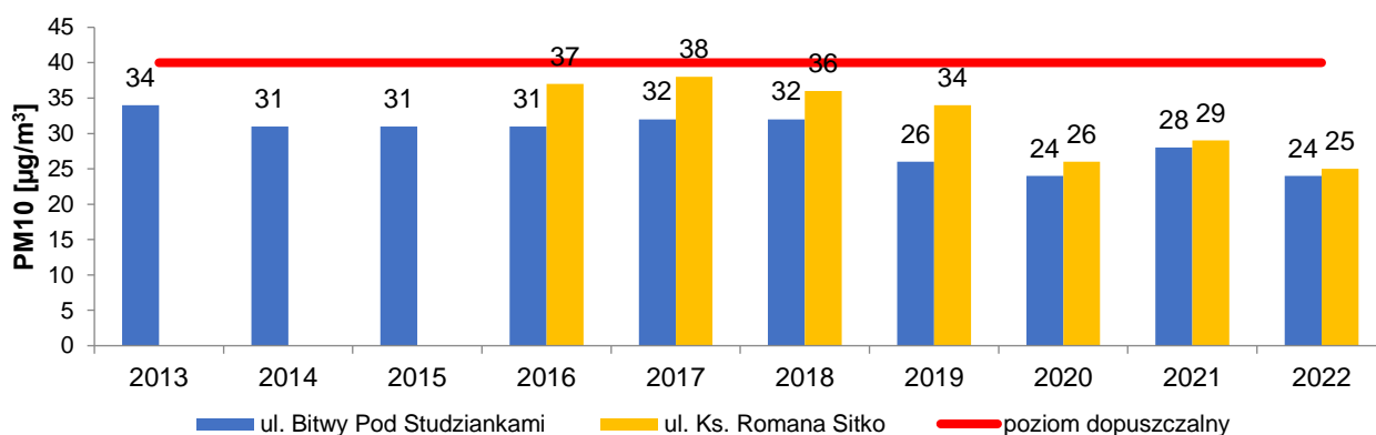
Rysunek 11. Stężenia średnioroczne pyłu PM10 na stacjach pomiarowych PMS w strefie miasto Tarnów w latach 2013-2022 54
