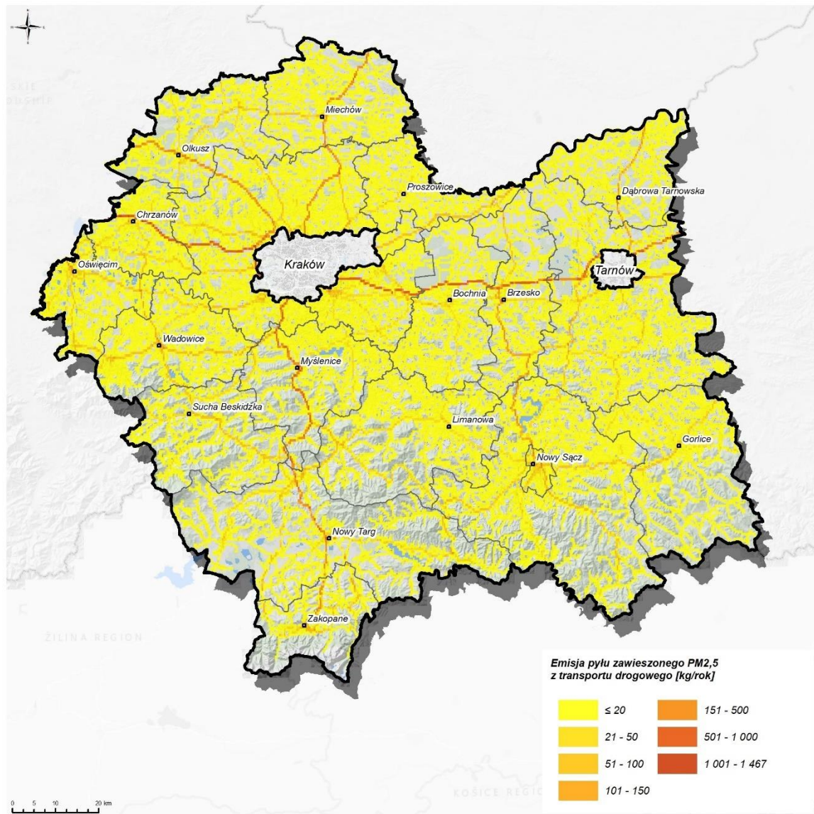
Rysunek 84. Emisja pyłu zawieszonego PM 2,5 z transportu drogowego w strefie małopolskiej w 2021 r.
