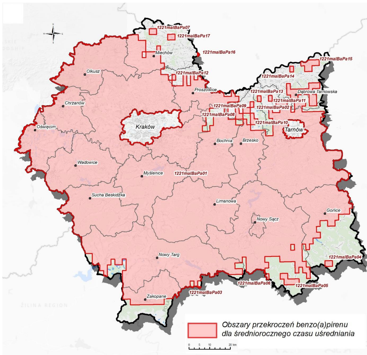
Rysunek 33. Obszary przekroczeń stężeń średniorocznych benzo(a)pirenu w strefie małopolskiej w 2021 roku. 84
