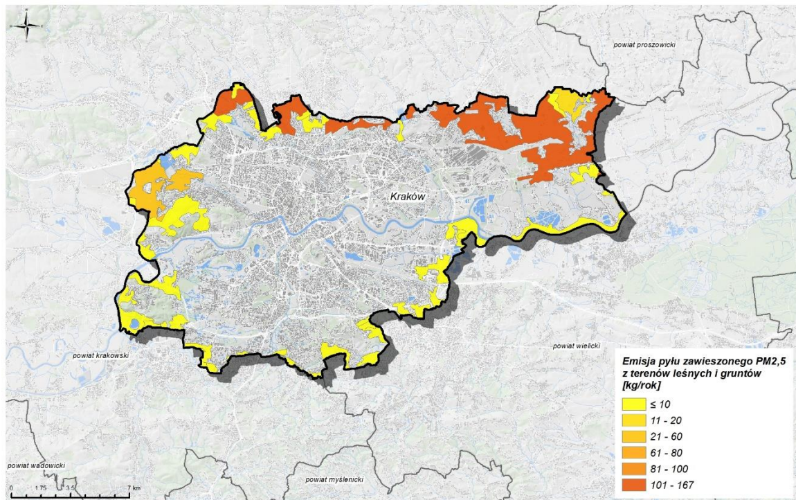
Rysunek 96. Emisja pyłu zawieszonego PM 2,5 ze źródeł rolniczych (uprawy, nawożenie, maszyny rolnicze) w strefie Aglomeracja Krakowska w 2021 r.
