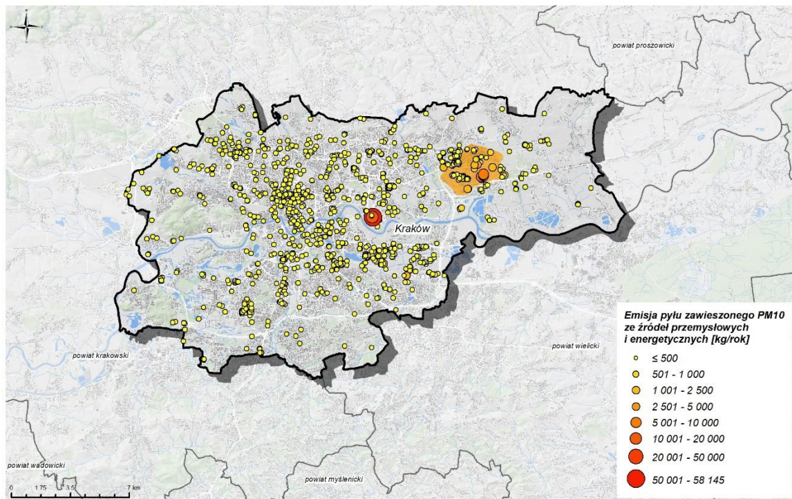
Rysunek 65. Emisja pyłu zawieszonego PM10 ze źródeł przemysłowych i energetycznych w strefie Aglomeracja Krakowska w 2021 r.
