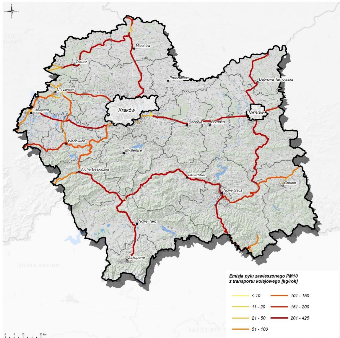
Rysunek 61. Emisja pyłu zawieszzonego PM10 z innych źródeł transportowych – kolej w strefie małopolskiej w 2021 r.
