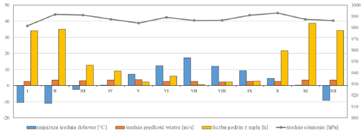
Rysunek 2. Miesięczny rozkład parametrów mogących sprzyjać powstawaniu epizodów wysokich stężeń w Krakowie w 2021 roku 27
