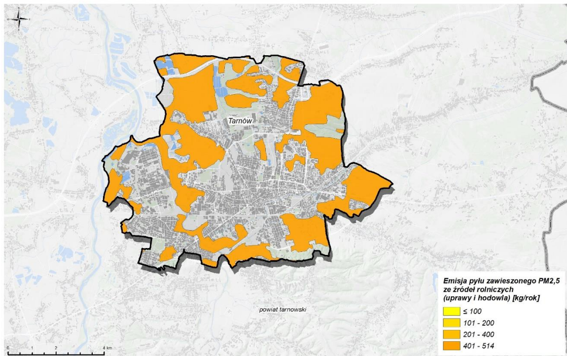
Rysunek 103. Emisja pyłu zawieszonoego PM 2,5 ze źródeł rolniczych (hodowla) w strefie miasto Tarnów w 2021 r.
