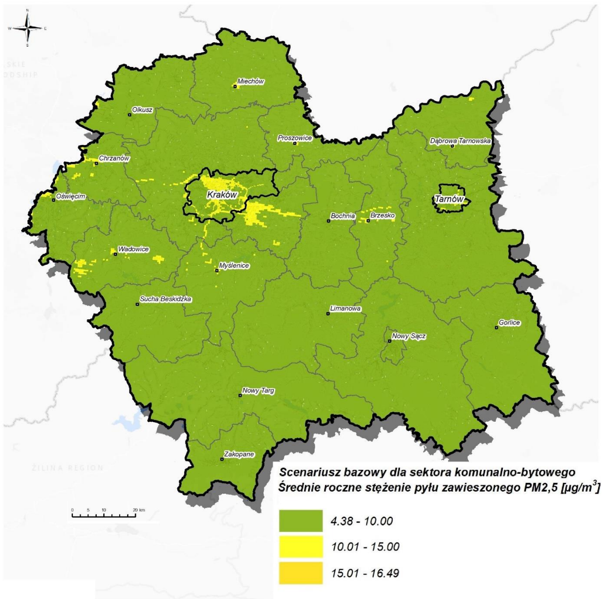
Rysunek 48. Rozkład stężeń średniorocznych pyłu PM 2,5 na obszarze województwa w roku prognozy 2026 w ramach scenariusza bazowego 138 .
