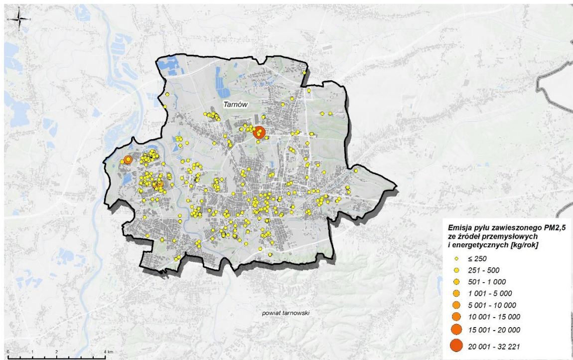
Rysunek 97. Emisja pyłu zawieszonego PM 2,5 ze źródeł przemysłowych i energetycznych w strefie miasto Tarnów w 2021 r.
