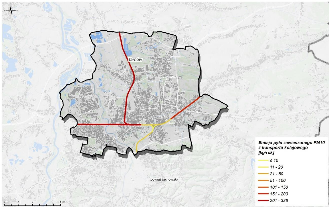
Rysunek 77. Emisja pyłu zawieszonego PM10 z innych źródeł (kolej) w strefie miasto Tarnów w 2021 r.
