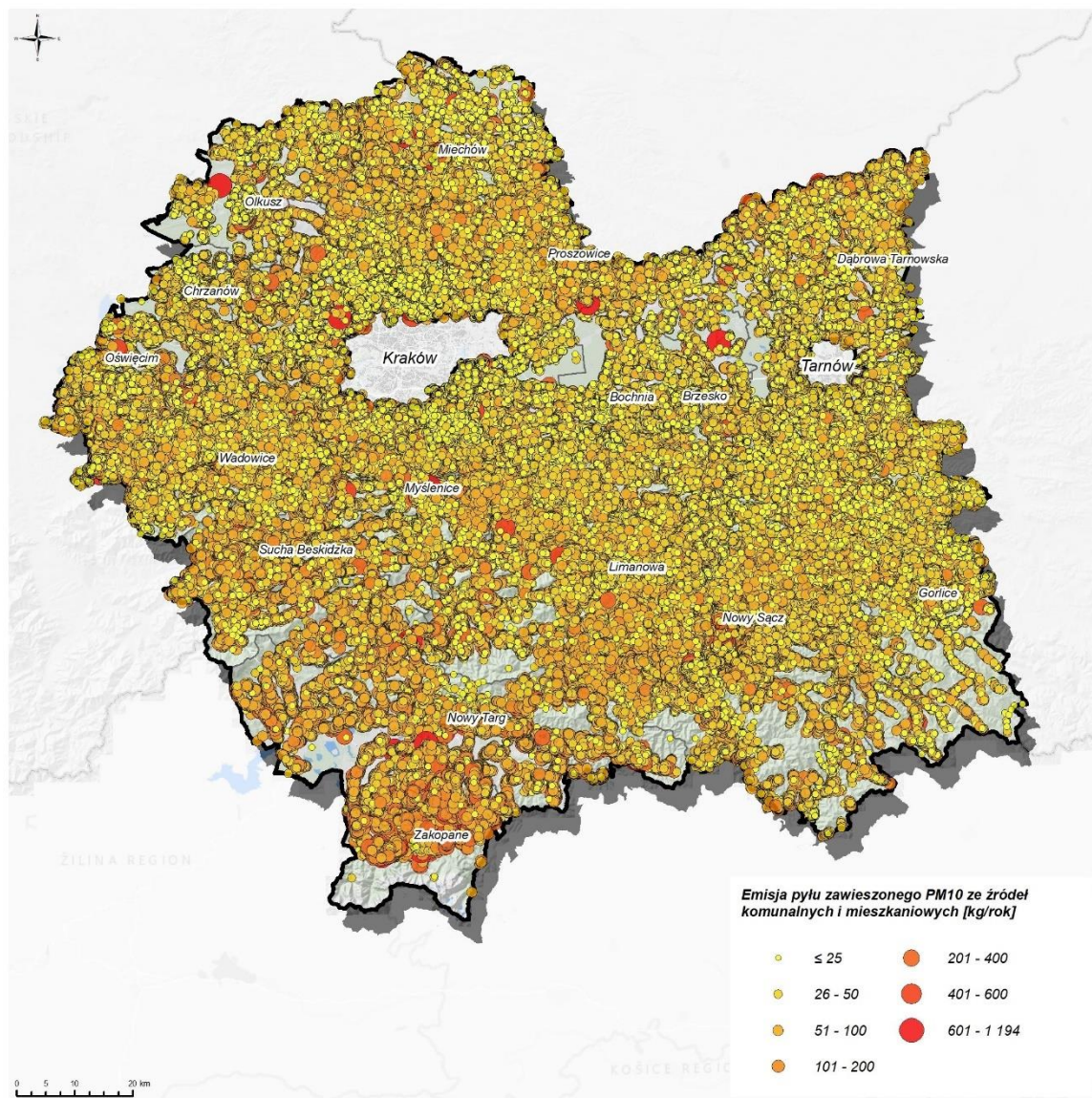
Rysunek 58. Emisja pyłu zawieszonego PM10 ze źródeł komunalno-bytowych w strefie małopolskiej w 2021 r.
