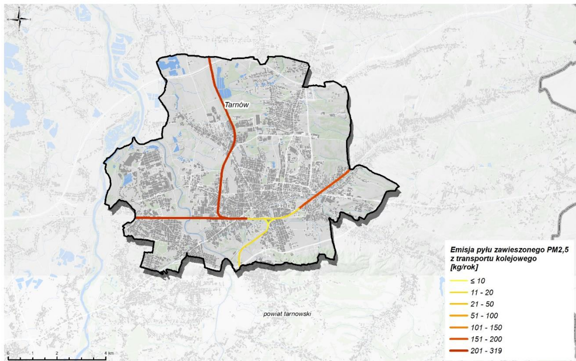
Rysunek 101. Emisja pyłu zawieszonoego PM2,5 z innych źródeł transportowych – kolej w strefie miasto Tarnów w 2021 r.
