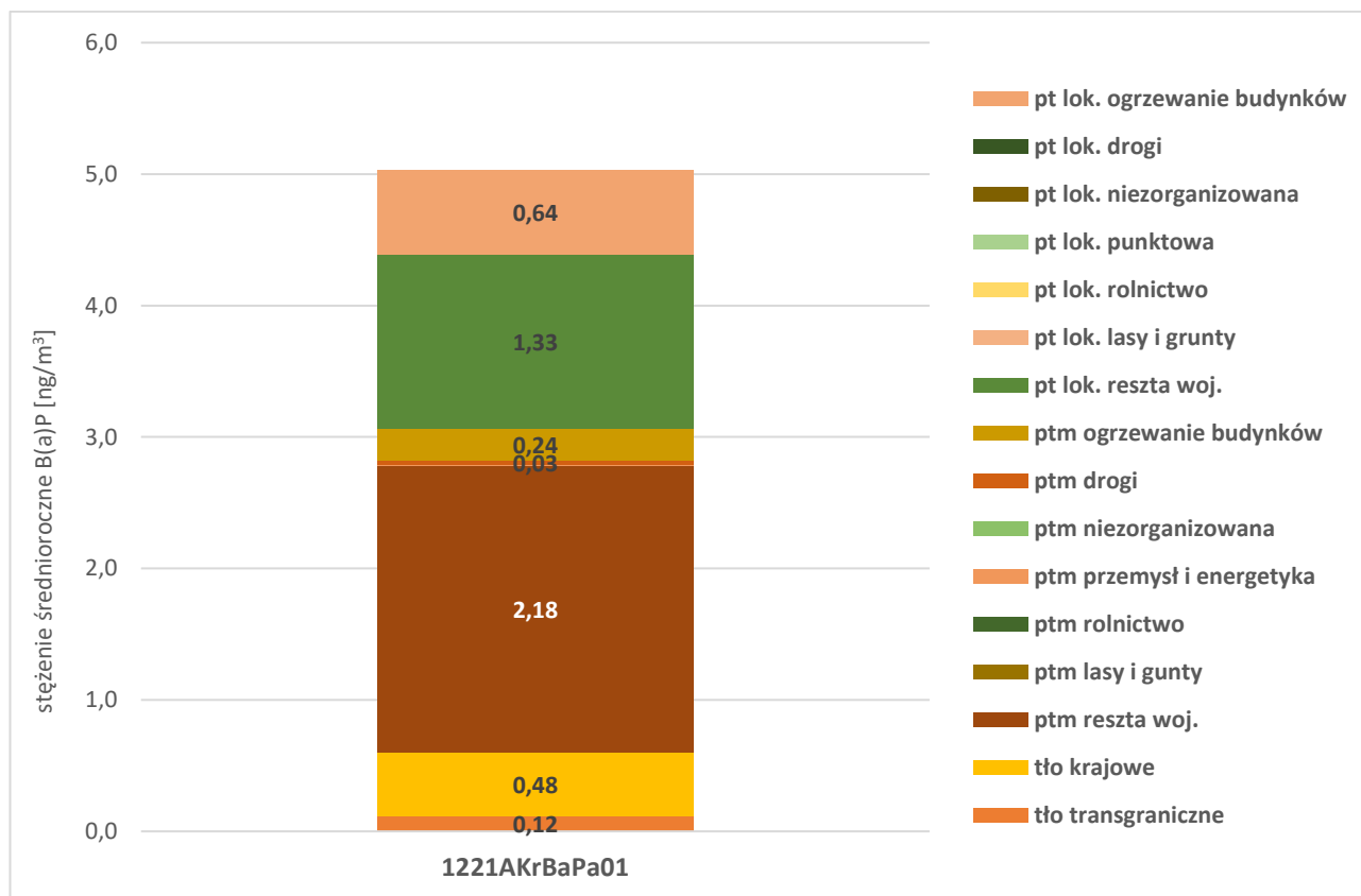
Rysunek 36. Prezentacja poziomów tła regionalnego, tła miejskiego oraz przyrostu tła lokalnego benzo(a)pirenu w obszarze przekroczeń w strefie Aglomeracja Krakowska w 2021 roku 93
