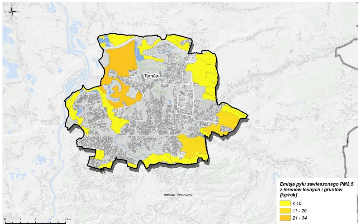
Rysunek 104. Emisja pyłu zawieszonoego PM 2,5 ze źródeł rolniczych (uprawy, nawożenie, maszyny rolnicze) w strefie miasto Tarnów w 2021 r.
