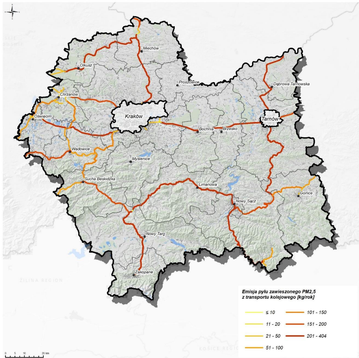
Rysunek 85. Emisja pyłu zawieszonego PM 2,5 z innych źródeł transportowych – kolej w strefie małopolskiej w 2021 r.
