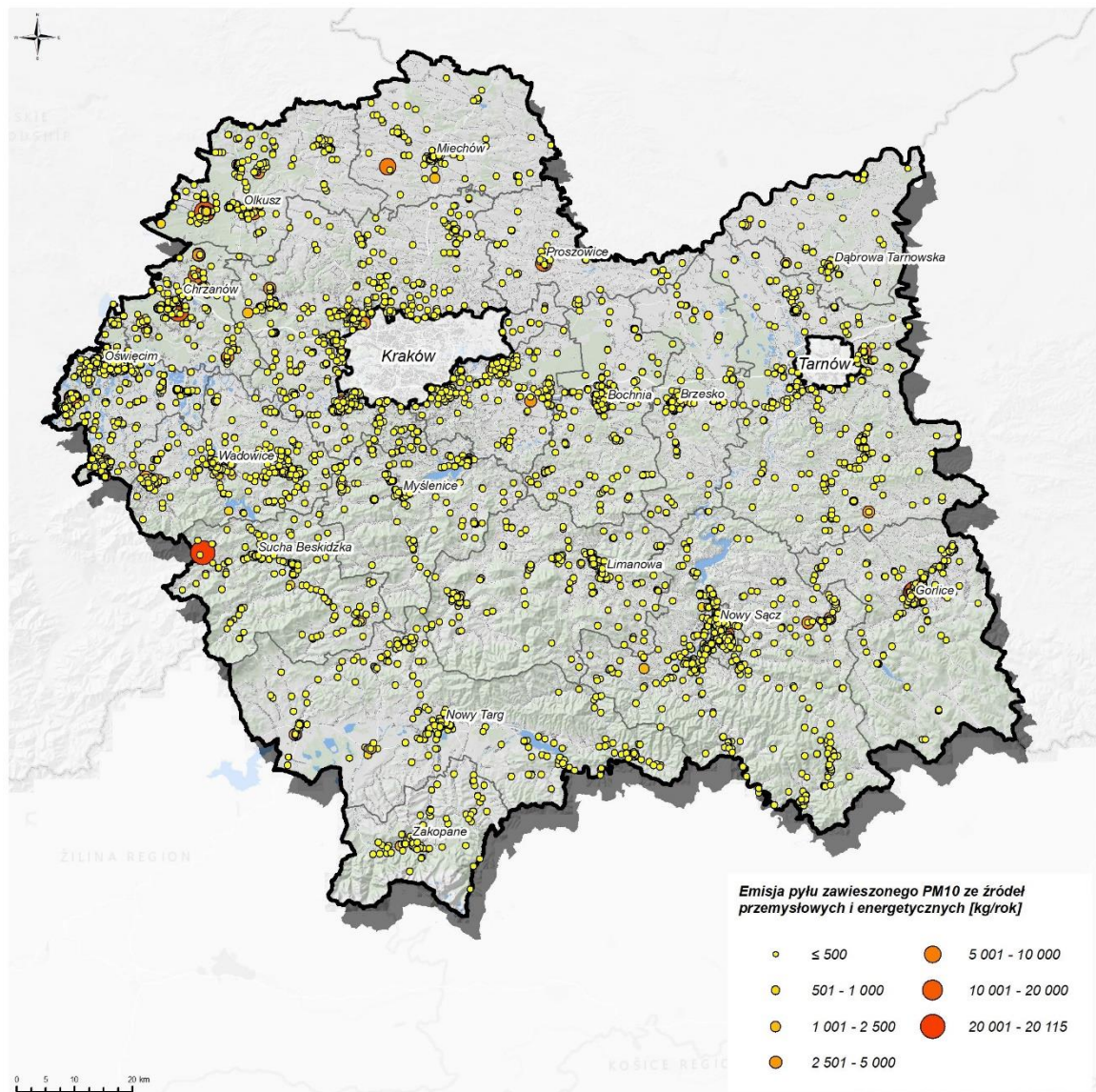
Rysunek 57. Emisja pyłu zawieszonego PM10 ze źródeł przemysłowych i energetycznych w strefie małopolskiej w 2021 r.
