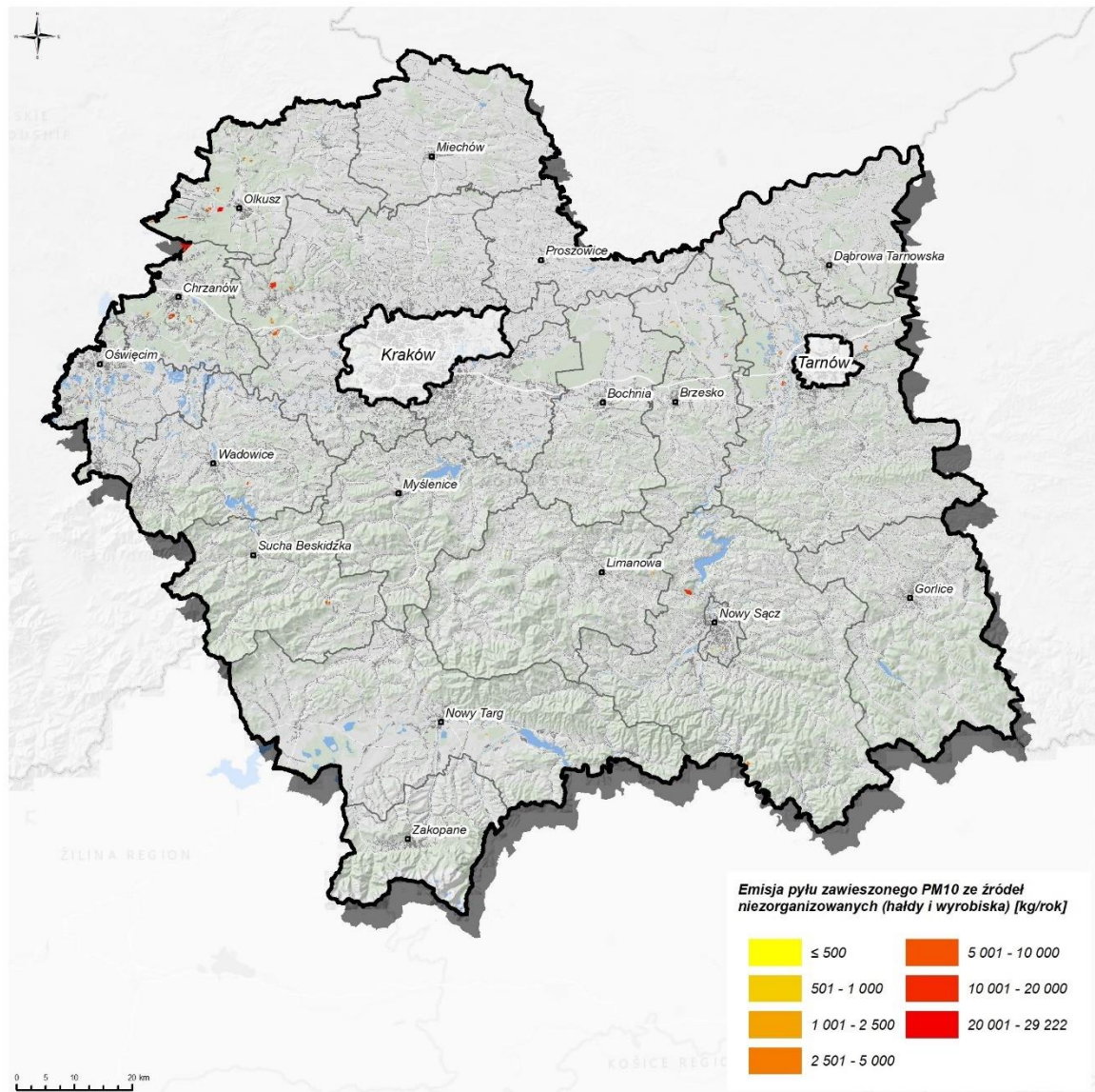
Rysunek 59. Emisja pyłu zawieszonego PM10 ze źródeł nieorganizowanych w strefie małopolskiej w 2021 r.
