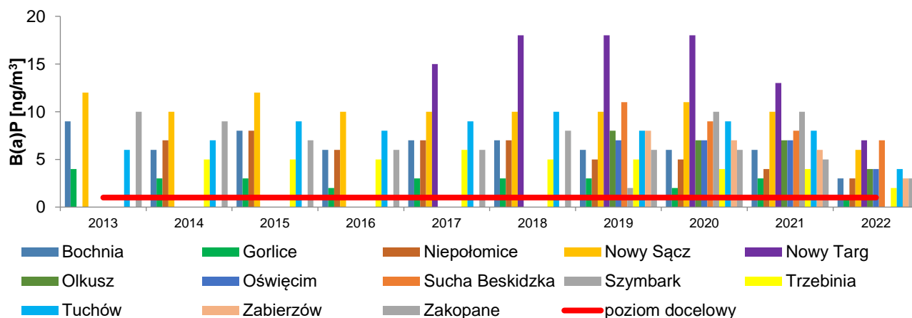
Rysunek 22. Stężenia średnioroczne benzo(a)pirenu na stacjach pomiarowych PMŚ w strefie małopolskiej w latach 2013-2022 67
