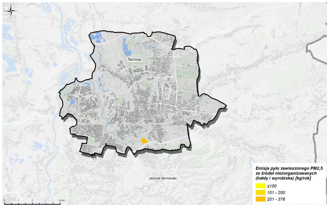
Rysunek 99. Emisja pyłu zawieszonoego PM 2,5 ze źródeł niezorganizowanych w strefie miasto Tarnów w 2021 r.
