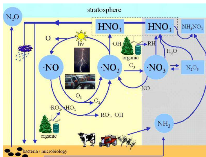
Rysunek 15. Procesy i wybrane reakcje chemiczne tlenków azotu w atmosferze 64
