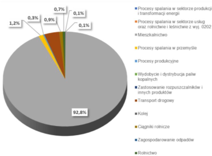
Rysunek 1-22 Udziały [%] poszczególnych rodzajów emisji z napływu na strefę miasto Rzeszów w łącznej emisji napływowej pyłu zawieszonego PM2,5 w 2021 r.
