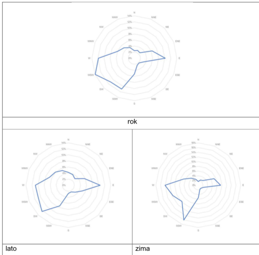
Rysunek 1-9 Róża wiatru ze stacji pomiarowej Rzeszów-Jasionka w strefie miasto Rzeszów w 2021 r.
