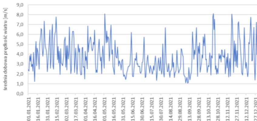
Rysunek 1-7 Przebieg średniej dobowej prędkości wiatru [m/s] dla strefy miasto Rzeszów w 2021 r.
