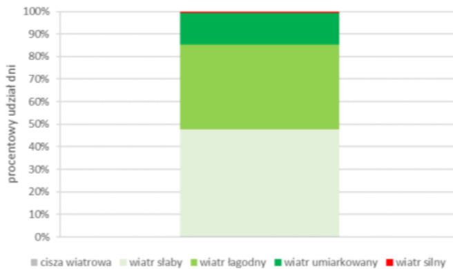
Rysunek 1-8 Procentowy udział dni z wiatrem słabym (1,1 - 3,3 m/s), łagodnym (3,4 - 5,4 m/s), umiarkowanym (5,5 - 7,9 m/s) i silnym (>8,0 m/s) oraz udział ciszy wiatrowych (<1,0 m/s) w strefie miasto Rzeszów w 2021 r.
