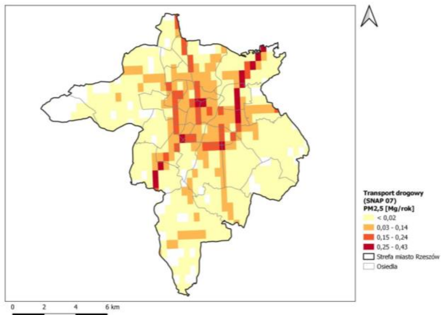
Rysunek 5-9 Rozmieszczenie oraz ładunki emisji pyłu zawieszonego PM 2,5 w sektorze transport drogowy (SNAP 07) w strefie miasto Rzeszów w 2021 r.
