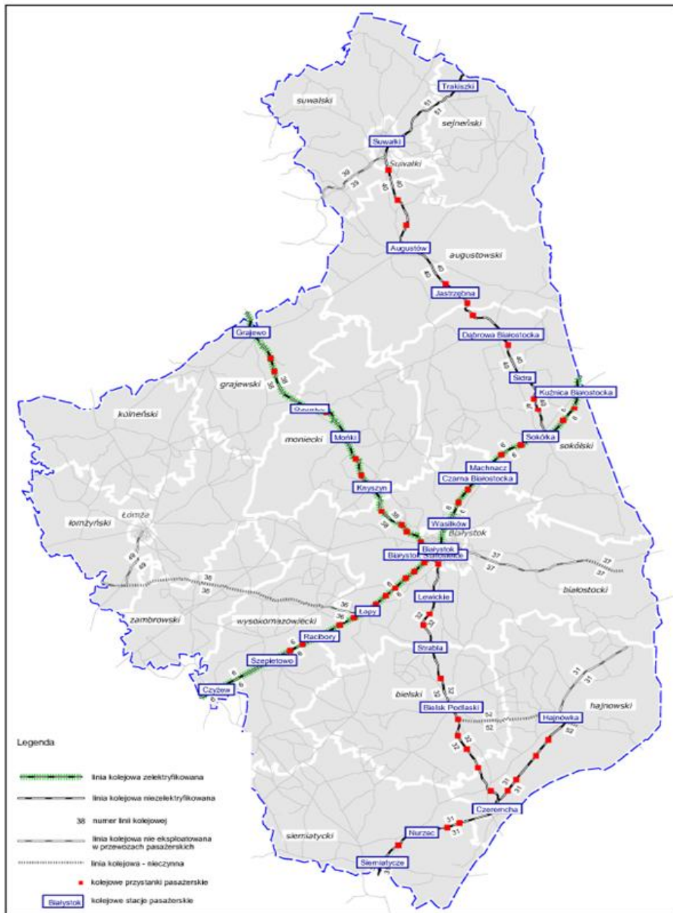
Rysunek 2.8.3.1 Schemat sieci kolejowej województwa podlaskiego.
