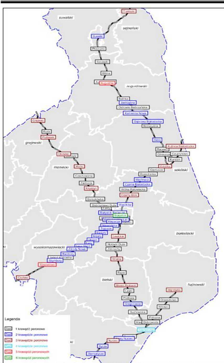
Rysunek 2.8.3.2.3 Standardy obsługi na przystankach i stacjach sieci kolejowej województwa podlaskiego - liczba krawędzi peronowych.
