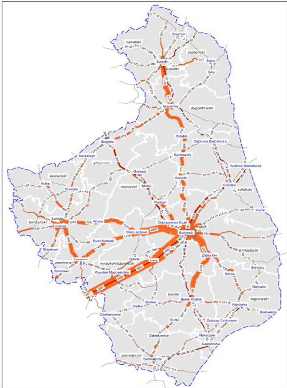
Rysunek 4.1.1 Rozkład potoków pasażerskich – stan istniejący 2013 r. [pasażerów/dobę].
