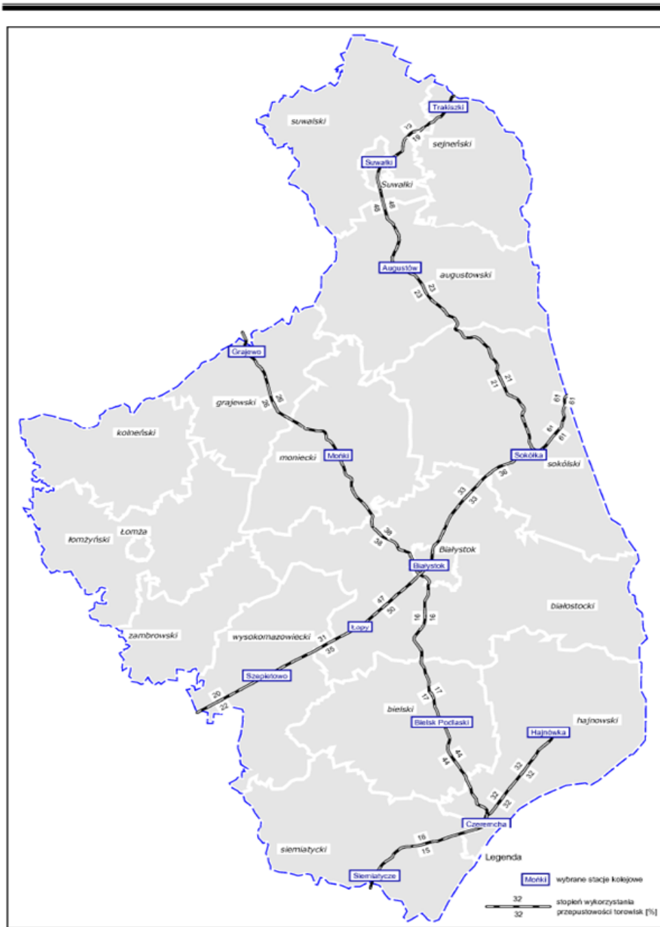
Rysunek 2.8.3.2.2 Stopień wykorzystania przepustowości sieci kolejowej województwa podlaskiego.
