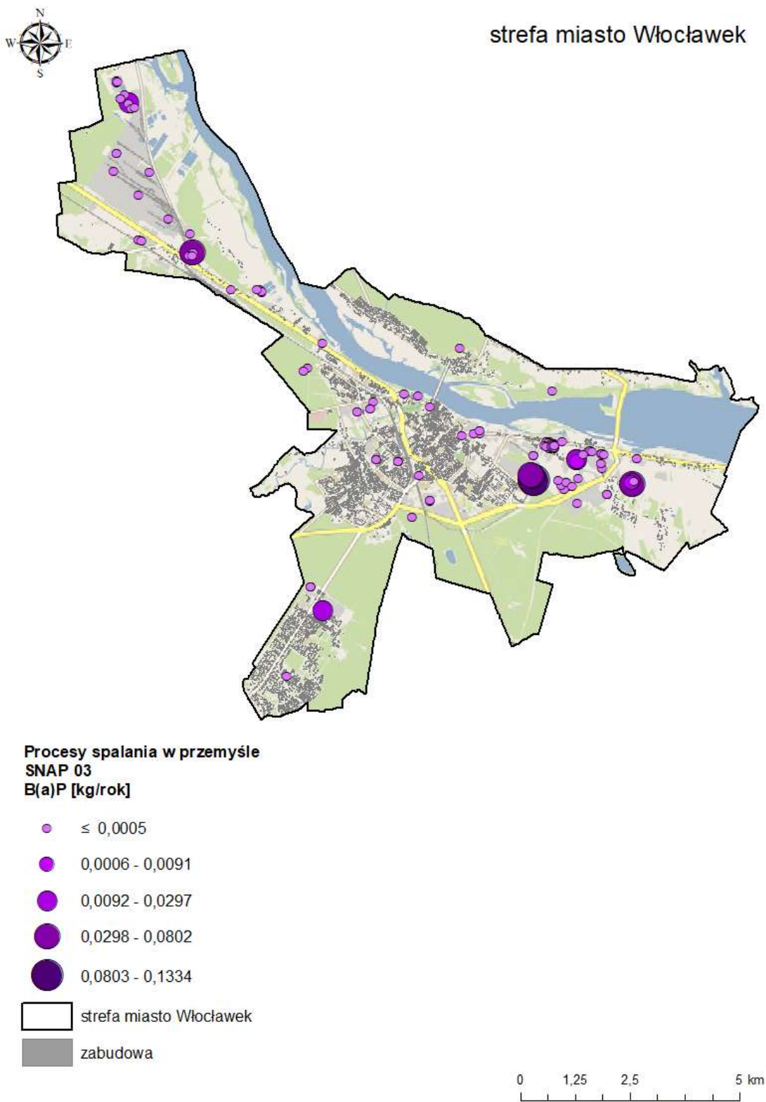
Rysunek 45. Emisja benzo(a)pirenu z procesów spalania w przemyśle (SNAP 03) 120
