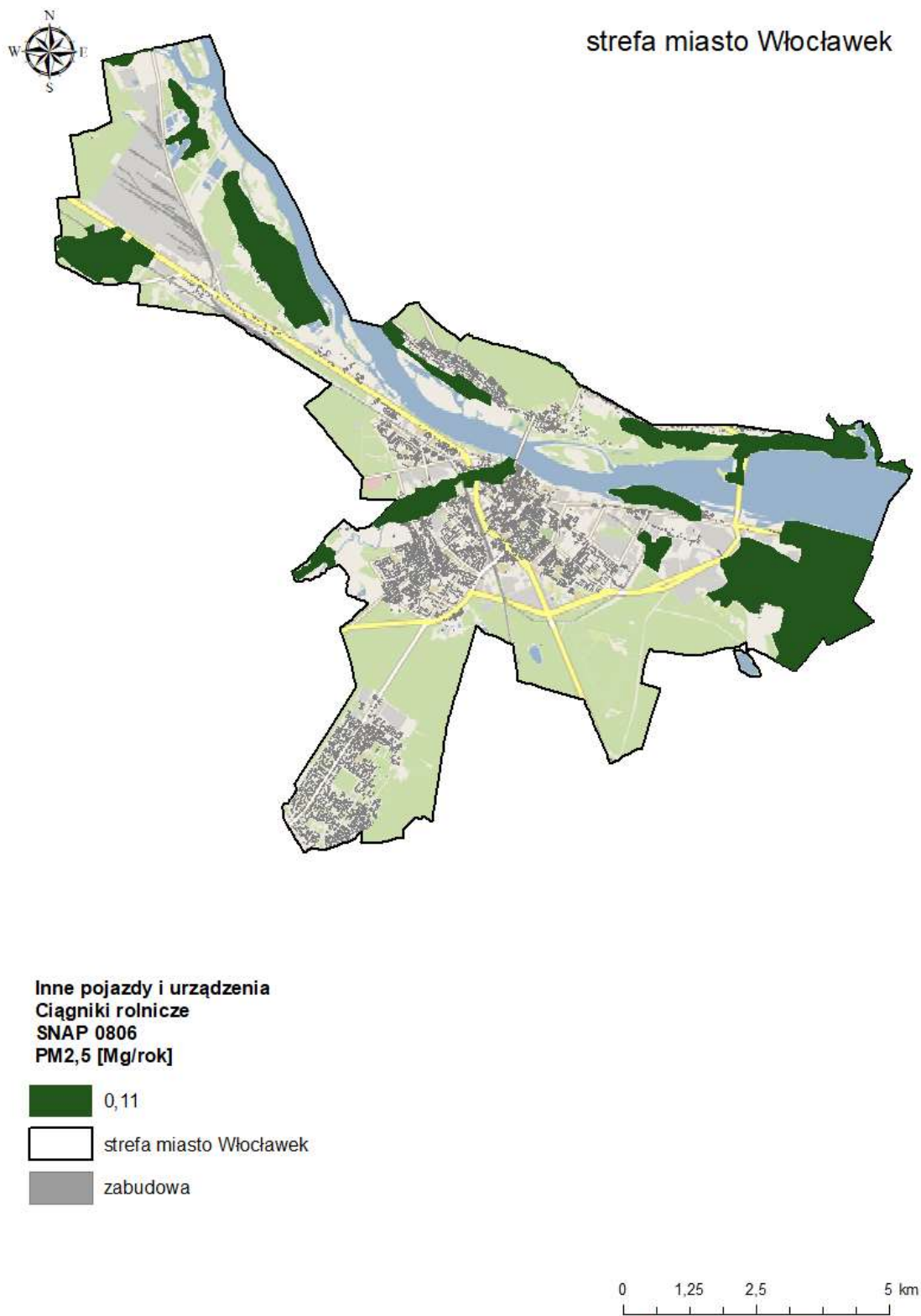
Rysunek 40. Emisja pyłu zawieszonego PM 2,5 z innych pojazdów i urządzeń - ciągników rolniczych (SNAP 0806) 115
