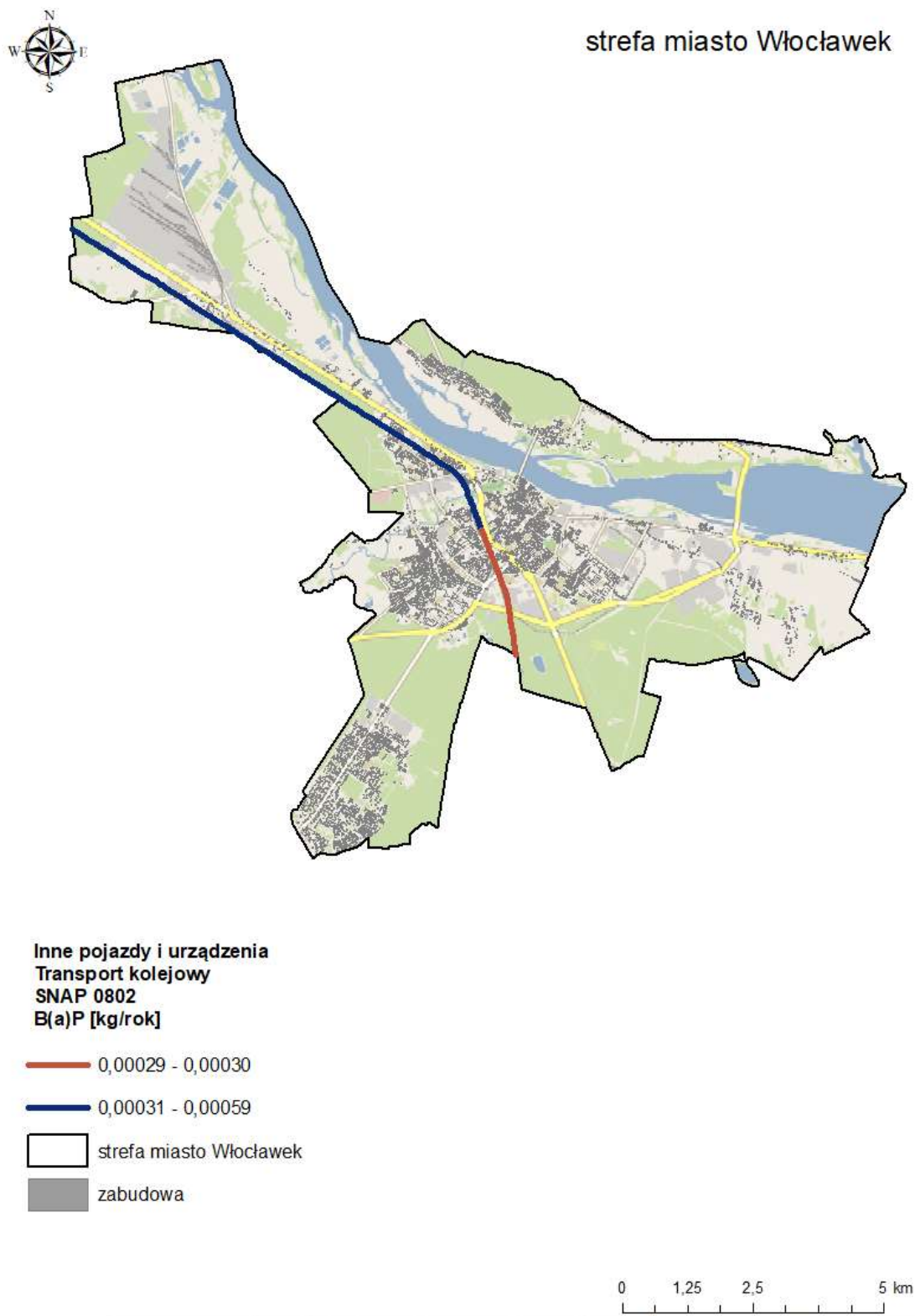
Rysunek 48. Emisja benzo(a)pirenu z innych pojazdów i urządzeń - transportu kolejowego (SNAP 0802) 123
