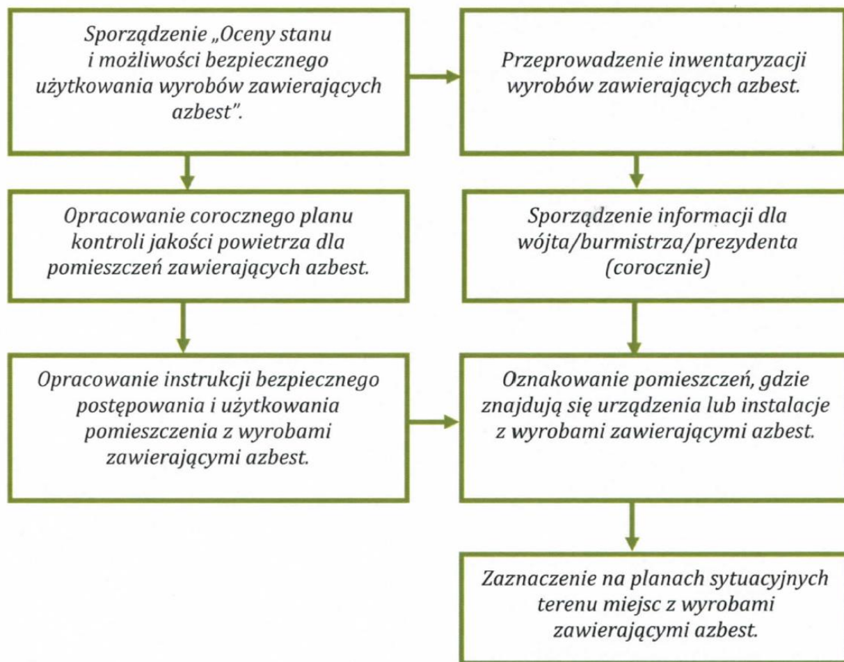
Rysunek 5. Procedura 1 - obowiązki i postępowanie właścicieli oraz zarządców, przy użytkowaniu obiektów i terenów z wyrobami zawierającymi azbest
