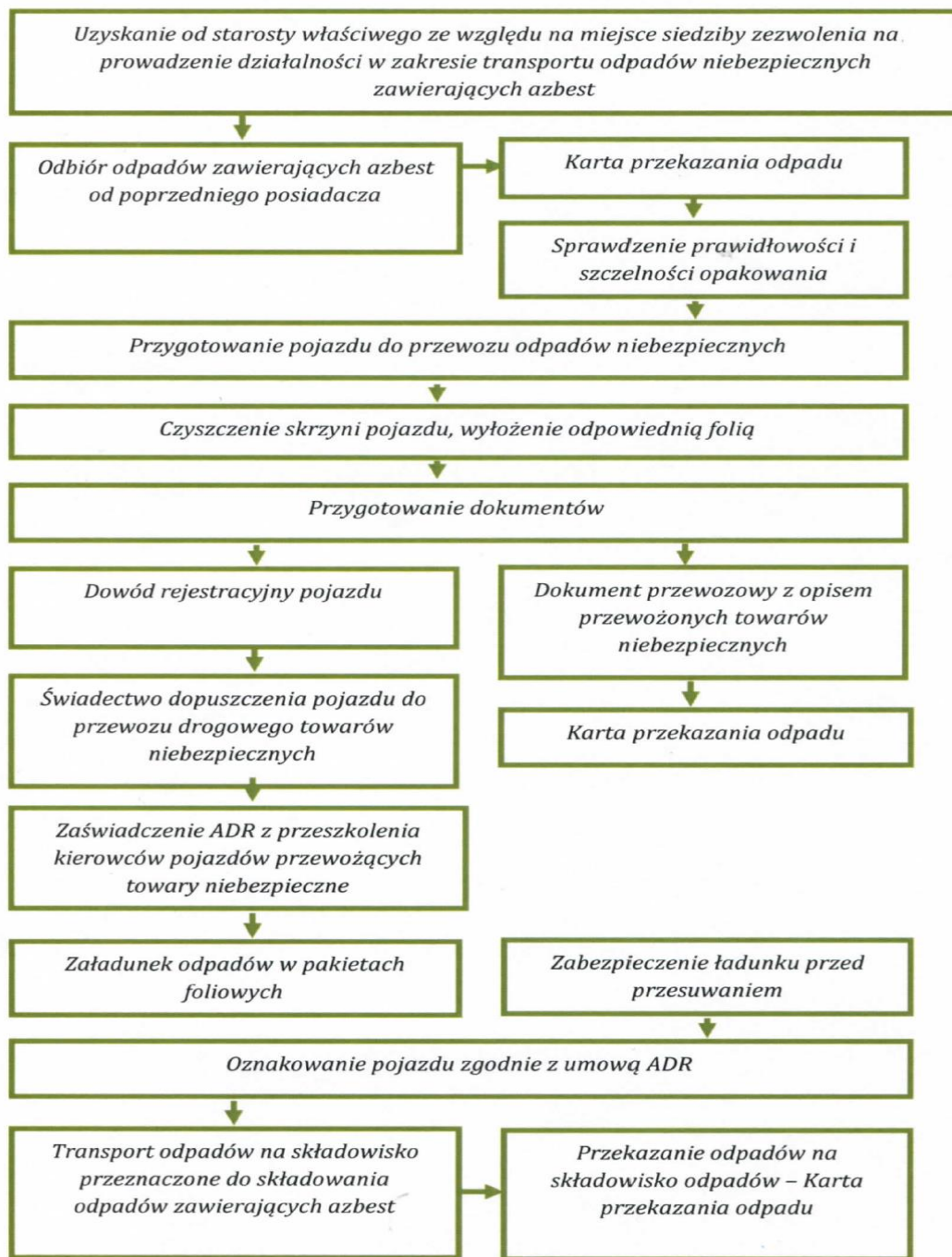
Rysunek 8. Procedura 5 - Przygotowanie i transport odpadów niebezpiecznych zawierających azbest
