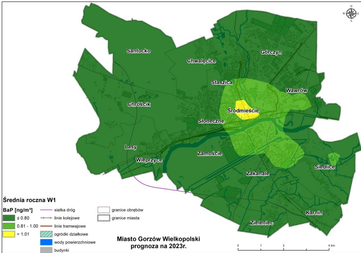
19. Rozkład przestrzenny stężeń średniorocznych benzo(a)pirenu w Gorzowie Wielkopolskim w roku prognozy 2023 52
