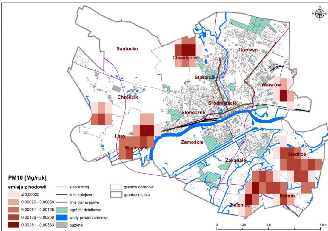
Rysunek 30. Lokalizacja źródeł emisji z hodowli zwierząt pyłu zawieszonego PM10 w Gorzowie Wielkopolskim w roku bazowym 2017 78
