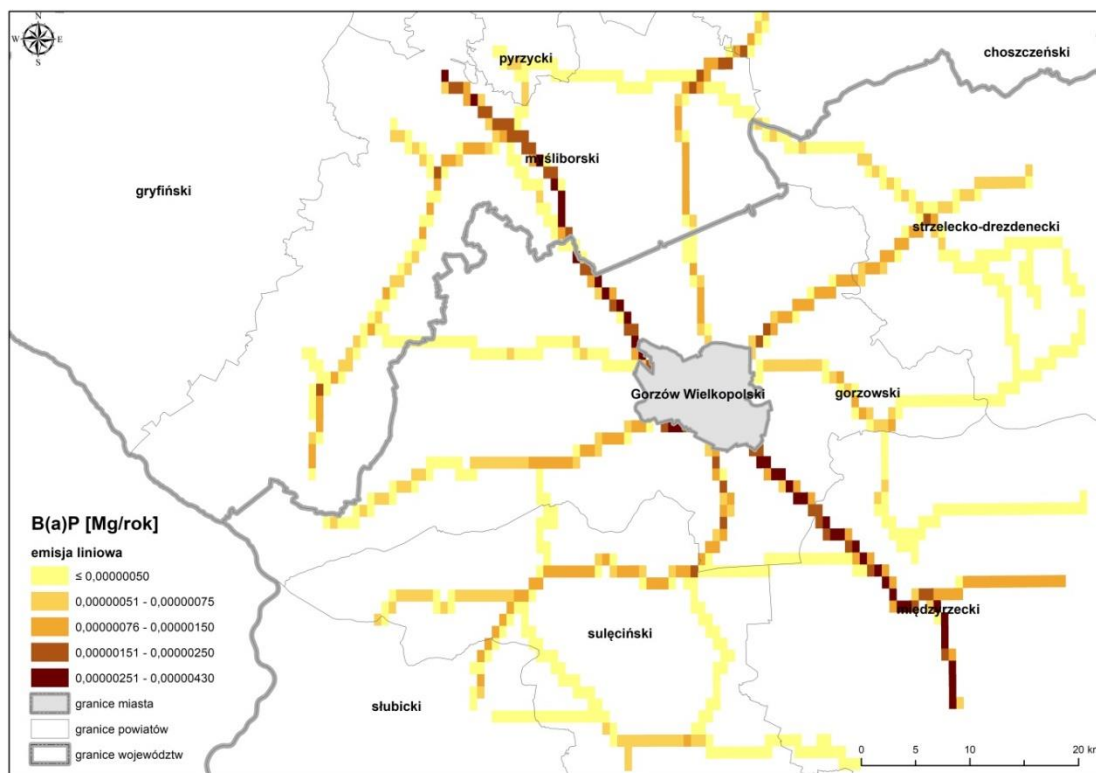
Rysunek 37. Lokalizacja źródeł emisji liniowych B(a)P na drogach krajowych i wojewódzkich z pasa 30 km wokół Gorzowa Wielkopolskiego w roku bazowym 2017 89
