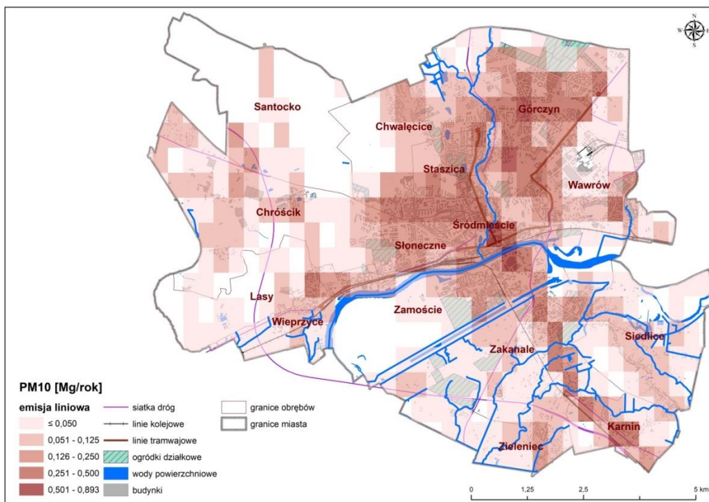
Rysunek 25. Lokalizacja źródeł emisji liniowej pyłu zawieszanego PM10 w Gorzowie Wielkopolskim na drogach powiatowych i gminnych w roku bazowym 2017 72
