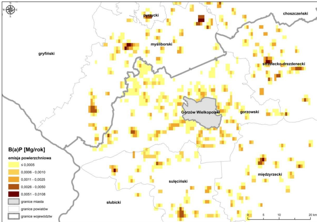
Rysunek 34. Lokalizacja źródeł emisji powierzchniowych B(a)P z pasa 30 km wokół Gorzowa Wielkopolskiego w roku bazowym 2017 86
