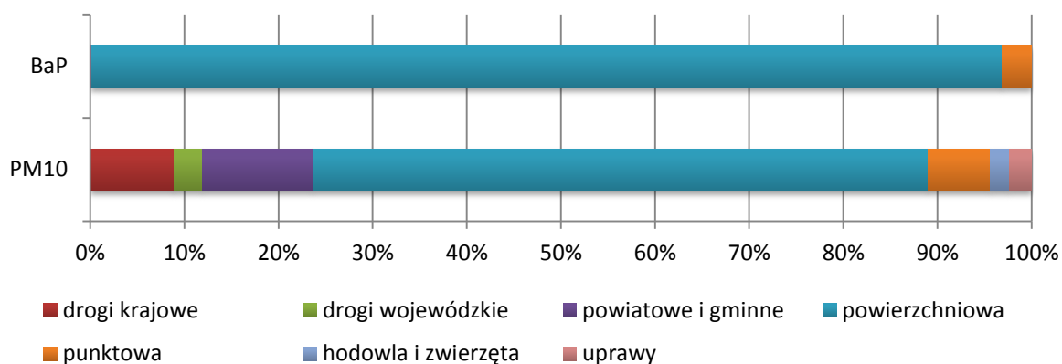
Rysunek 10. Procentowe udziały poszczególnych rodzajów emisji w rocznej emisji pyłu zawieszonego PM10 i benzo(a)pirenu w 2017 roku w Gorzowie Wielkopolskim 30
