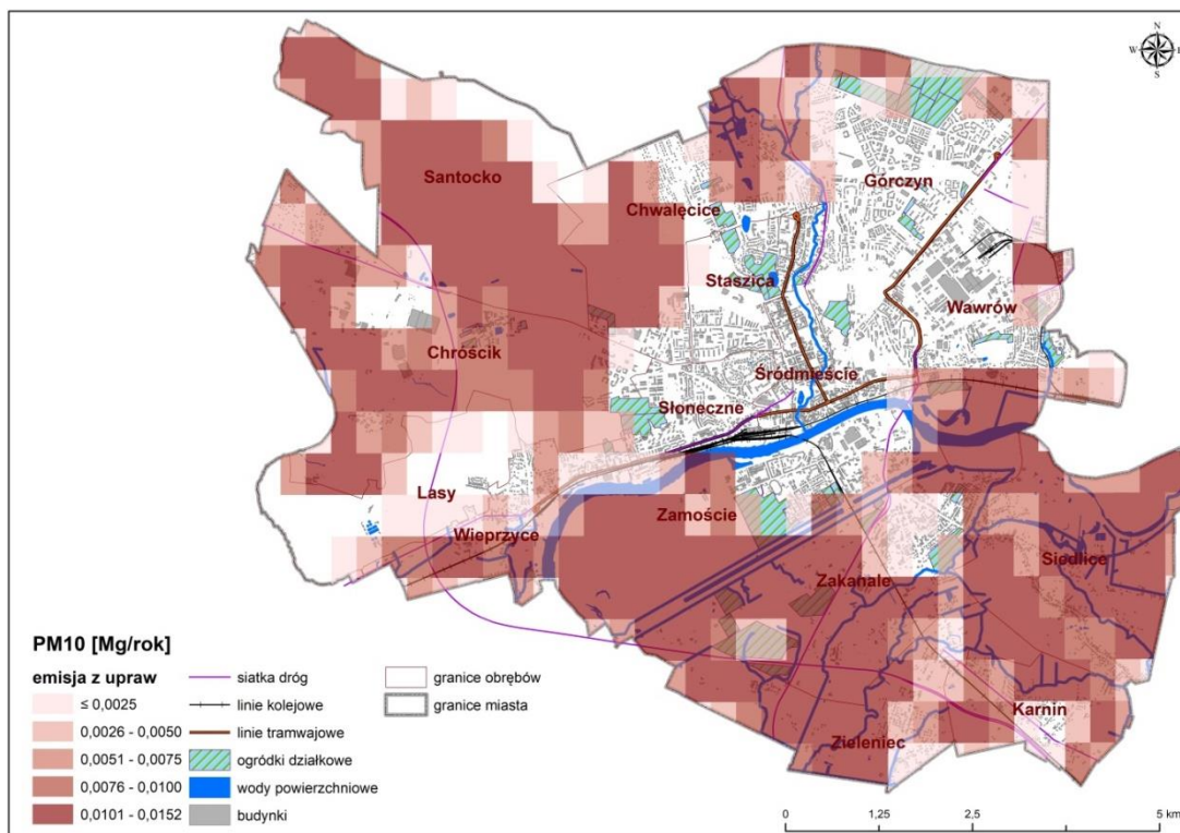
Rysunek 28. Lokalizacja źródeł emisji z upraw pyłu zawieszonego PM10 w Gorzowie Wielkopolskim w roku bazowym 2017 76
