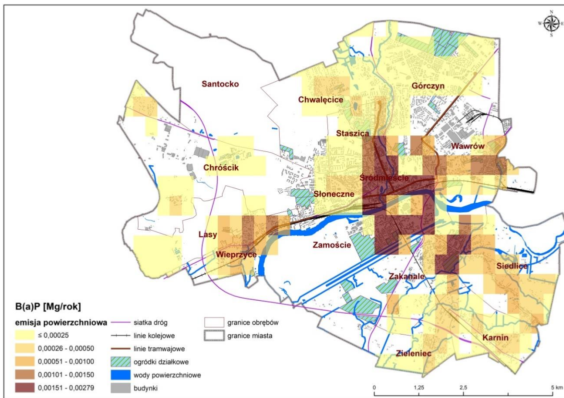
Rysunek 23. Lokalizacja źródeł emisji powierzchniowej B(a)P w Gorzowie Wielkopolskim w roku bazowym 2017 69
