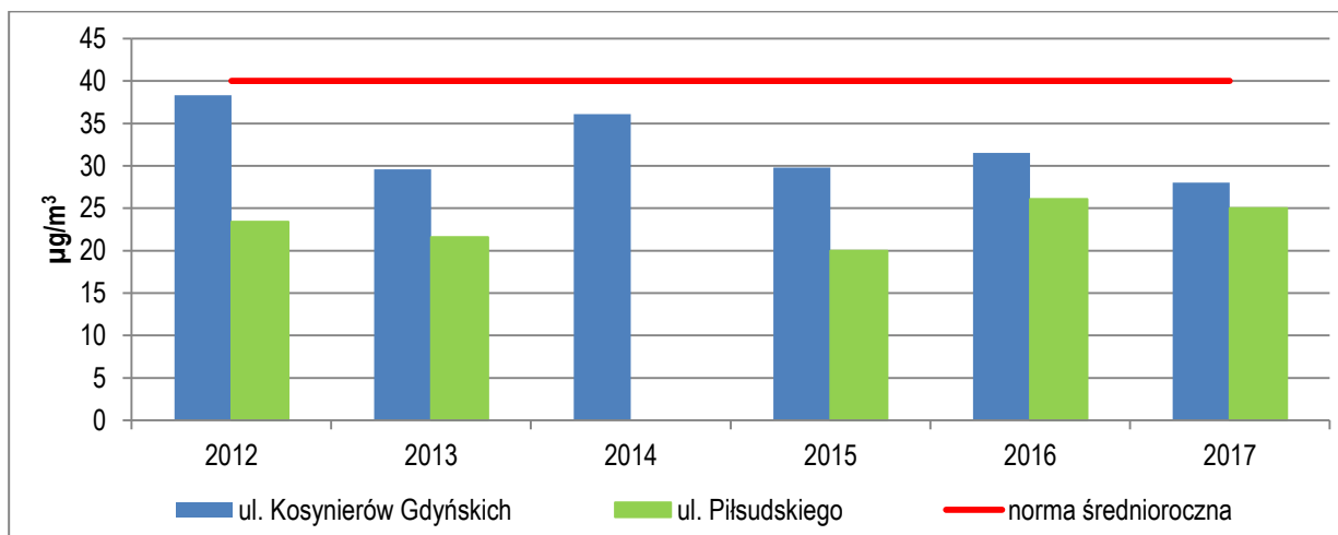
Rysunek 5. Wartości stężeń średniorocznych pyłu zawieszonego PM10 zmierzonych na stacjach w Gorzowie Wielkopolskim w latach 2012-2017
