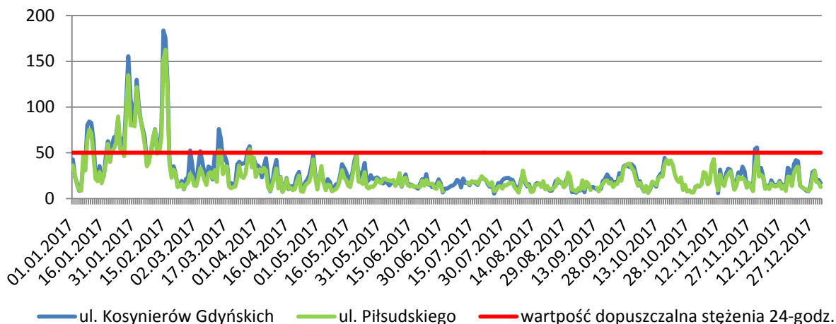
Rysunek 7. Rozkład stężeń 24-godzinnych pyłu zawieszonego PM10 zmierzonych na stacjach w Gorzowie Wielkopolskim w 2017 roku
