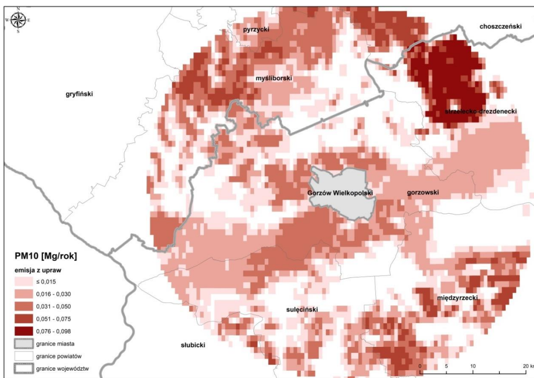
Rysunek 39. Lokalizacja źródeł emisji z upraw pyłu zawieszonego PM10 z pasa 30 km wokół Gorzowa Wielkopolskiego w roku bazowym 2017 91
