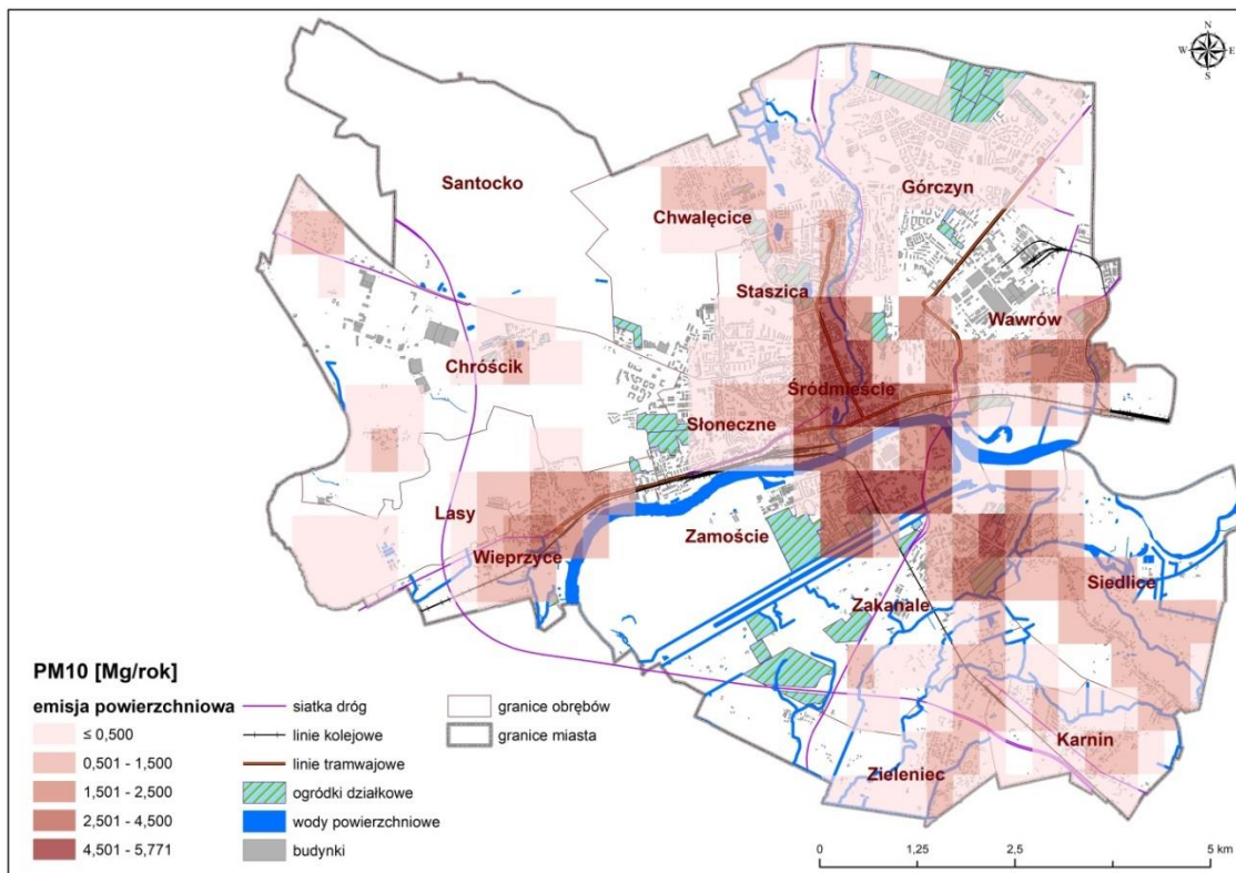
Rysunek 22. Lokalizacja źródeł emisji powierzchniowej pyłu zawieszonego PM10 w Gorzowie Wielkopolskim w roku bazowym 2017 68
