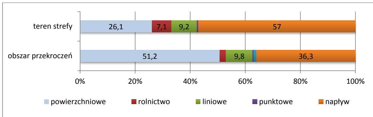
Rysunek 14. Udział emisji poszczególnych źródeł w stężeniach 24-godzinnych pyłu zawieszonego PM10 w Gorzowie Wielkopolskim w 2017 roku 37
