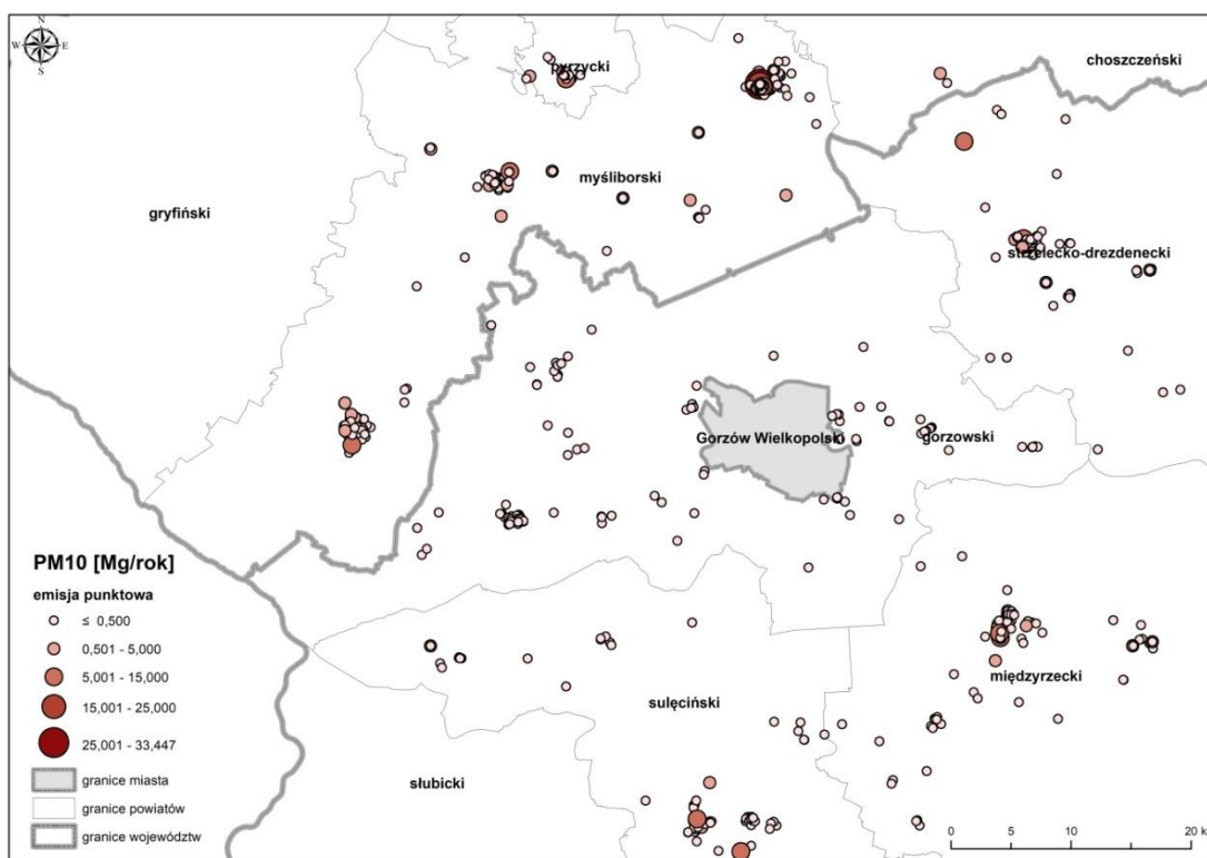
Rysunek 31. Lokalizacja źródeł emisji punktowych pyłu zawieszonego PM10 z pasa 30 km wokół Gorzowa Wielkopolskiego w roku bazowym 2017 83
