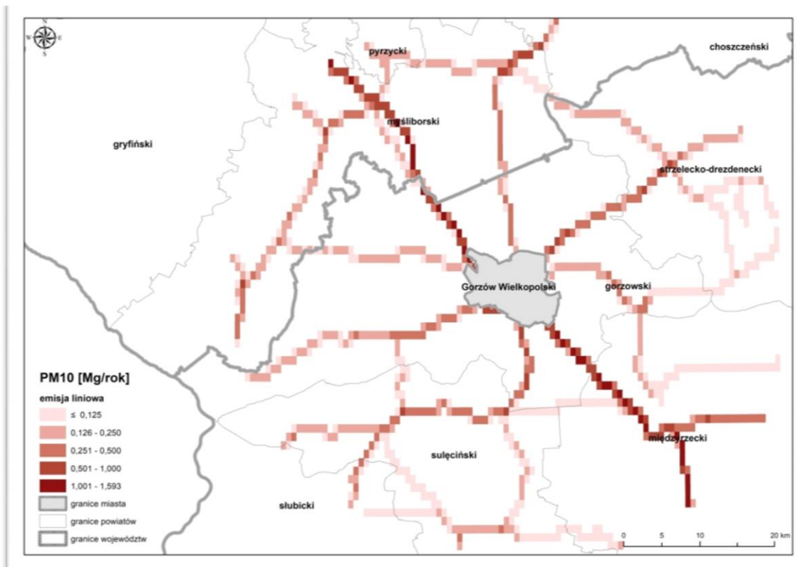
Rysunek 35. Lokalizacja źródeł emisji liniowych pyłu zawieszanego PM10 na drogach krajowych i wojewódzkich z pasa 30 km wokół Gorzowa Wielkopolskiego w roku bazowym 2017 87
