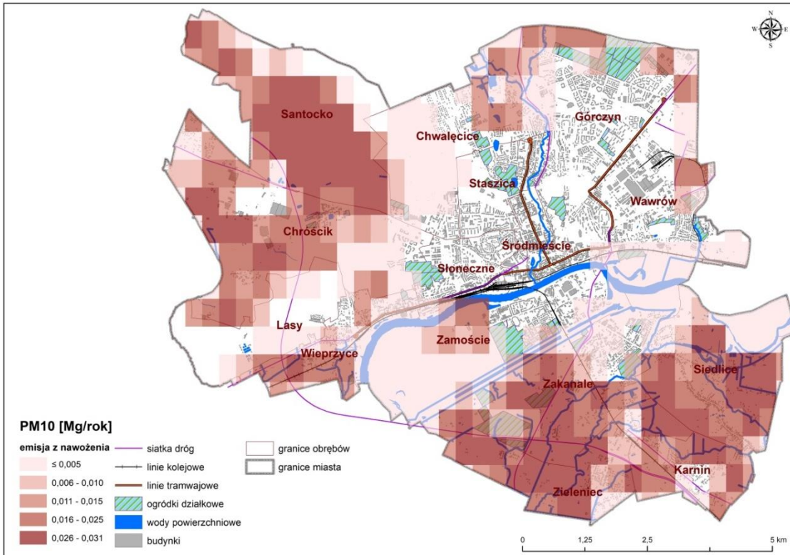
Rysunek 29. Lokalizacja źródeł emisji z nawożenia pyłu zawieszonego PM10 w Gorzowie Wielkopolskim w roku bazowym 2017 77
