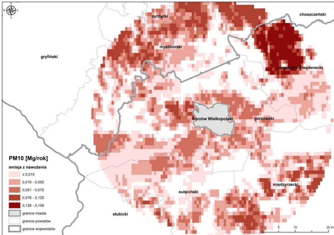
Rysunek 40. Lokalizacja źródeł emisji z nawożenia pyłu zawieszonego PM10 z pasa 30 km wokół Gorzowa Wielkopolskiego w roku bazowym 2017 92
