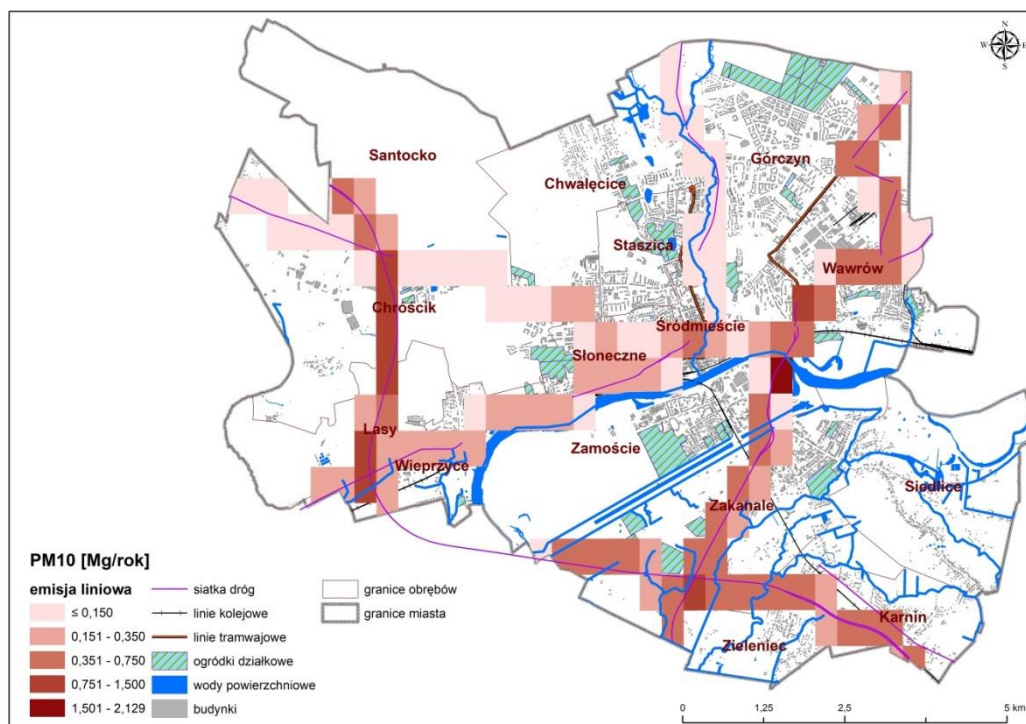
Rysunek 24. Lokalizacja źródeł emisji liniowej pyłu zawieszonego PM10 w Gorzowie Wielkopolskim na drogach krajowych i wojewódzkich w roku bazowym 2017 71
