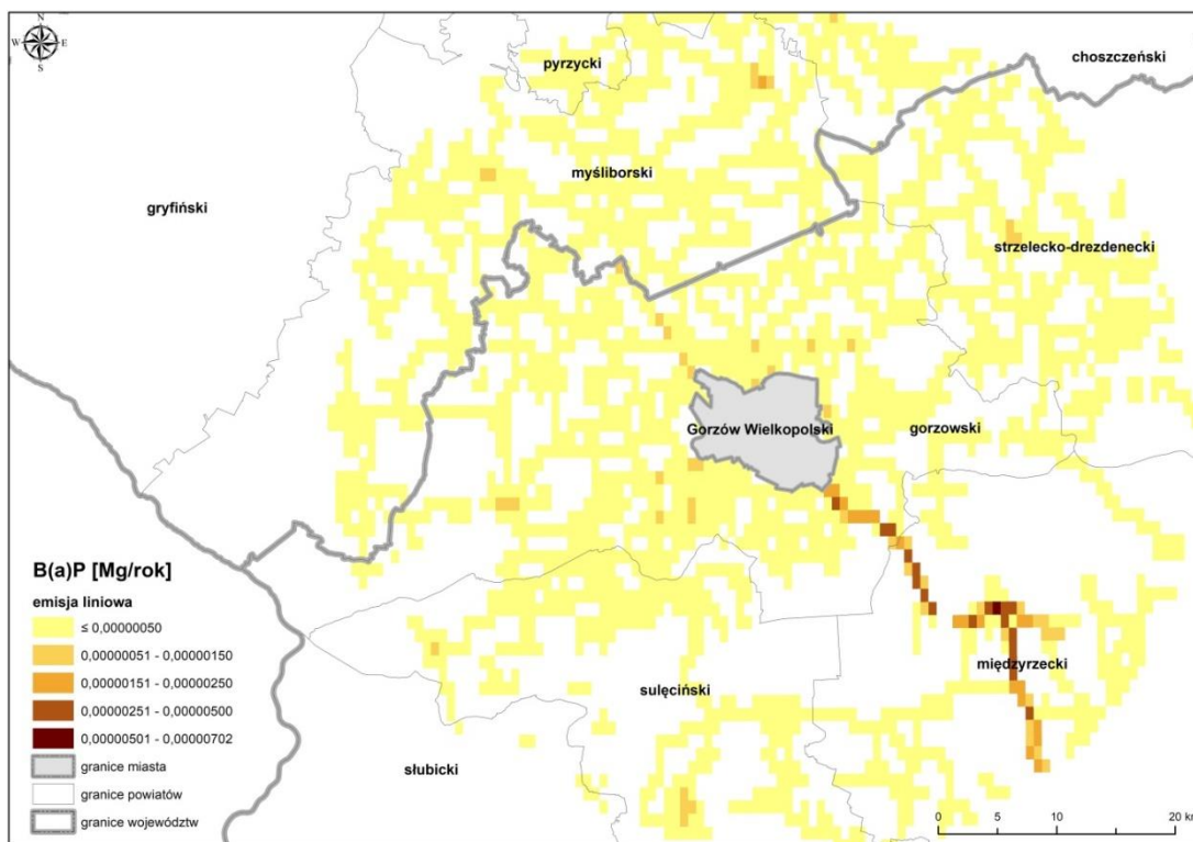
Rysunek 38. Lokalizacja źródeł emisji liniowych B(a)P na drogach powiatowych i gminnych z pasa 30 km wokół Gorzowa Wielkopolskiego w roku bazowym 2017 90
