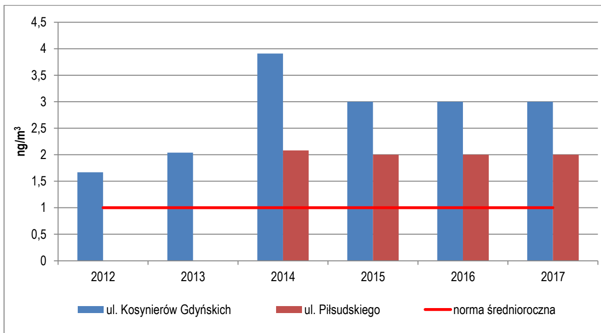
Rysunek 8. Wartości stężeń średniorocznych benzo(a)pirenu zmierzonych na stacjach w Gorzowie Wielkopolskim w latach 2012-2017
