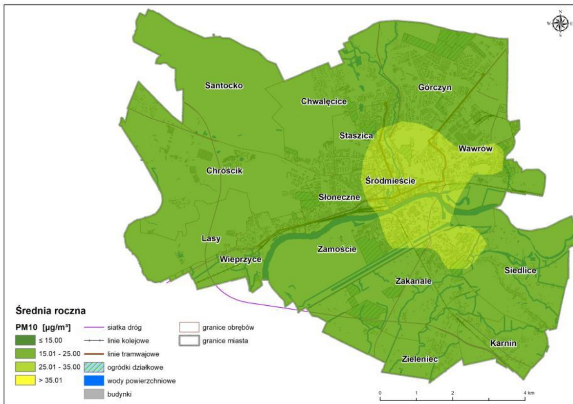
Rysunek 11. Rozkład przestrzenny stężeń średniorocznych pyłu zawieszonego PM10 w Gorzowie Wielkopolskim w 2017 roku 31
