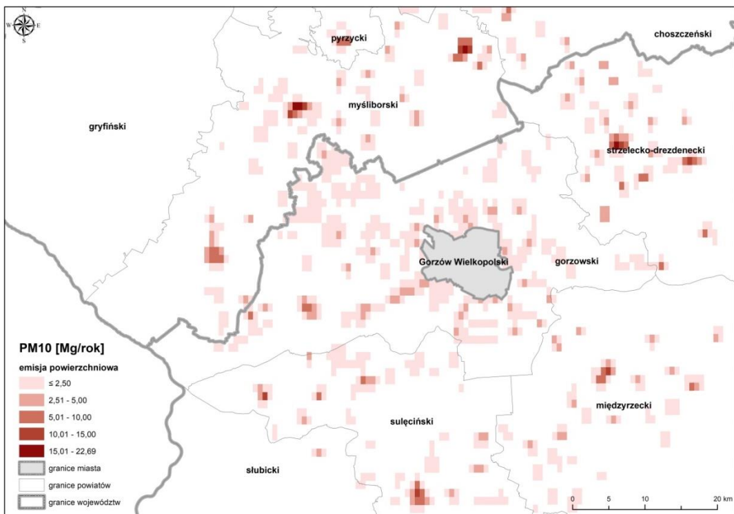
Rysunek 33. Lokalizacja źródeł emisji powierzchniowych pyłu zawieszzonego PM10 z pasa 30 km wokół Gorzowa Wielkopolskiego w roku bazowym 2017 85
