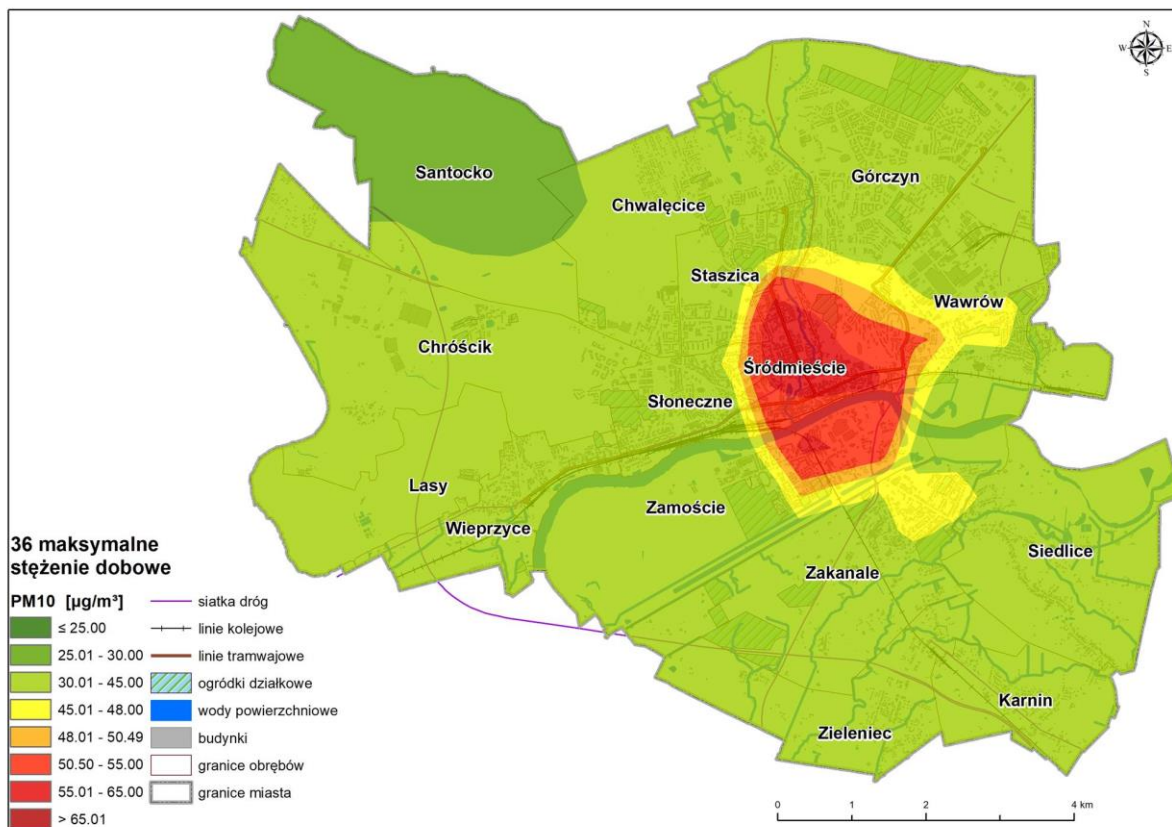
Rysunek 12. Rozkład przestrzenny stężeń średnich 24-godzinnych pyłu zawieszonego PM10 w Gorzowie Wielkopolskim w 2017 roku 33
