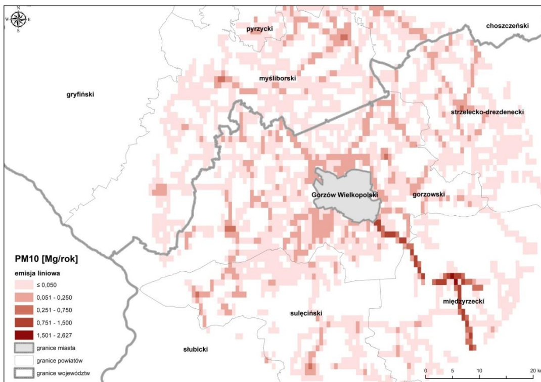
Rysunek 36. Lokalizacja źródeł emisji liniowych pyłu zawieszonego PM10 na drogach powiatowych i gminnych z pasa 30km wokół Gorzowa Wielkopolskiego w roku bazowym 2017 88
