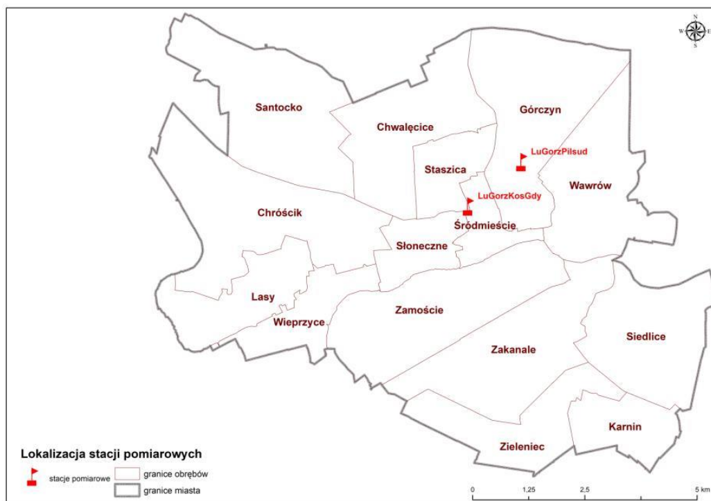
Rysunek 4. Lokalizacja stacji pomiarowych pyłu zawieszzonego PM10 i benzo(a)pirenu w Gorzowie Wielkopolskim 25
