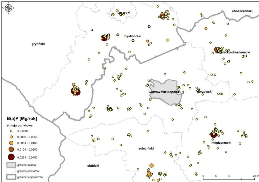
Rysunek 32. Lokalizacja źródeł emisji punktowych B(a)P z pasa 30 km wokół Gorzowa Wielkopolskiego w roku bazowym 2017 84
