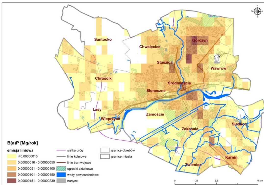
Rysunek 27. Lokalizacja źródeł emisji liniowej B(a)P w Gorzowie Wielkopolskim na drogach powiatowych i gminnych w roku bazowym 2017 74
