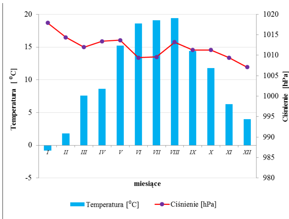
Rysunek 3. Rozkład temperatury średniomiesięcznej oraz ciśnienia w Gorzowie Wielkopolskim w 2017 r. (źródło: Roczna ocena jakości powietrza w województwie lubuskim za rok 2017, WIOŚ)
