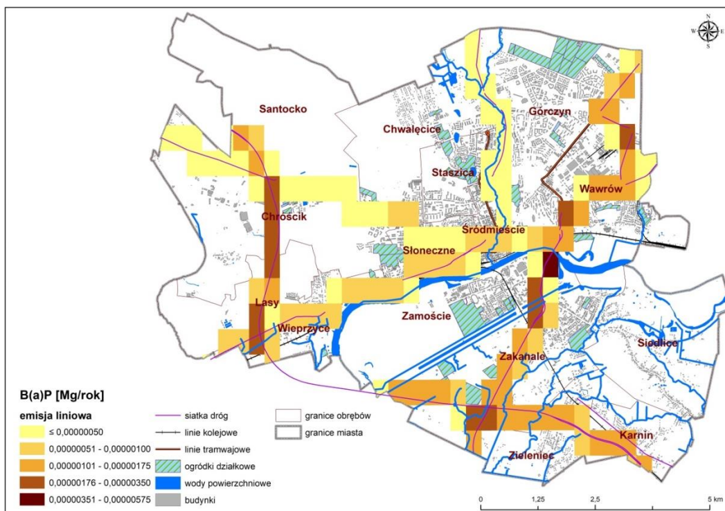
Rysunek 26. Lokalizacja źródeł emisji liniowej B(a)P w Gorzowie Wielkopolskim na drogach krajowych i wojewódzkich w roku bazowym 2017 73
