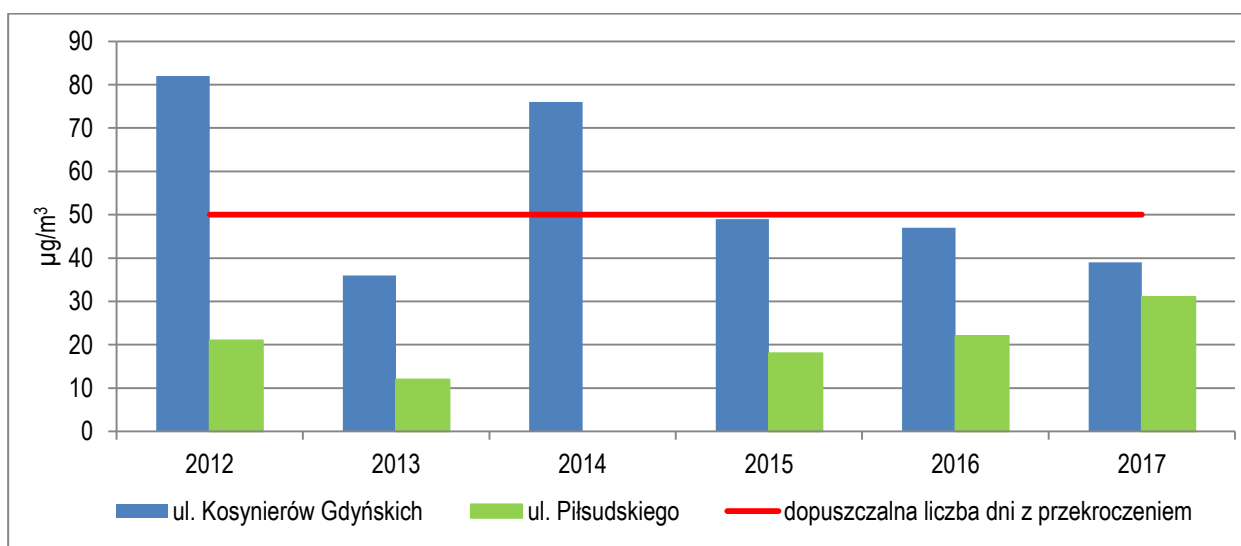
Rysunek 6. Liczba dni z przekroczeniem wartości dopuszczalnej dobowej stężenia pyłu zawieszonego PM10 na stacjach w Gorzowie Wielkopolskim w latach 2012-2017
