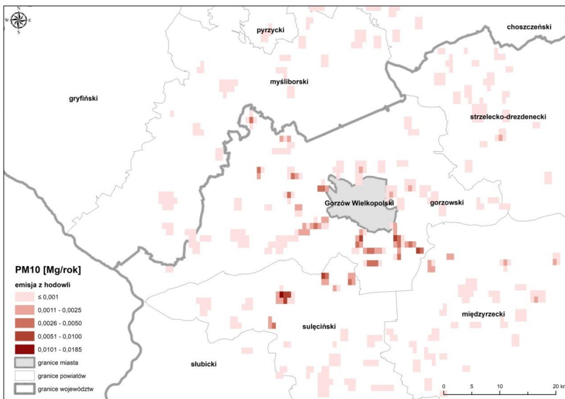
Rysunek 41. Lokalizacja źródeł emisji z hodowli zwierząt pyłu zawieszonego PM10 z pasa 30 km wokół Gorzowa Wielkopolskiego w roku bazowym 2017 93
