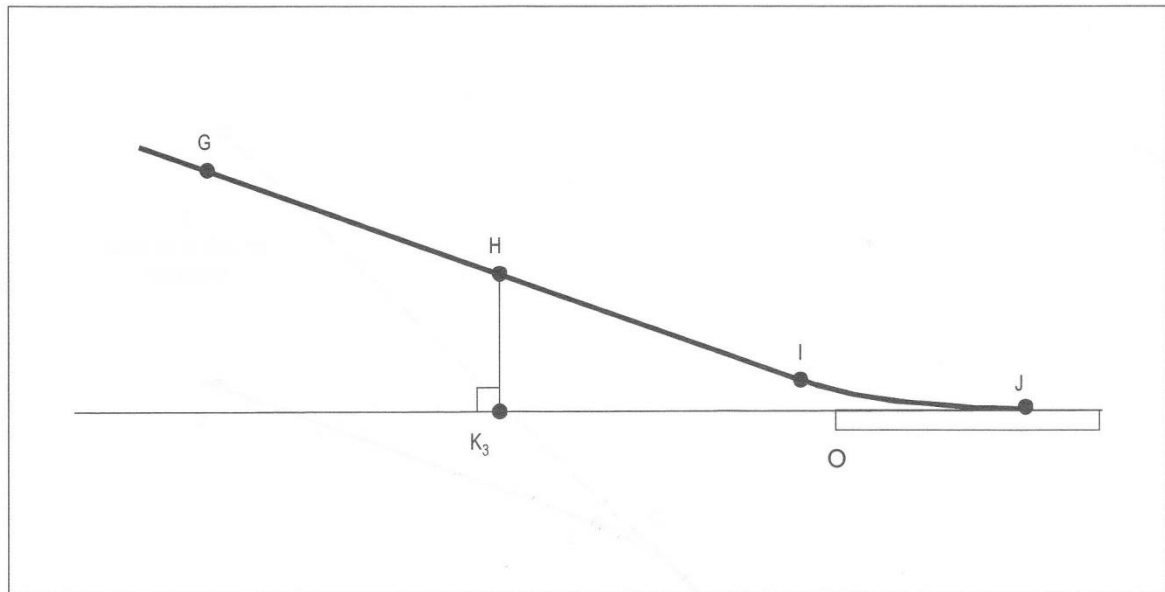
Rys. A2-6. Charakterystyki wzorcowego profilu dla podejścia do lądowania samolotu
