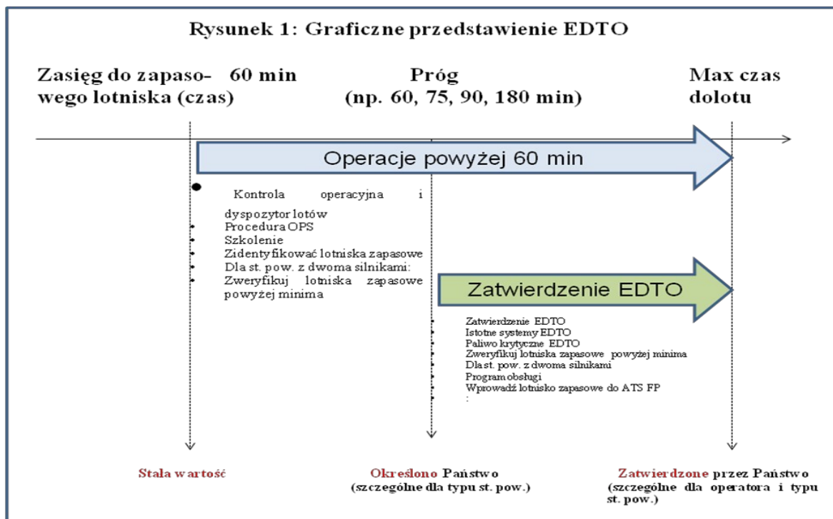
Rysunek B-1 . Ogólna prezentacja graficzna EDTO
