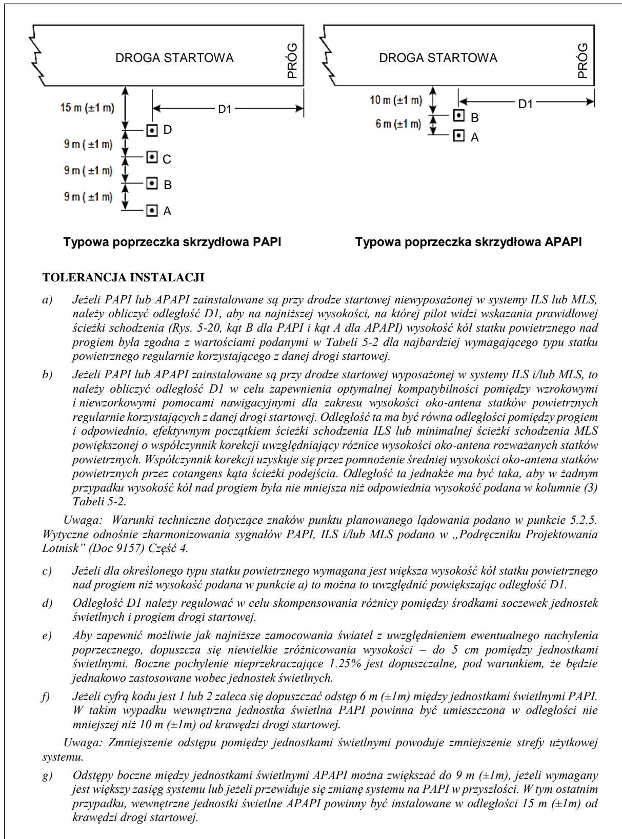
Rysunek 5-19. Ustawienie PAPI i APAPI
