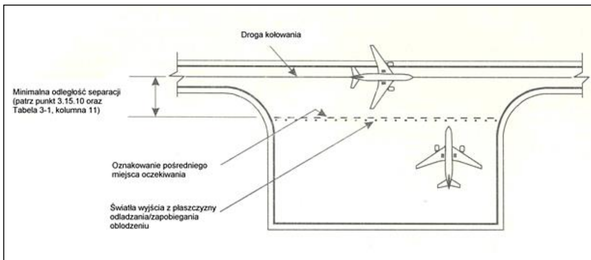
Rysunek 5-28. Przykład oddalonego stanowiska do odladzania / przeciwdziałania oblodzeniu
