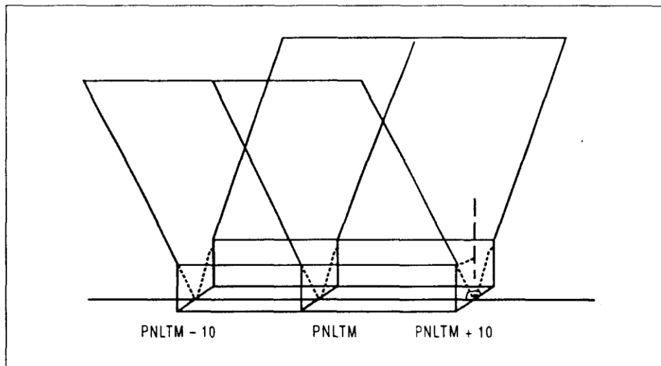
Rys. 8-1. Zakres tolerancji odchylenia bocznego śmigłowca.
