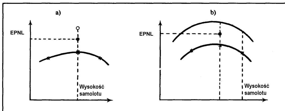
Rys. A2-13. Korekcja uwzględniająca niesymetryczność hałasu bocznego
