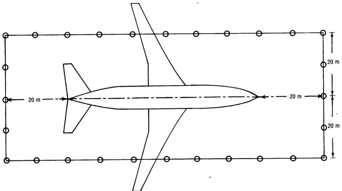
Rys. C-2. Prostokąt punktów pomiarowych hałasu
