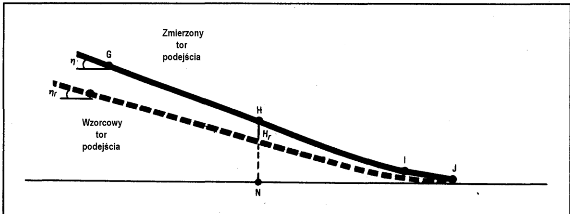
Rys. A1-8. Porównanie zmierzonego i skorygowanego profilu podejścia
