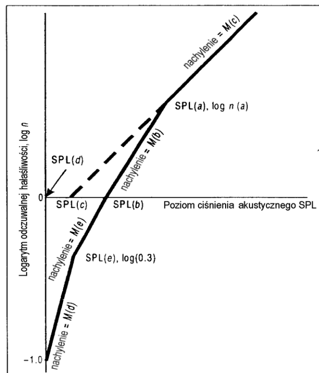
Rys. A2-3. Przykład poziomu odczuwalnego hałasu, skorygowanego tonowo, jako funkcji czasu przelotu samolotu.
