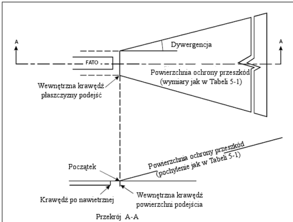
Rysunek 5-12. Powierzchnia ochrony przeszkód dla systemów podejść z widocznością z użyciem wskaźnika ścieżki.
