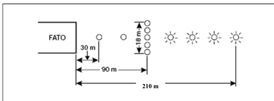
Rysunek 5-10. System światel podejścia
