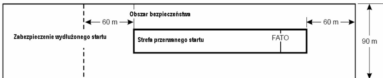
Rysunek 3-1. Obszar bezpieczeństwa dla FATO przyrządowego
