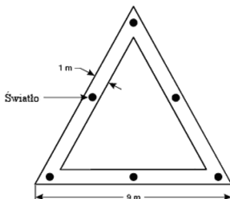
Rysunek 5-4. Oznakowanie punktu celowania
