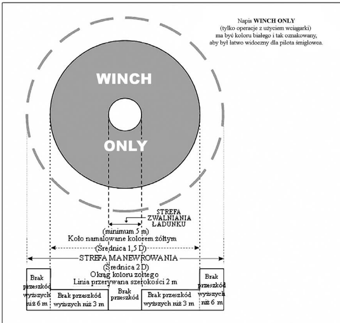
Rysunek 4-11. Obszar najednostce plywajacej dla operacji z uzyciem wciagarki
