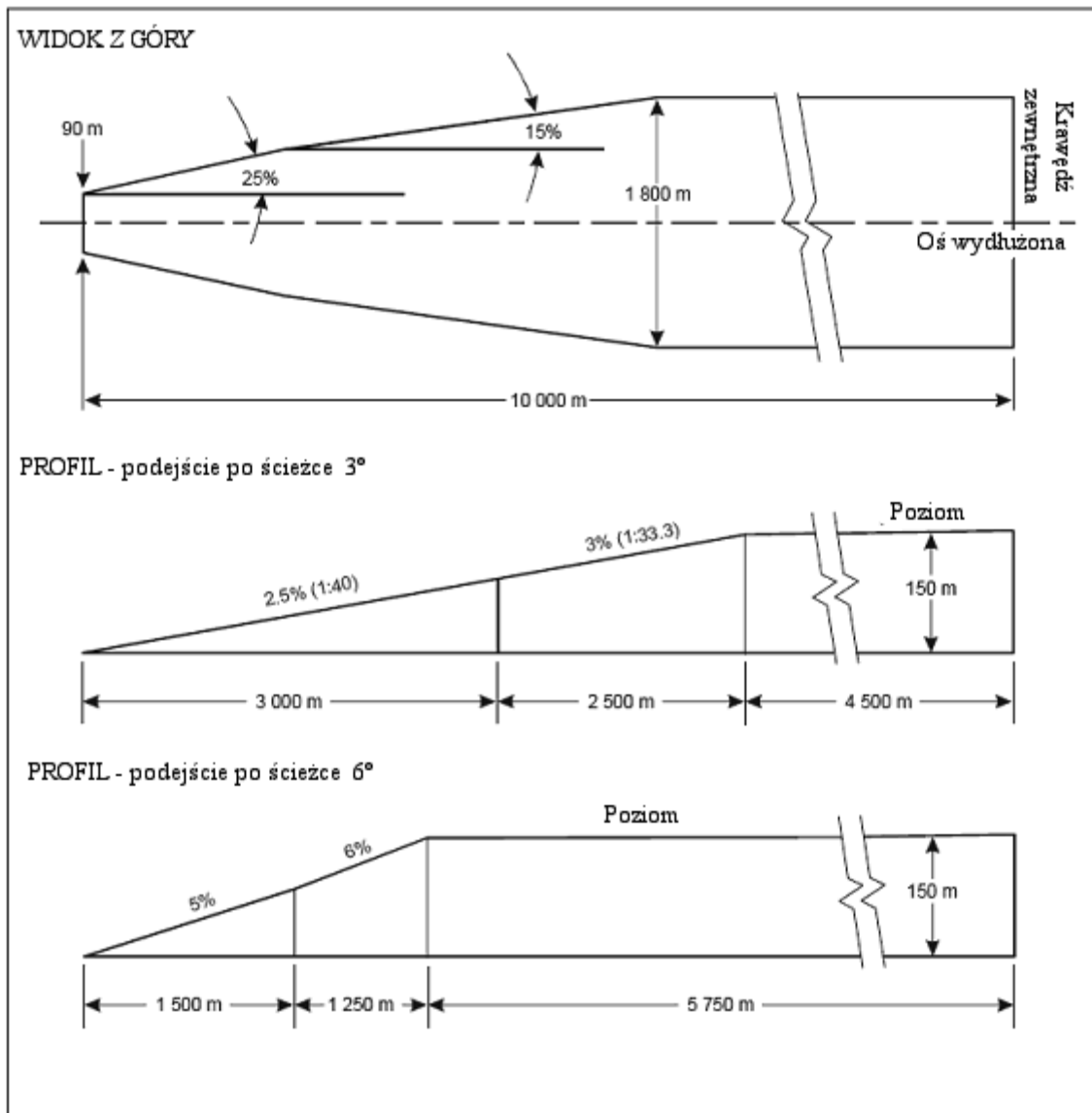
Rysunek 4-6. Powierzchnia podejścia dla obszaru FATO podejść precyzyjnych
