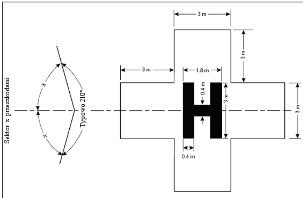
Rysunek 5-1. Oznakowanie tożsamości lotniska dla śmigłowców (pokazane wraz z krzyżem szpitalnym i wskazaniem sektora wolnego od przeszkód)
