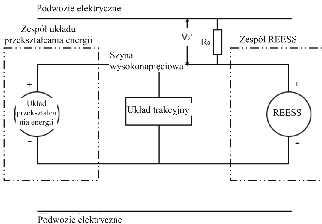
Rysunek 4 Pomiar V_2'
