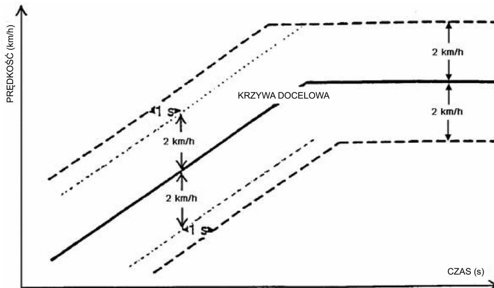
Rysunek 4 Tolerancja prędkości
