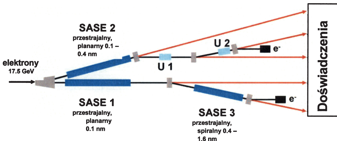
Rysunek 4.2: Schemat rozgałęziania linii promienia elektronów (czarna) i fotonów (czerwony) przez różne undulatory samowzmacniającej emisji spontanicznej (SASE) oraz emisji spontanicznej. Linie wiązek elektronowych kończą bieg w dwóch wiązkołapach, zaś linie promieni fotonowych w Hali Doświadczalnej.
