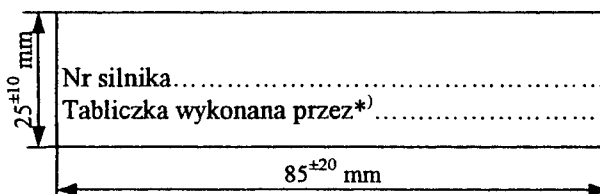
Rys. 2. PRZYKŁADOWY SPOSÓB UMIESZCZANIA CECHY IDENTYFIKACYJNEJ NA NALEPCE LUB TABLICZCE NUMERU SILNIKA
