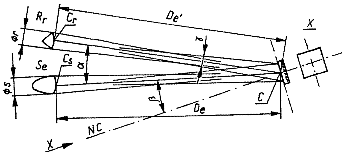
Rysunek 74. Schemat pomiaru współczynnika odbicia
