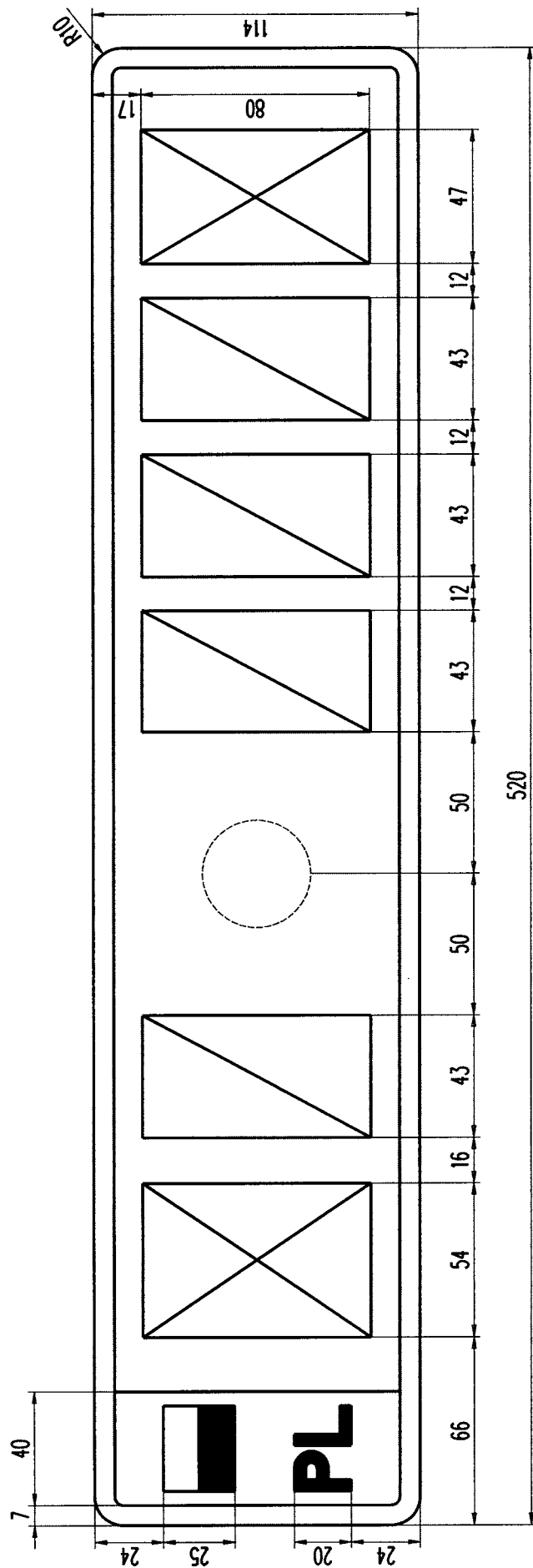
Rysunek 57. Tablica samochodowa tymczasowa jednorzędowa (1 litera, 1 cyfra, 3 cyfry, 1 litera)
