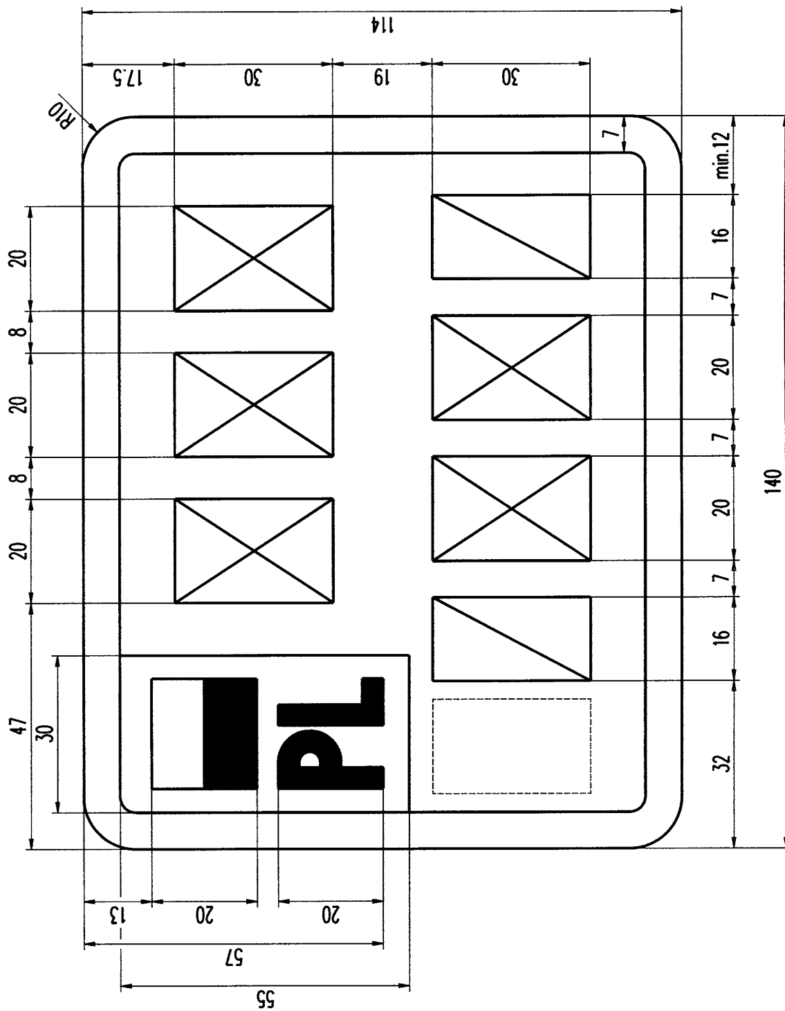
Rysunek 49. Tablica motorowerowa zwyczajna (3 litery, 1 cyfra, 2 litery, 2 litery, 1 cyfra)
