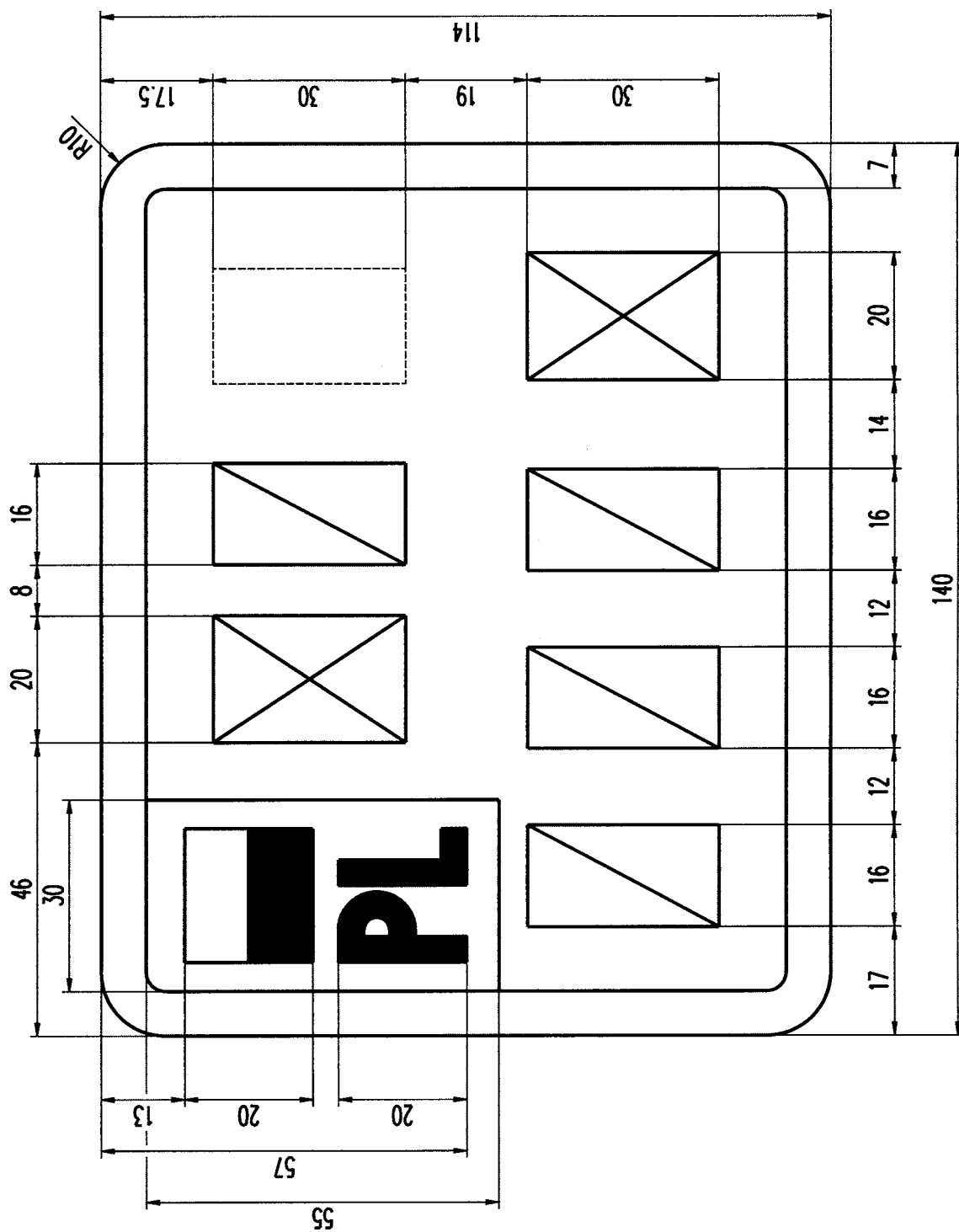
Rysunek 67. Tablica motorowerowa tymczasowa badawcza
