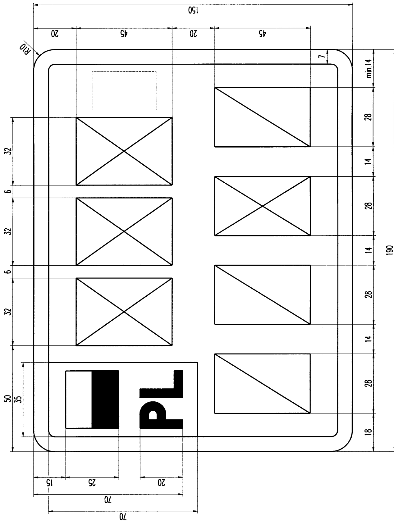
Rysunek 37. Tablica motocyklowa zwyczajna (3 litery, 2 cyfry, 1 litera, 1 cyfra)
