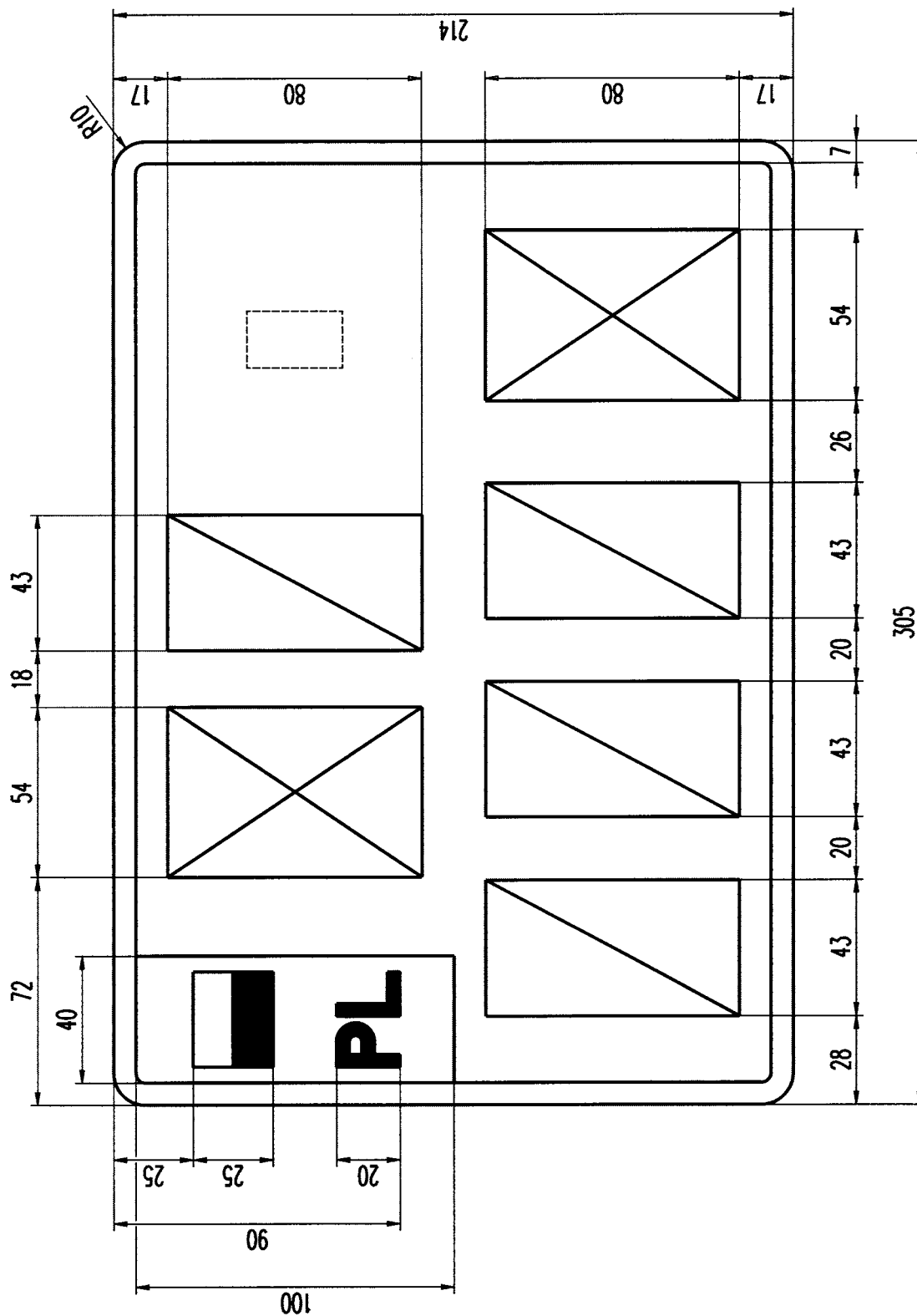
Rysunek 61. Tablica samochodowa tymczasowa dwurzędowa badawcza
