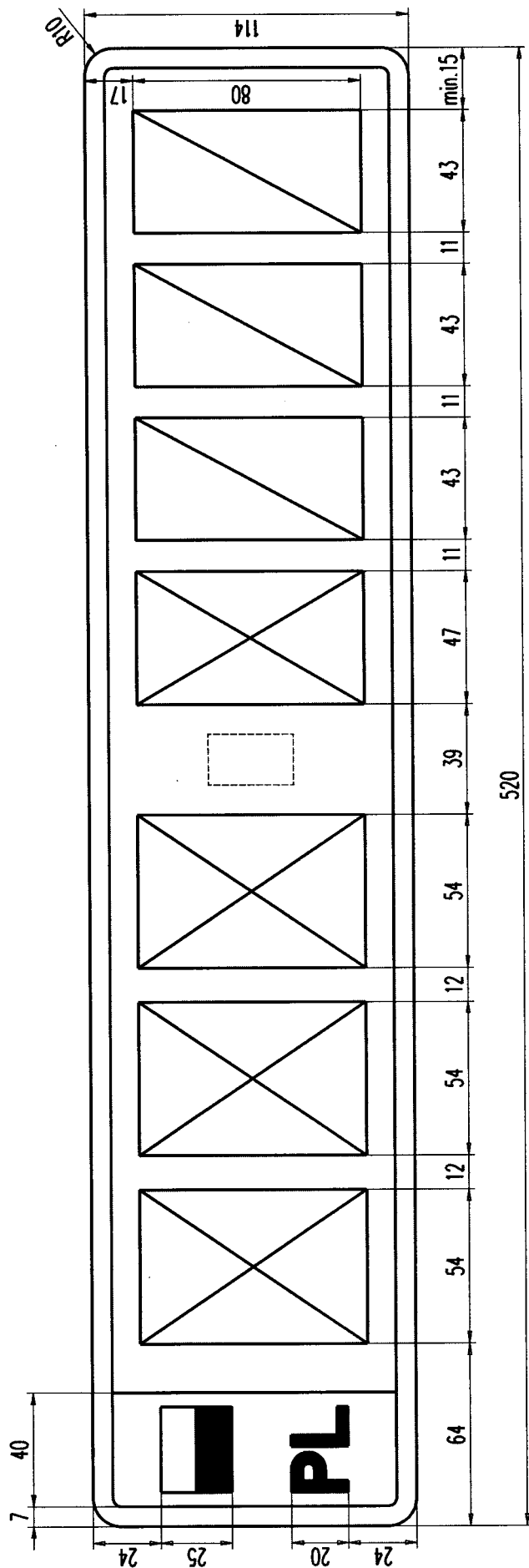
Rysunek 14. Tablica samochodowa zwyczajna jednorzędowa (3 litery, 1 litera, 1 litera, 3 cyfry)
