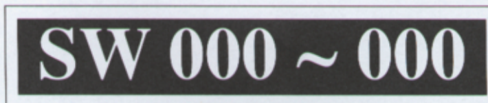
Rys. 2. Identyfikator numeryczny
