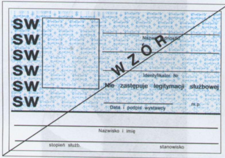
Rys. 1. Identyfikator foliowany
